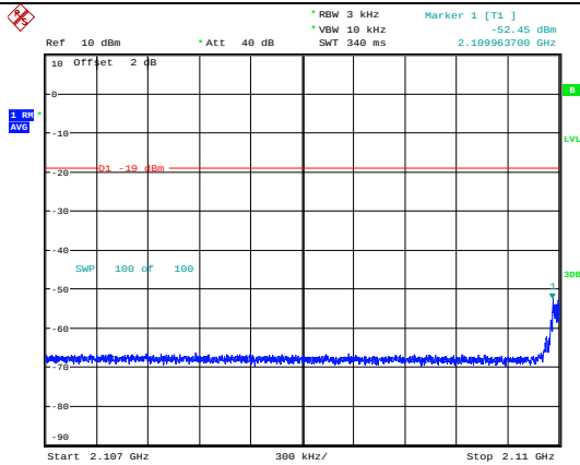
Left Side-GSM-Pre AGC
