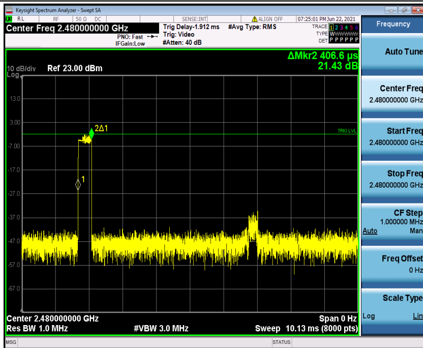
3DH1_Ant1_Hop_2480
