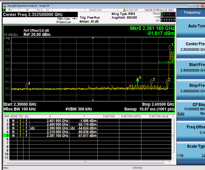
DH5_Ant1_Low_Hop_2402
