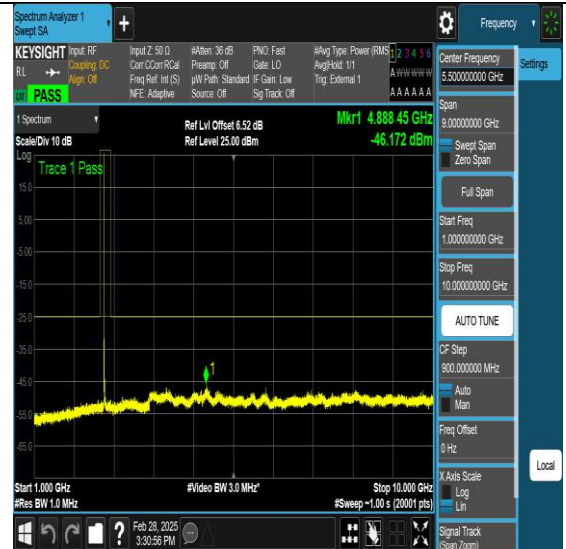
NTNV-N41-PC3-30-30-M-DFT-QPSK-Edge_1RB_Left-Ant1-PASS
