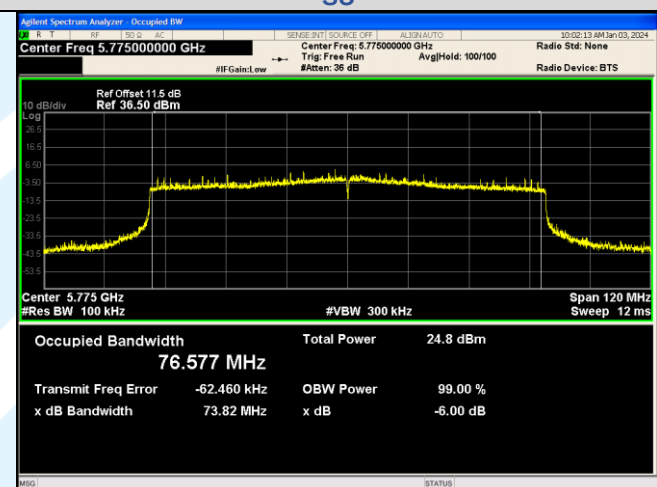
IEEE 802.11ax_Channel 155_80MHz_Antenna 1_RU&Index SU
