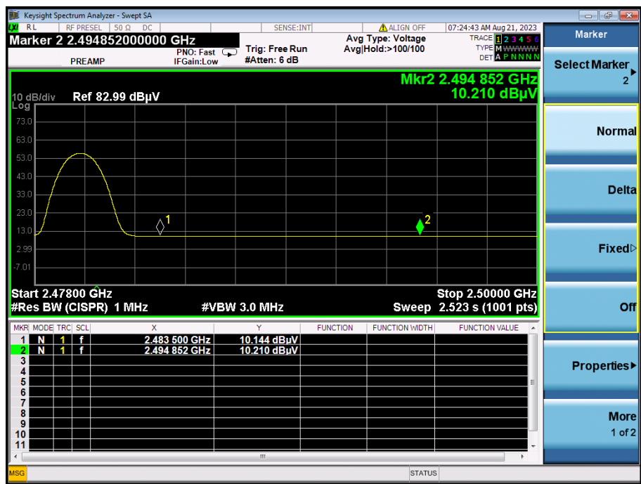
(AVERAGE, Channel 78, \pi/4 -DQPSK)
