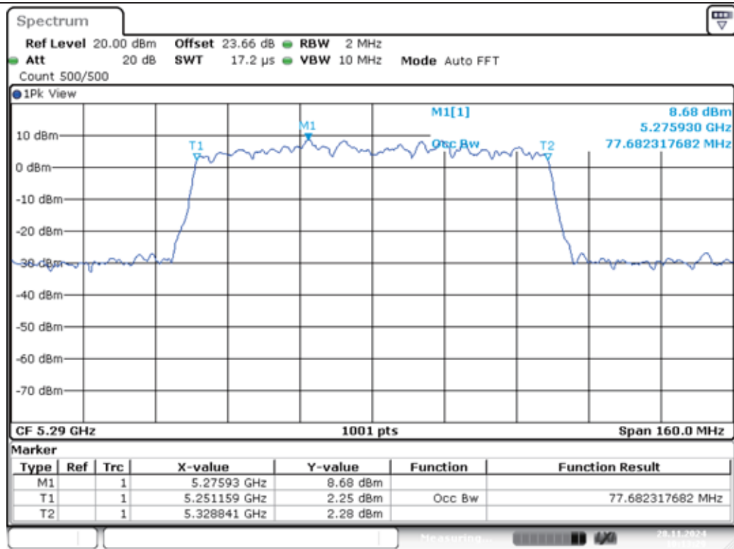
11AX80MIMO-Ant1-5290
