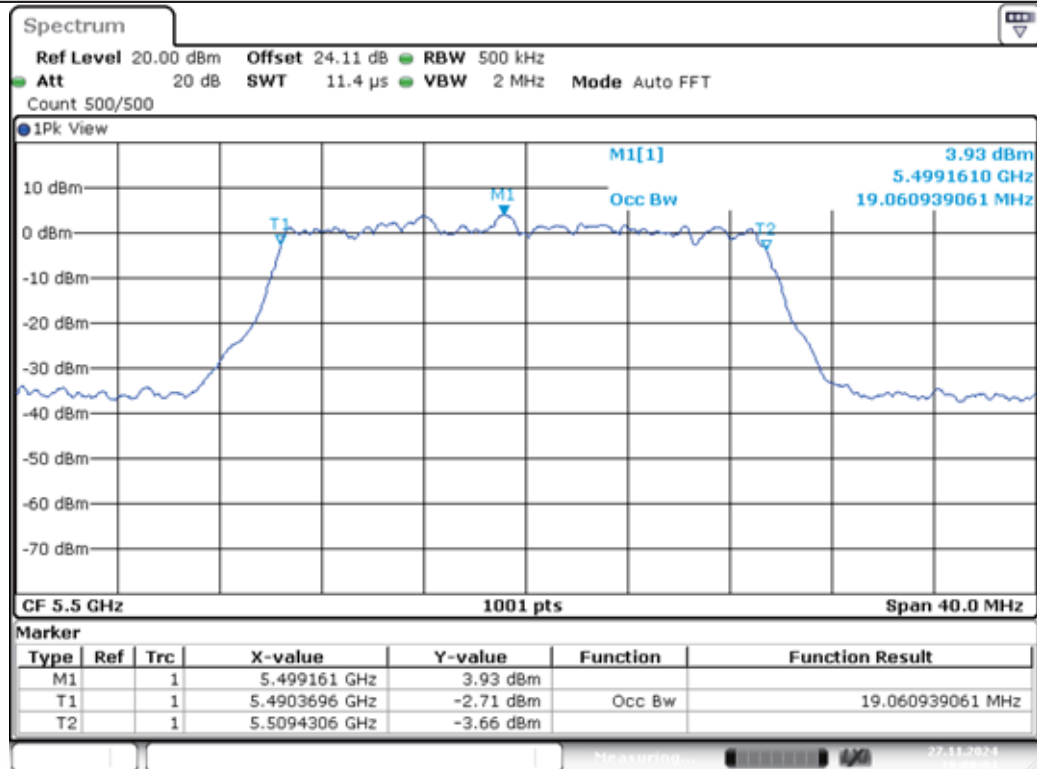
11AX20MIMO-Ant1-5500
