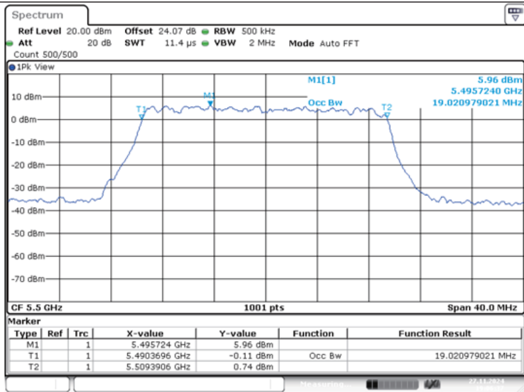
11AX20MIMO-Ant1-5500
