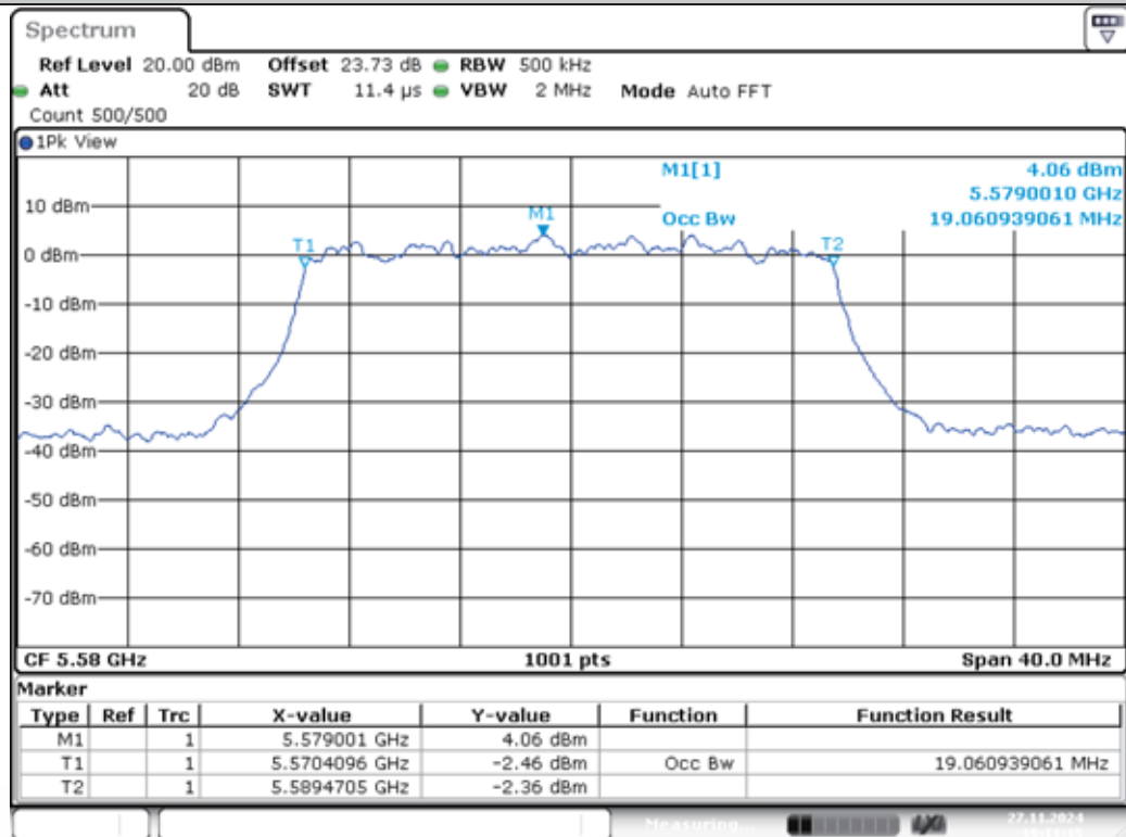
11AX20MIMO-Ant1-5580
