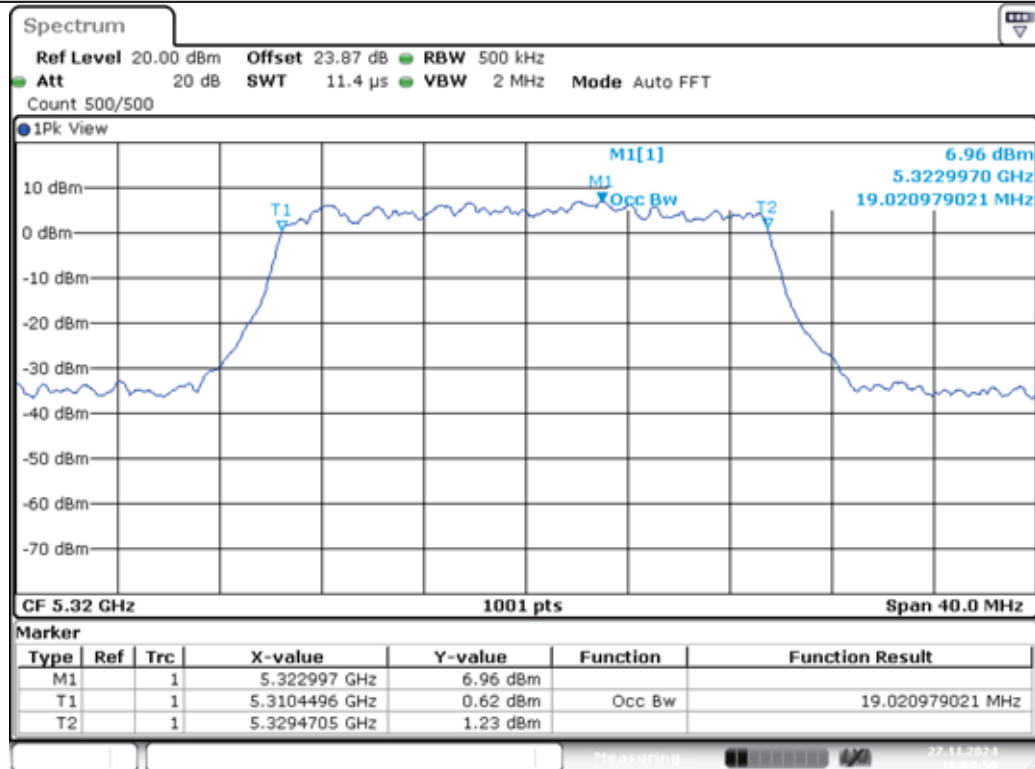
11AX20MIMO-Ant1-5320
