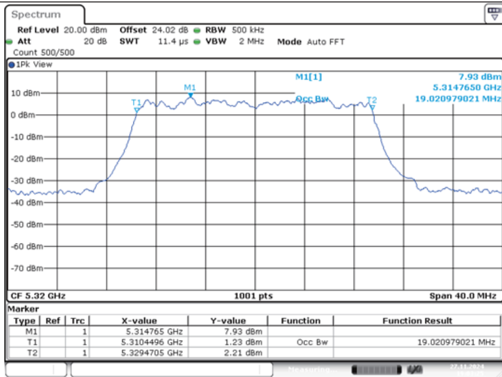
11AX20MIMO-Ant1-5320
