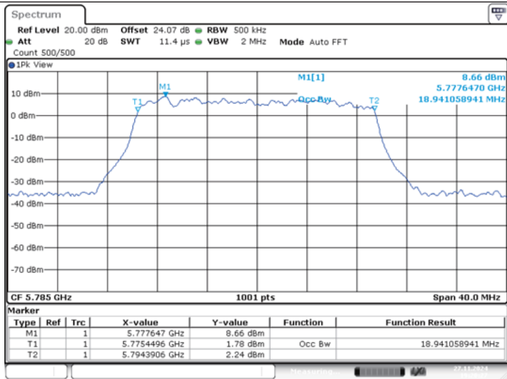
11AX20MIMO-Ant1-5785
