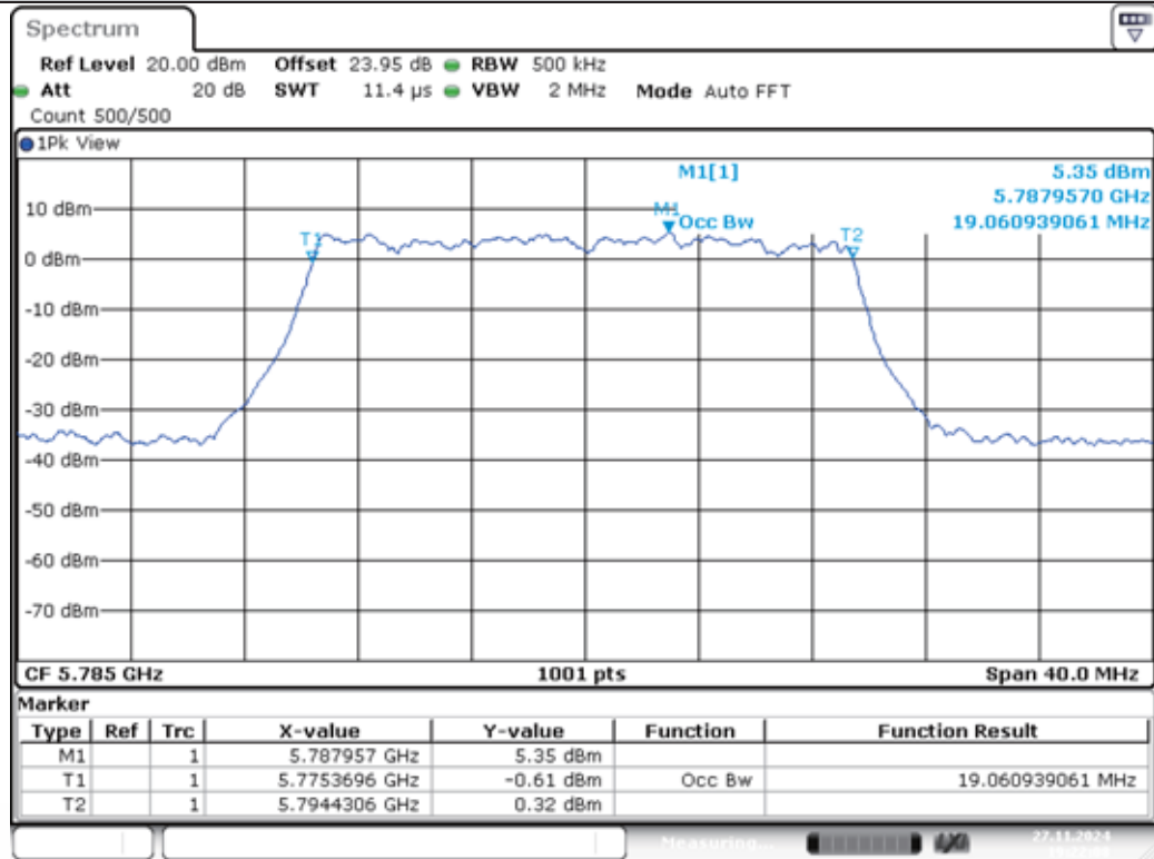
11AX20MIMO-Ant1-5785
