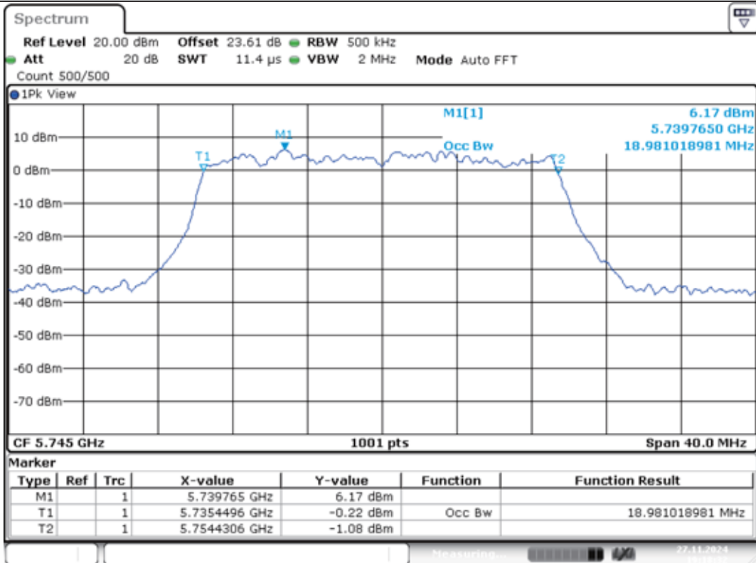
11AX20MIMO-Ant1-5745
