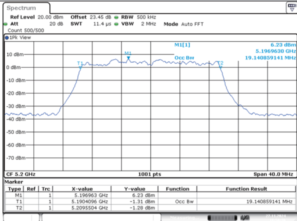
11AX20MIMO-Ant1-5200
