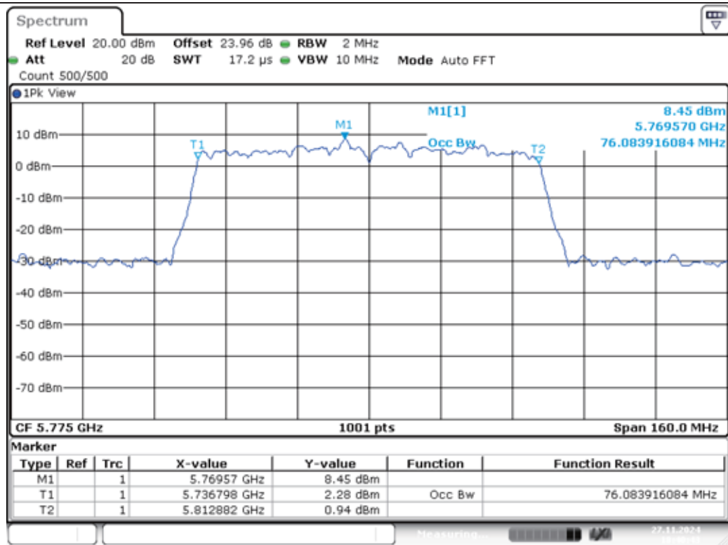
11AC80MIMO-Ant1-5775
