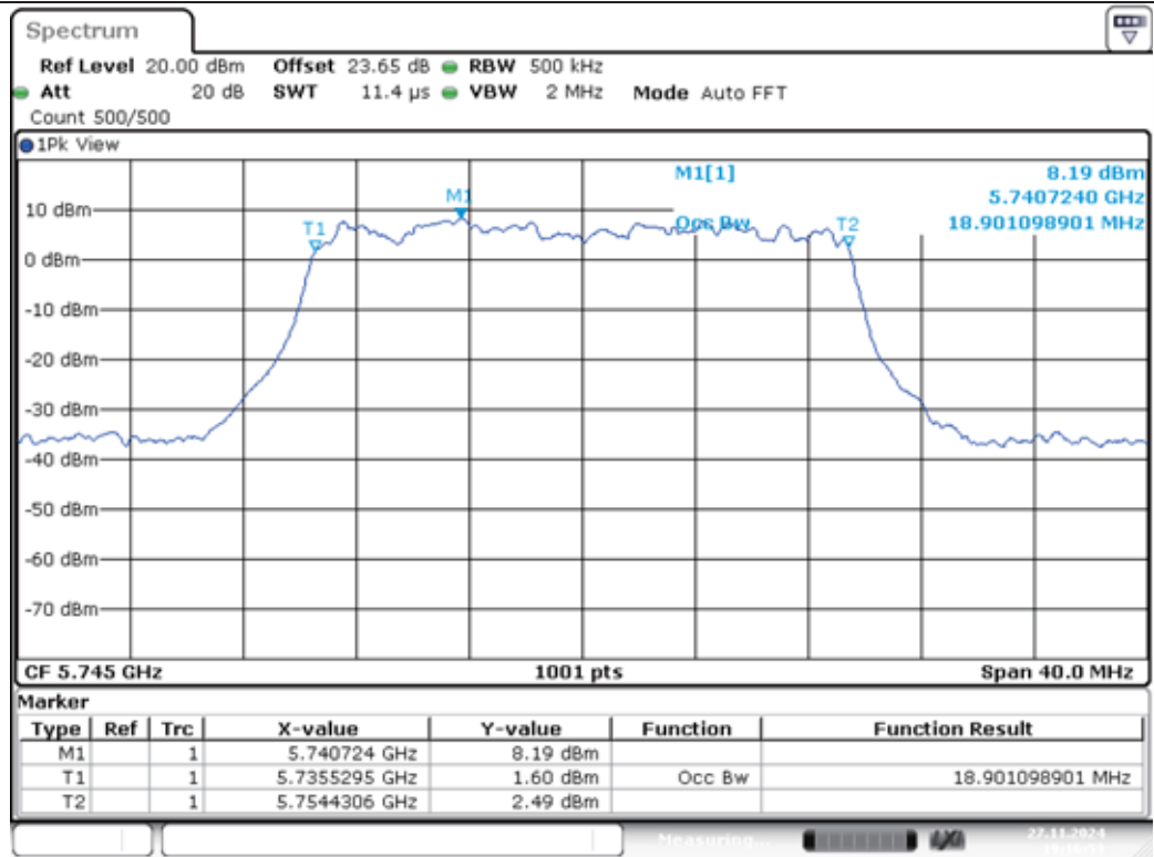
11AX20MIMO-Ant1-5745
