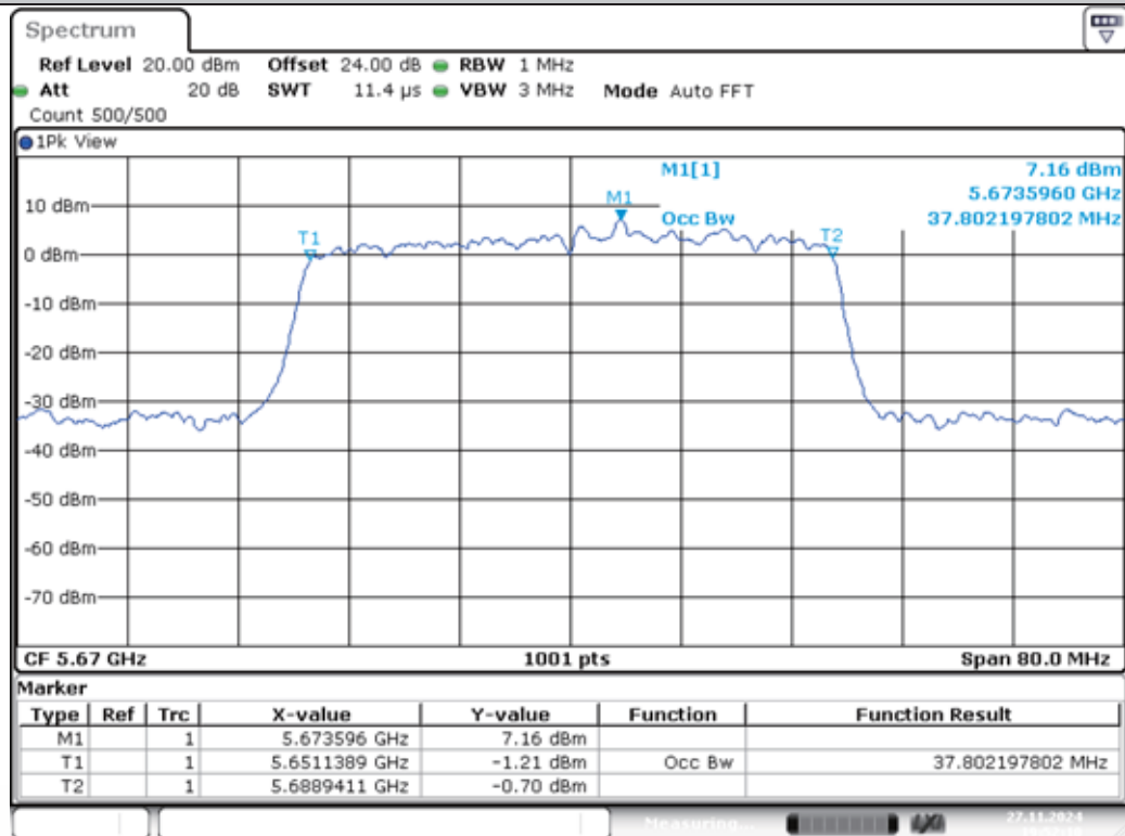
11AX40MIMO-Ant1-5670
