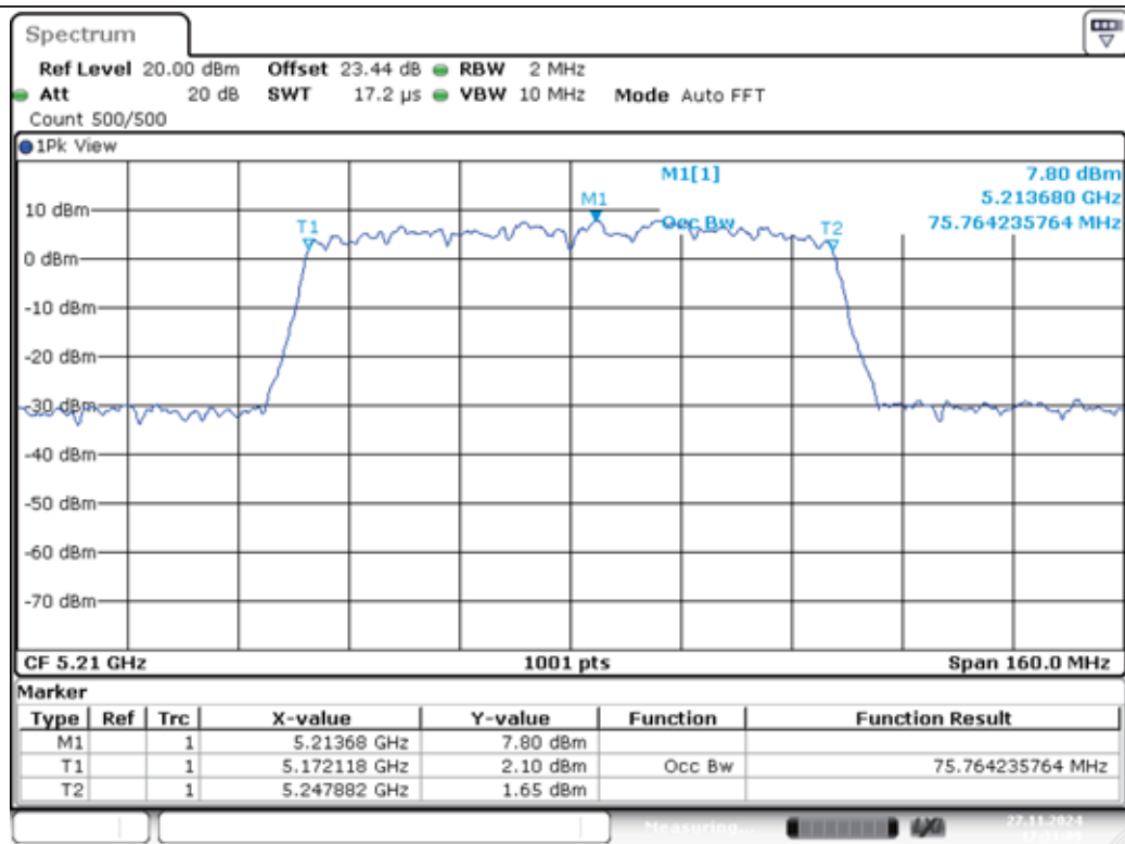
11AC80MIMO-Ant1-5210
