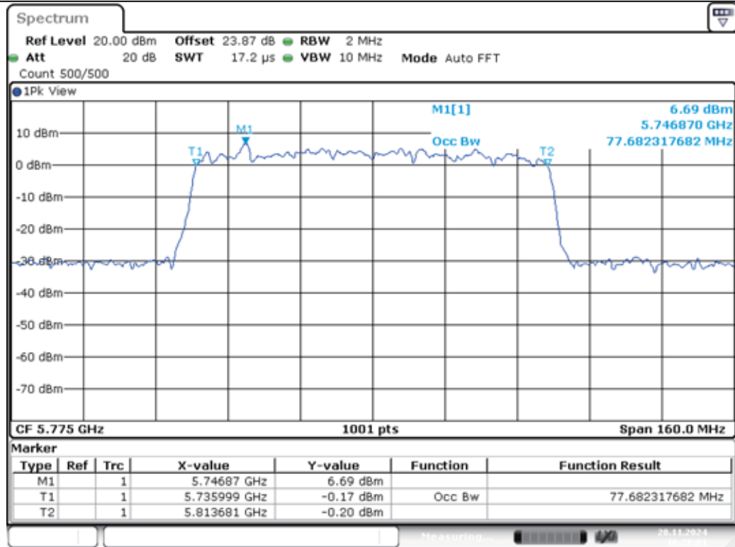
11AX80MIMO-Ant1-5775
