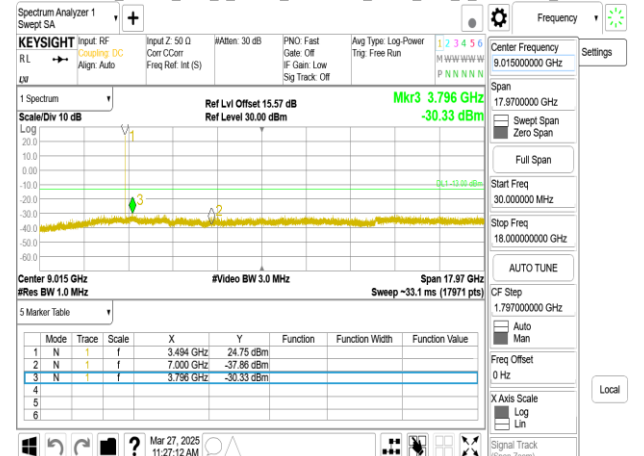
Band77-Part27_15MHz_DFT_s_OFDM_SCS30kHz_BPSK_RB1_1_CH633334_below 18G
