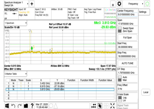
Band77-Part27_15MHz_DFT_s_OFDM_SCS30kHz_BPSK_RB1_1_CH630500upper 18G
