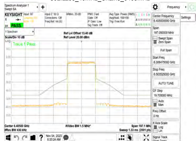
802.11be_40MHz_Chain3_6405MHz
