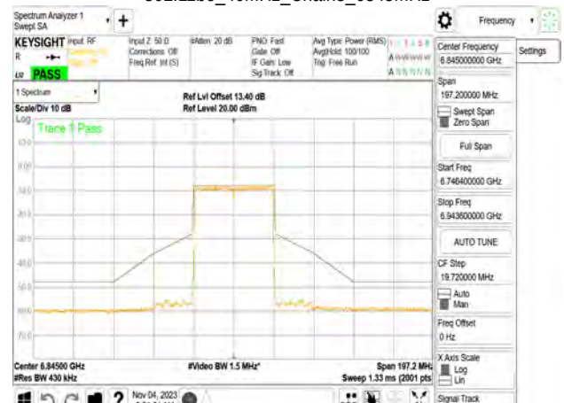
802.11be_40MHz_Chain3_6845MHz
