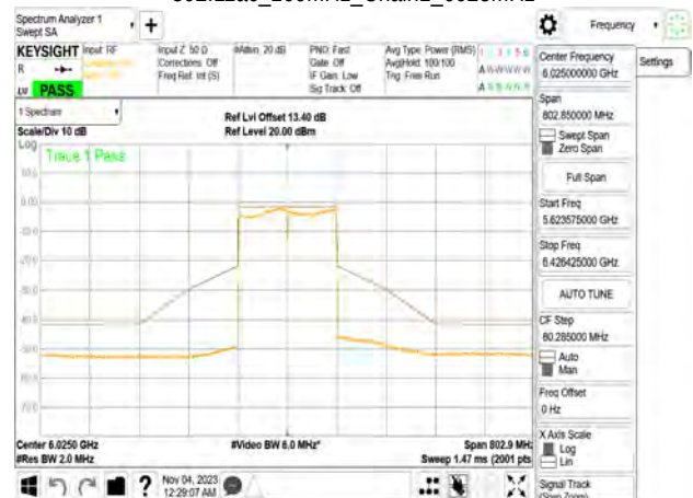
802.11ac_160MHz_Chain1_6025MHz
