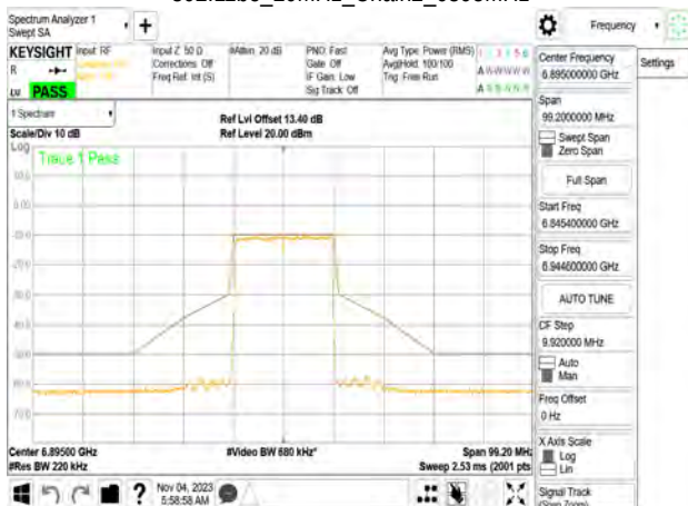
802.11be_20MHz_Chain2_6895MHz
