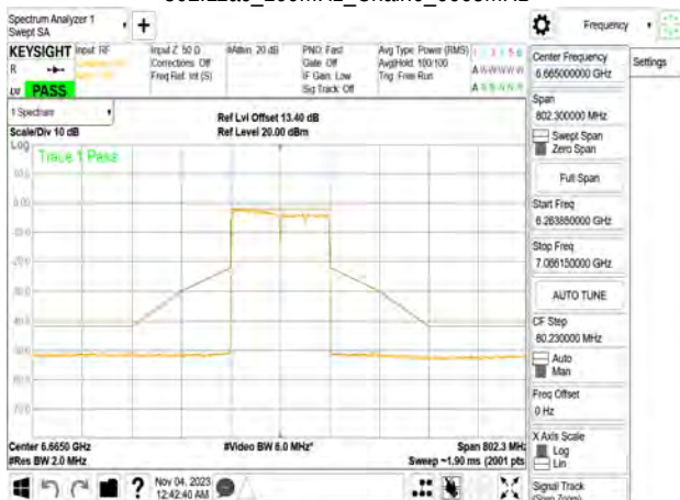
802.11ac_160MHz_Chain0_6665MHz
