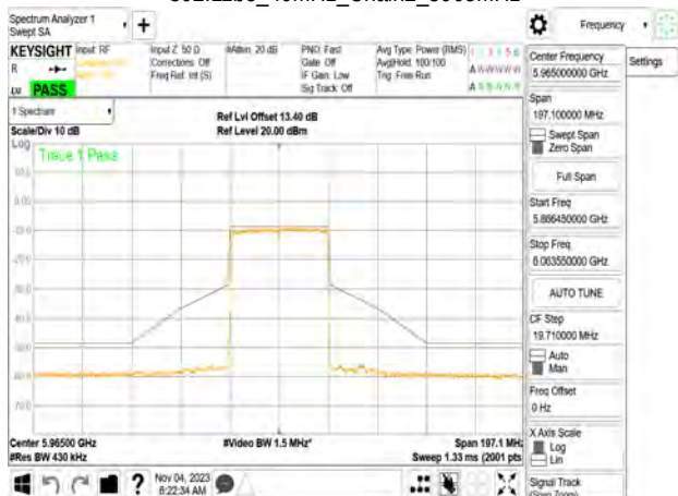
802.11be_40MHz_Chain2_5965MHz
