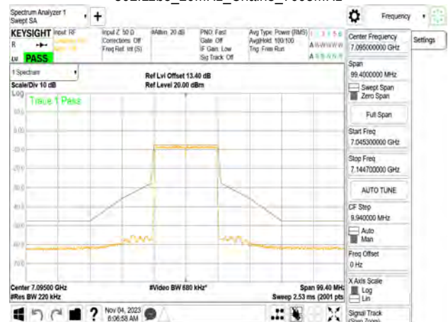
802.11be_20MHz_Chain3_7095MHz
