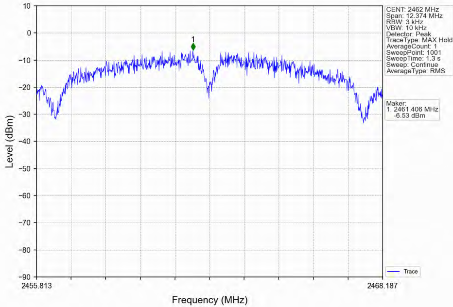
802.11b_HCH_2462MHz_Ant2 (MIMO) NTN
