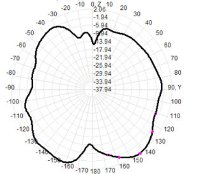
2500.0MHz Total(E2-YZ), Max= 1.81dBi
