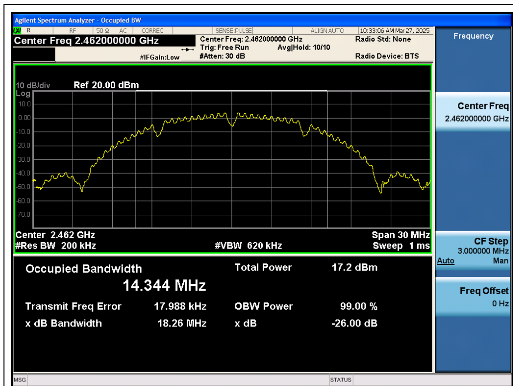
Test_Graph_802.11b_ANT2_2462_1Mbps_OBW
