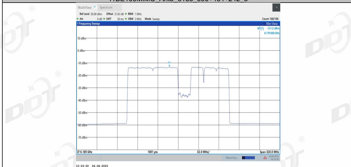
11BE160MIMO Ant3 6185 996+484+242 6
