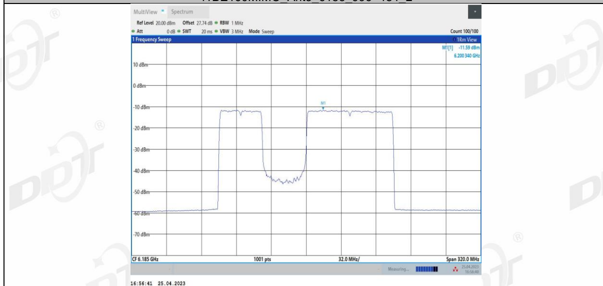
11BE160MIMO Ant3 6185 996+484 3
