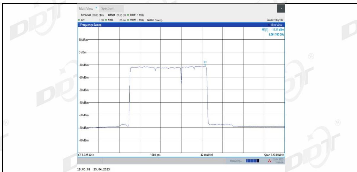
11BE160MIMO Ant4 6025_996+484+242_5
