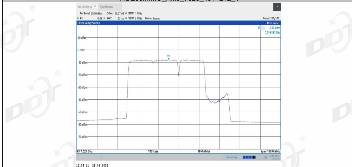
11BE80MIMO Ant4 7025 484+242 1
