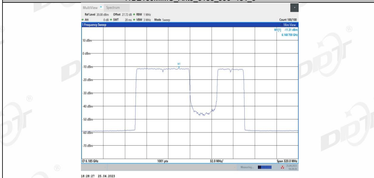
11BE160MIMO Ant3 6185 996+484 4
