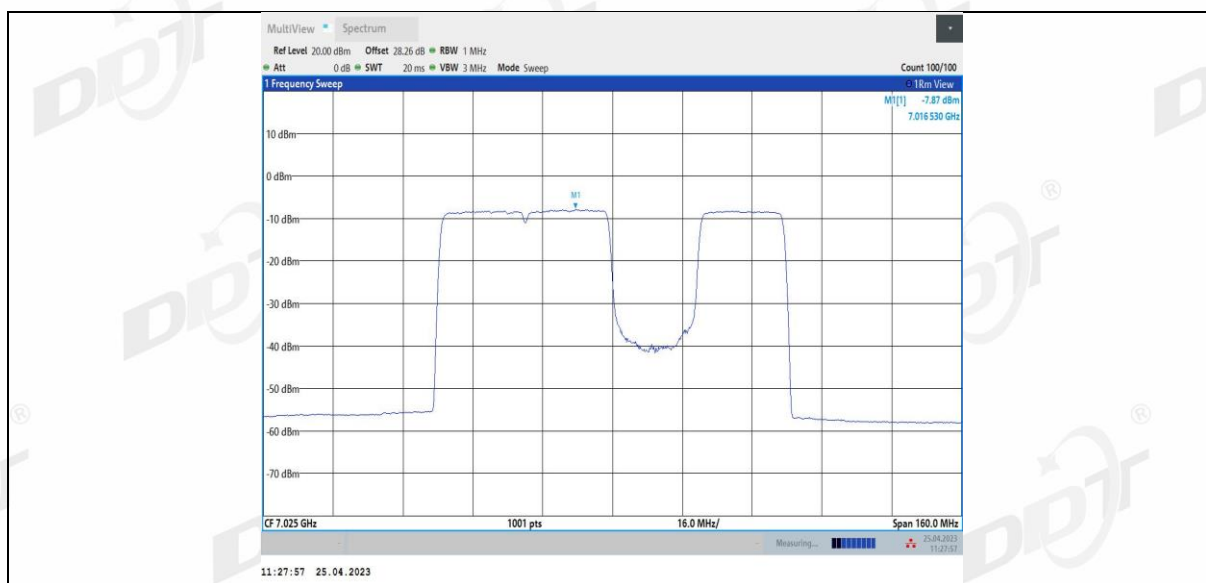
11BE80MIMO Ant3 7025 484+242 4
