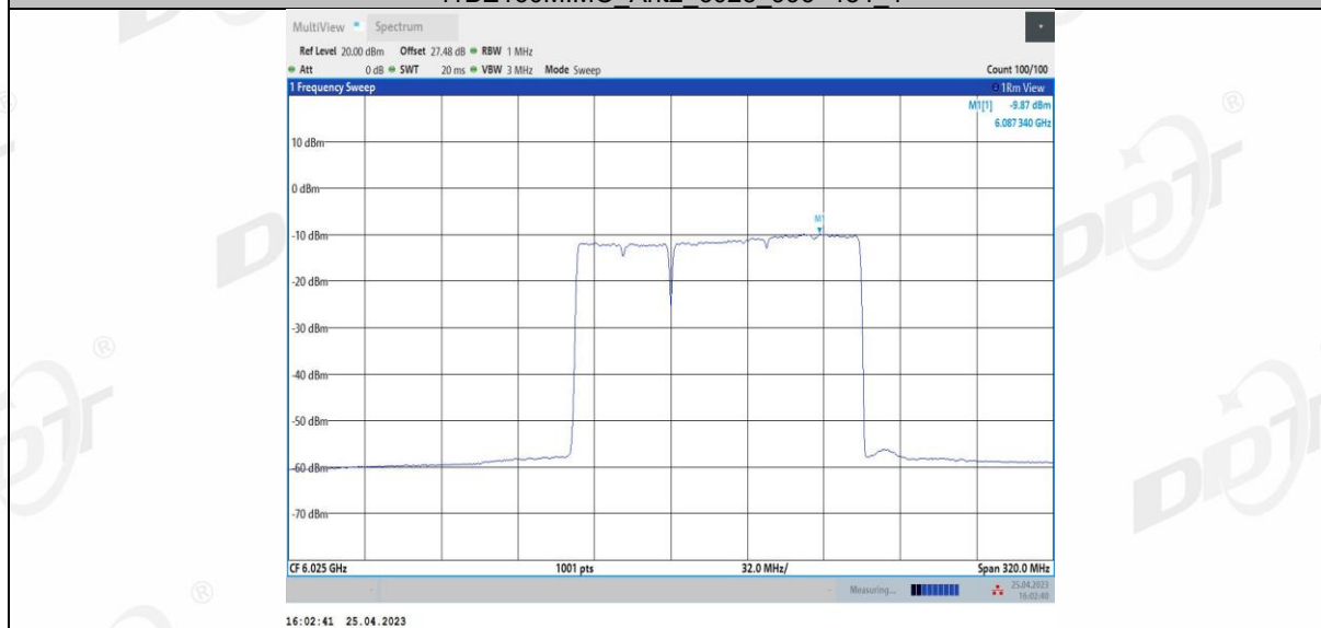
11BE160MIMO Ant2 6025 996+484 2
