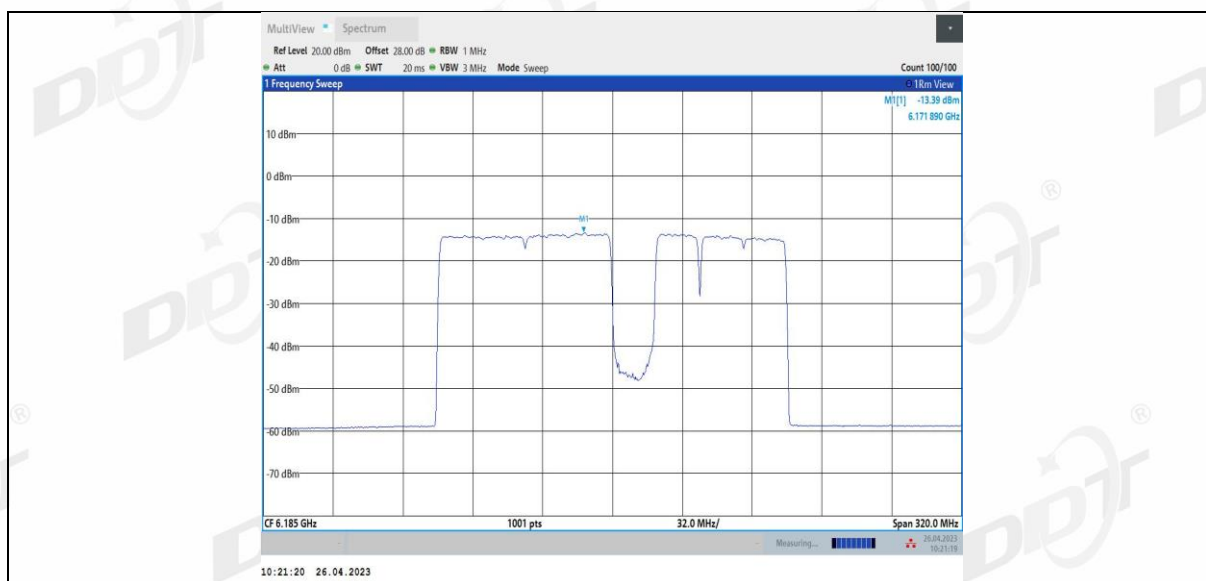
11BE160MIMO Ant1 6185 996+484+242 6
