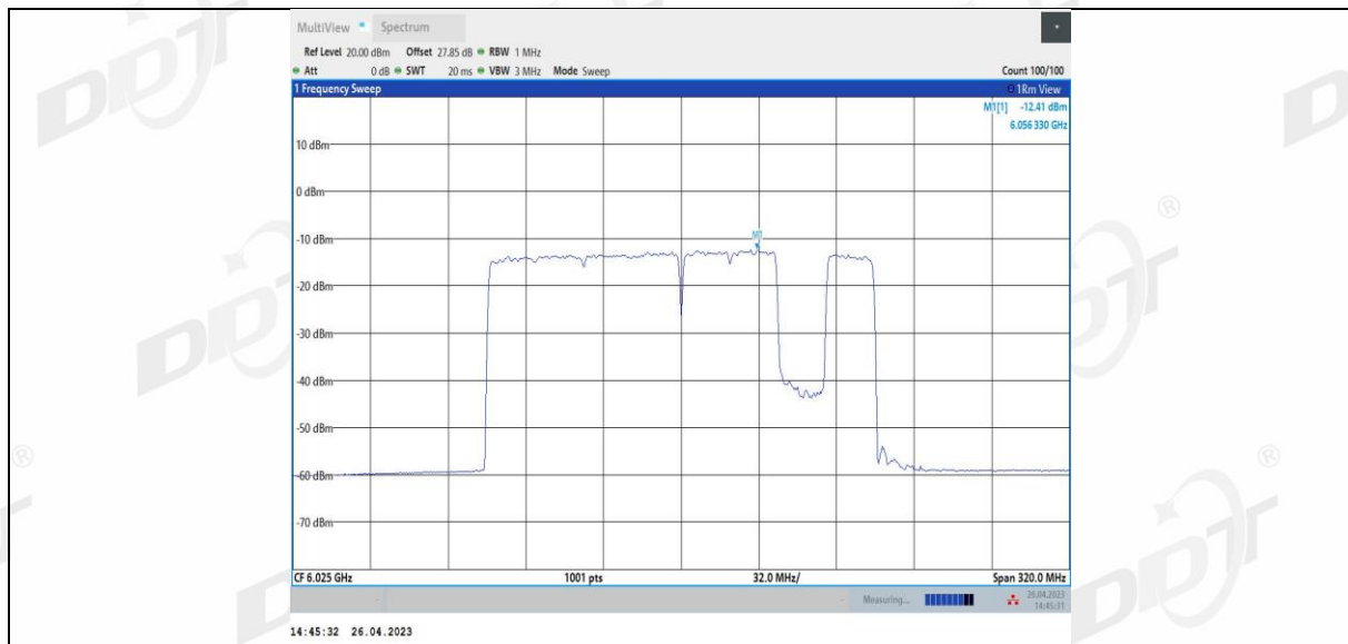
11BE160MIMO Ant4 6025 996+484+242 8
