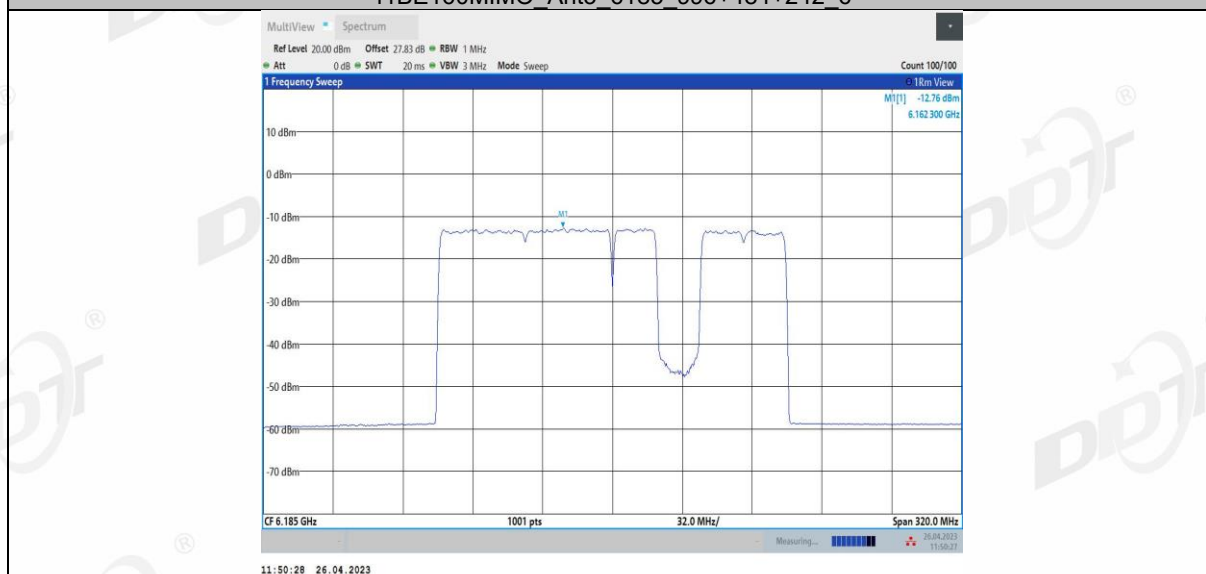
11BE160MIMO Ant3 6185 996+484+242 7
