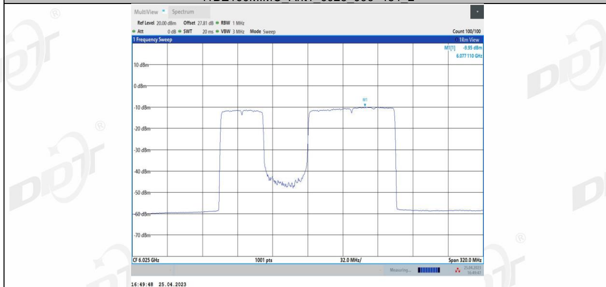
11BE160MIMO Ant1_6025_996+484_3
