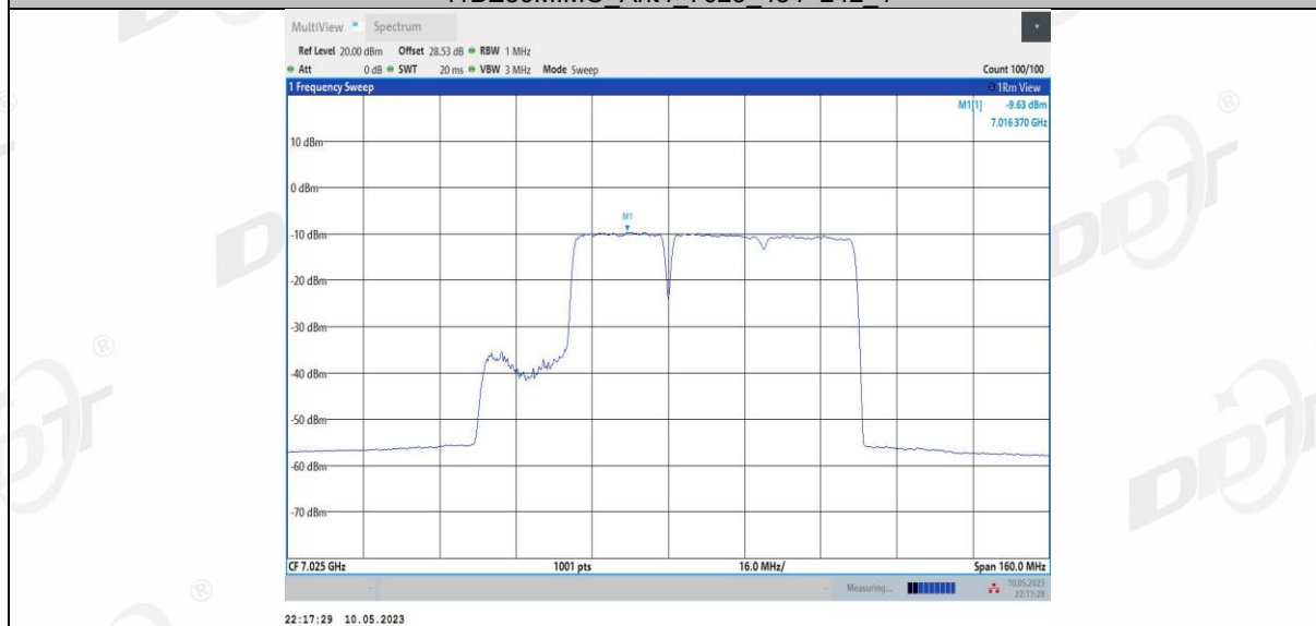
11BE80MIMO Ant4 7025 484+242 2
