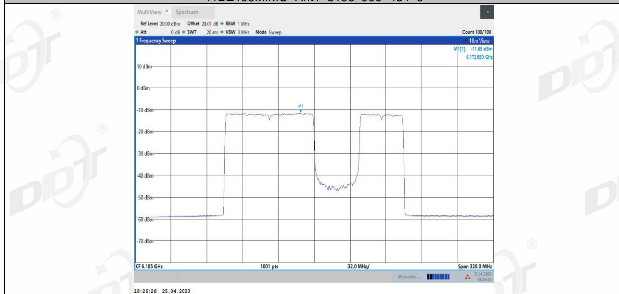
11BE160MIMO Ant1_6185_996+484_4
