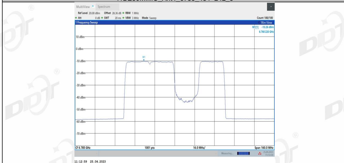
11BE80MIMO Ant4 6785 484+242_4
