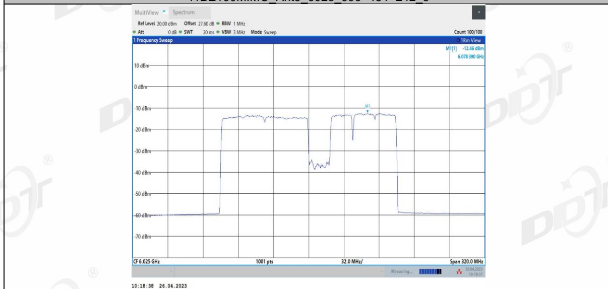
11BE160MIMO Ant3 6025 996+484+242_6
