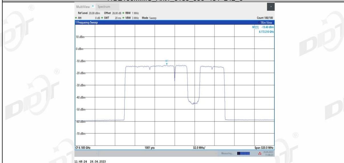
11BE160MIMO Ant1 6185 996+484+242 7
