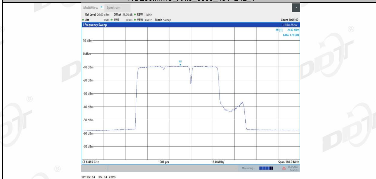
11BE80MIMO Ant4 6865 484+242_1
