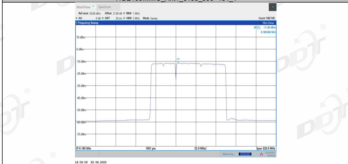
11BE160MIMO Ant1_6185 996+484 2
