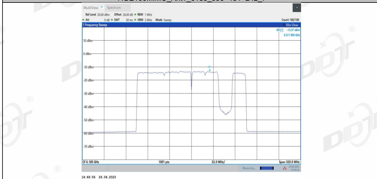
11BE160MIMO Ant1 6185 996+484+242 8
