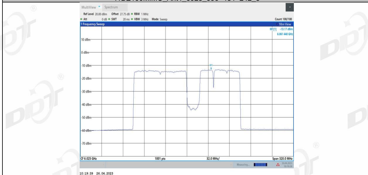
11BE160MIMO Ant4 6025_996+484+242_6
