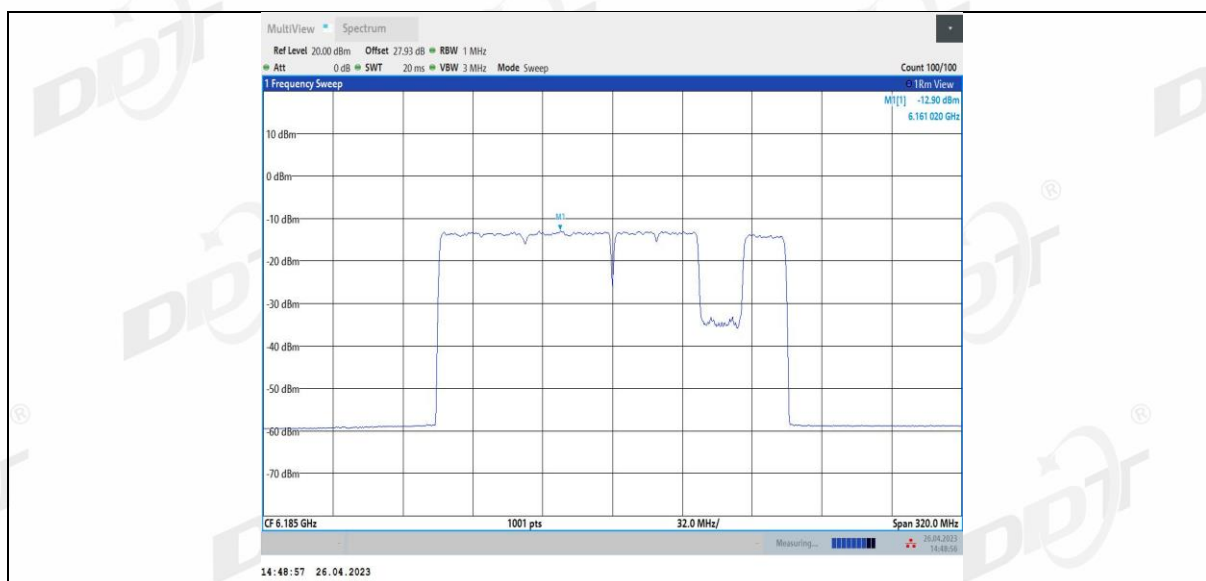
11BE160MIMO Ant3 6185 996+484+242 8
