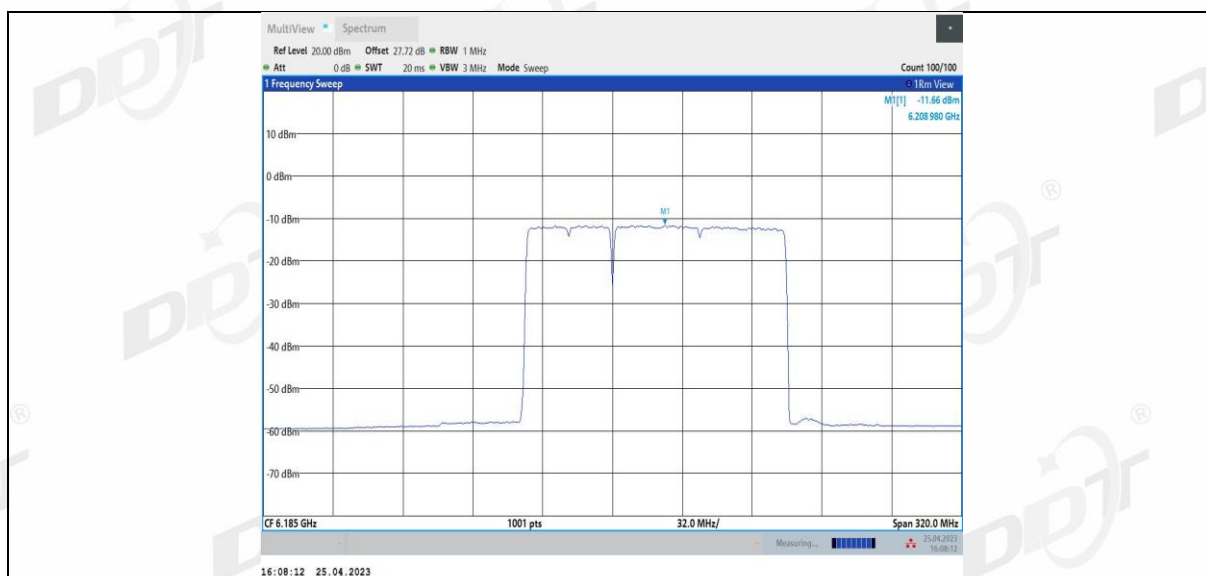
11BE160MIMO Ant3 6185 996+484 2
