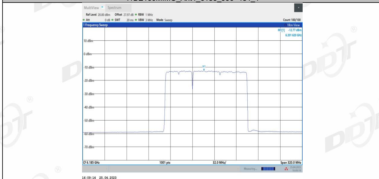
11BE160MIMO Ant4 6185 996+484 2
