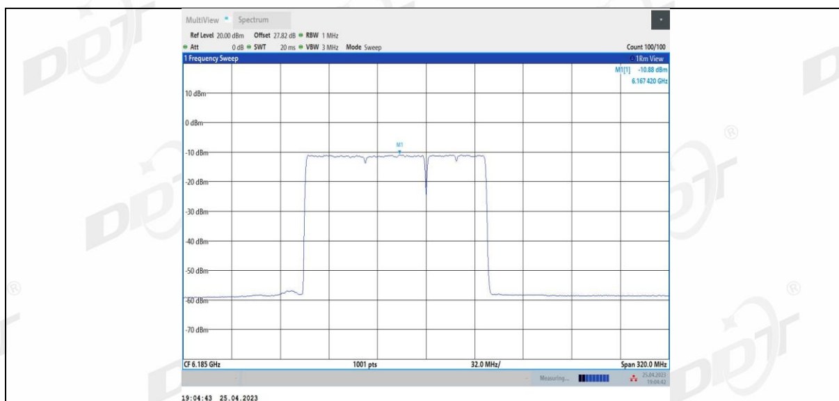
11BE160MIMO Ant3 6185 996+484+242 5
