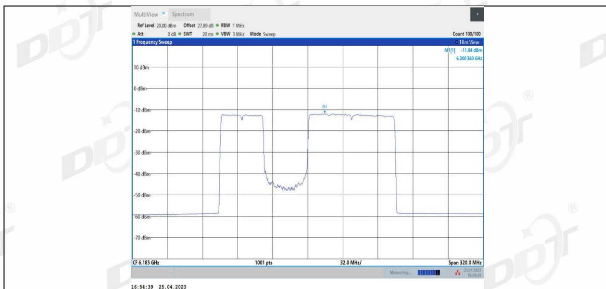
11BE160MIMO Ant1_6185_996+484_3
