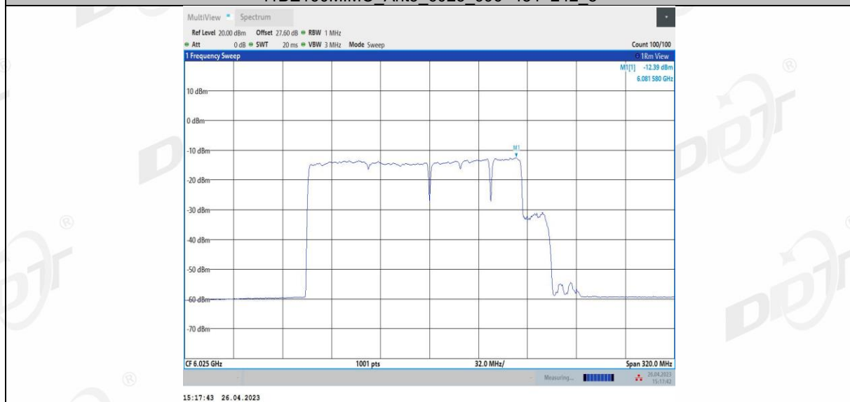
11BE160MIMO Ant4 6025_996+484_1
