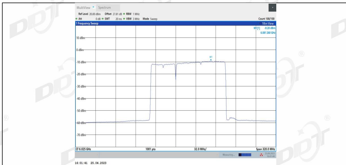
11BE160MIMO Ant1_6025_996+484_2
