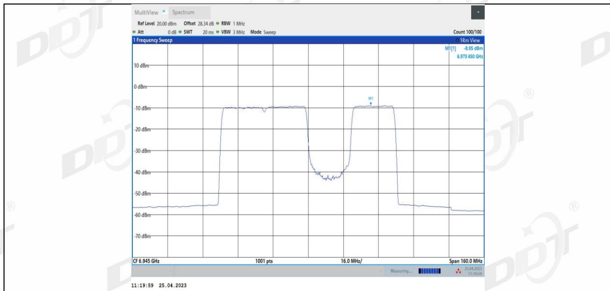
11BE80MIMO Ant1 6945 484+242 4
