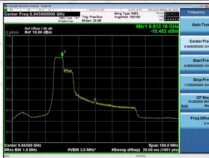
11AX80SISO-Ant1-6945-106Tone-RU53-PASS
