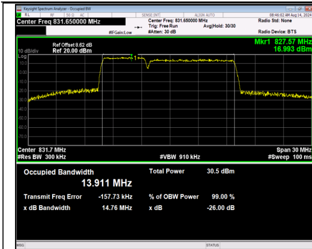
5-5-5MHz-10MHz-QPSK-QPSK-20428-20500-25RB#0-50 RB#0-PASS
