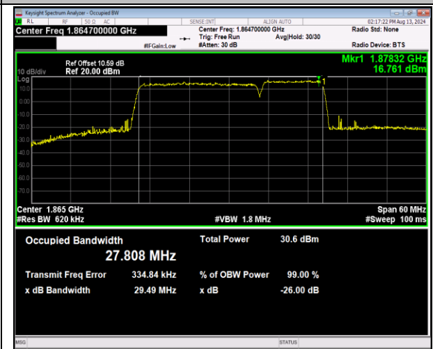
2-2-20MHz-10MHz-QPSK-QPSK-18700-18844-100RB# 0-50RB#0-PASS
