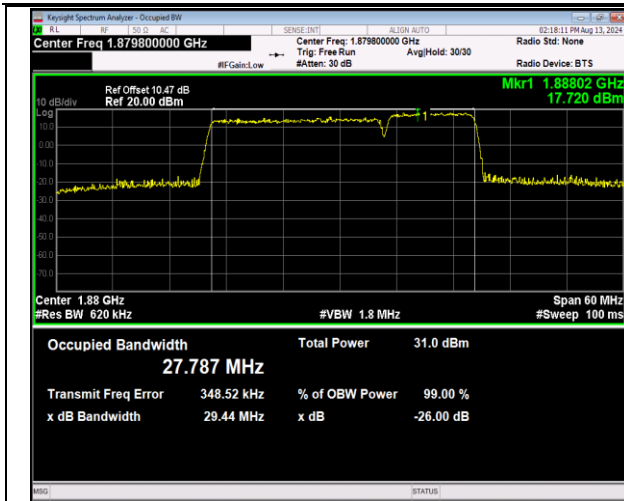
2-2-20MHz-10MHz-QPSK-QPSK-18851-18995-100RB#0-50RB#0-PASS
