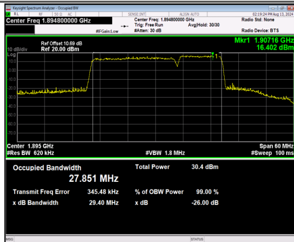
2-2-20MHz-10MHz-16QAM-16QAM-19001-19145-100RB#0-50RB#0-PASS
