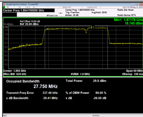
2-2-20MHz-10MHz-16QAM-16QAM-18700-18844-100RB #0-50RB#0-PASS
