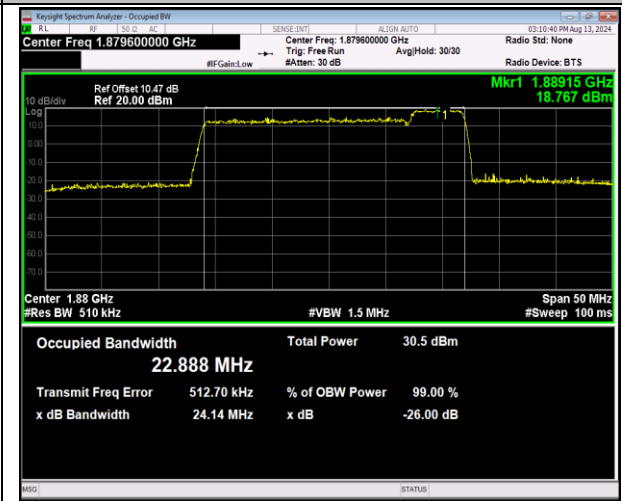
2-2-20MHz-5MHz-QPSK-QPSK-18875-18992-100RB#0- 25RB#0-PASS
