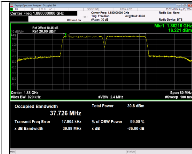
2-2-20MHz-20MHz-QPSK-QPSK-18801-18999-100RB#0-100RB#0-PASS
