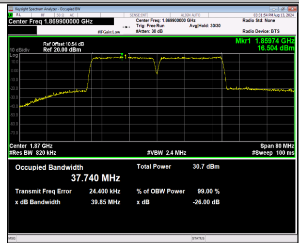
2-2-20MHz-20MHz-QPSK-QPSK-18700-18898-100RB#0-100RB#0-PASS
