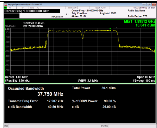
2-2-20MHz-20MHz-16QAM-16QAM-18801-18999-100RB#0-100RB#0-PASS
