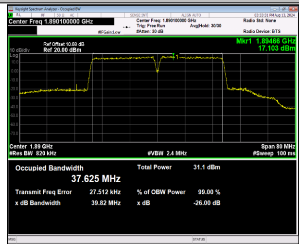
2-2-20MHz-20MHz-QPSK-QPSK-18902-19100-100RB#0-100RB#0-PASS
