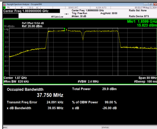
2-2-20MHz-20MHz-16QAM-16QAM-18700-18898-100RB#0-100RB#0-PASS
