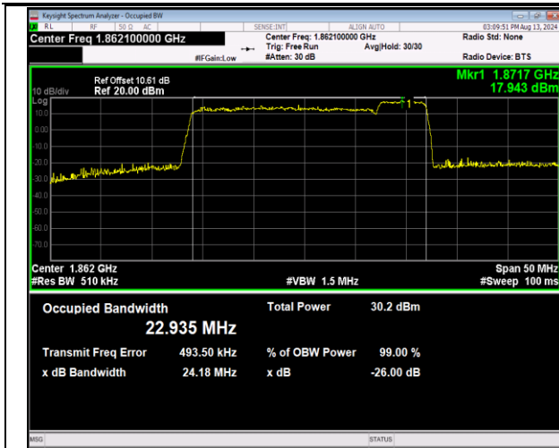
2-2-20MHz-5MHz-QPSK-QPSK-18700-18817-100RB#0-2 5RB#0-PASS
