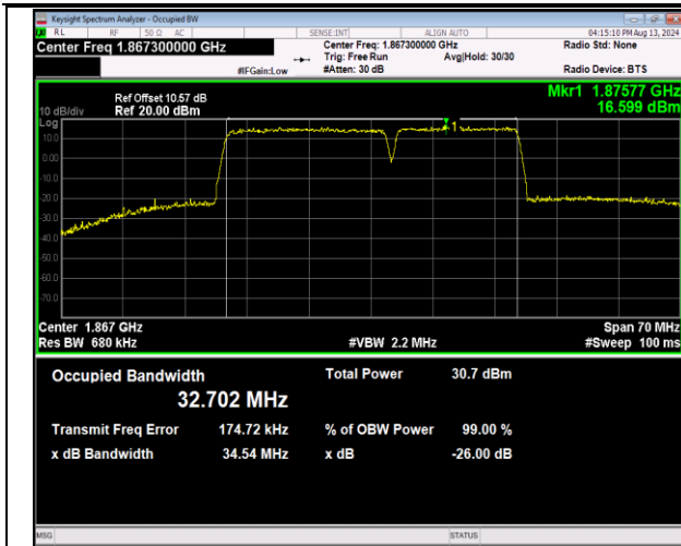
2-2-20MHz-15MHz-QPSK-QPSK-18700-18871-100RB#0-75RB#0-PASS
