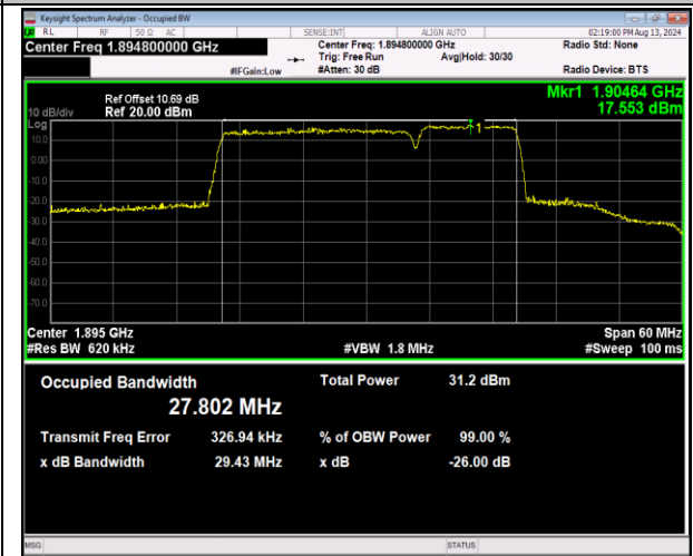
2-2-20MHz-10MHz-QPSK-QPSK-19001-19145-100RB#0-50RB#0-PASS
