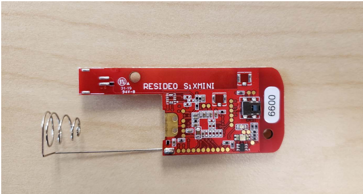
PCB Top
