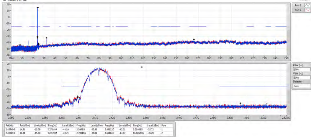
802.11b_Nss1,(1Mbps)_2TX 2437MHz
