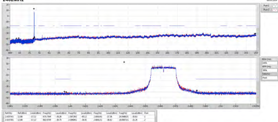
802.11g-BF_Nss1,(6Mbps)_2TX 2462MHz
