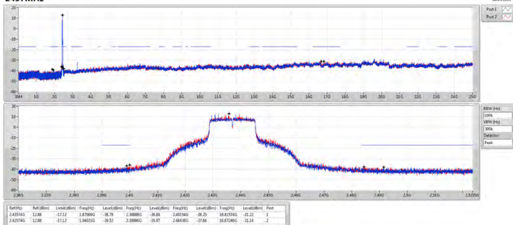
802.11g-BF_Nss1,(6Mbps)_2TX 2437MHz
