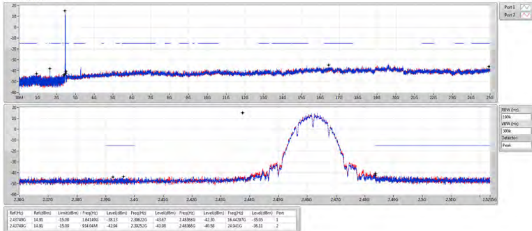
802.11b_Nss1,(1Mbps)_2TX 2462MHz
