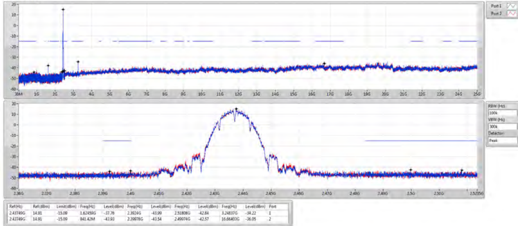
802.11b_Nss1,(1Mbps)_2TX 2437MHz
