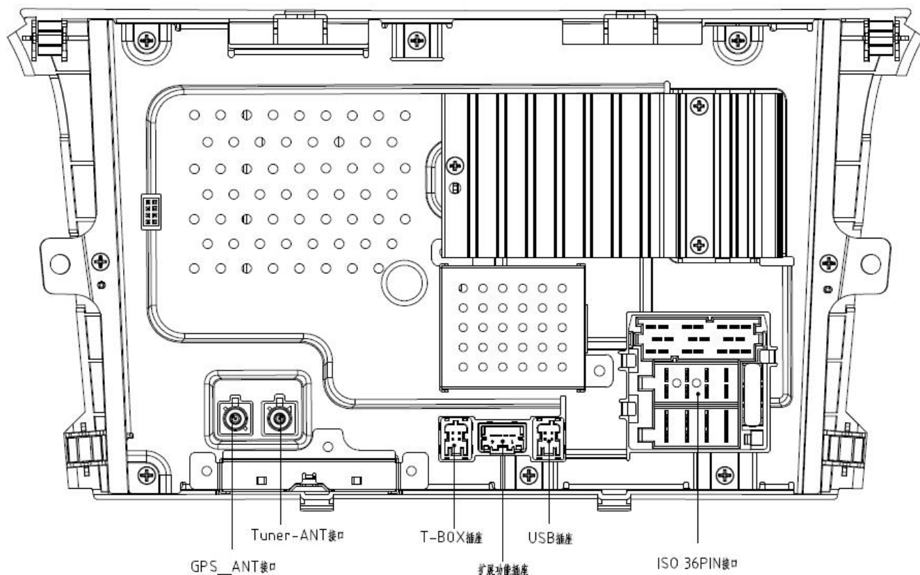
接线示意图
