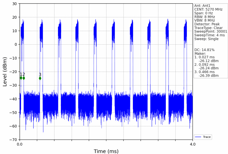
802.11ax(HEW40)_LCH_5270MHz_RU484_Left_Ant1_NTNV
