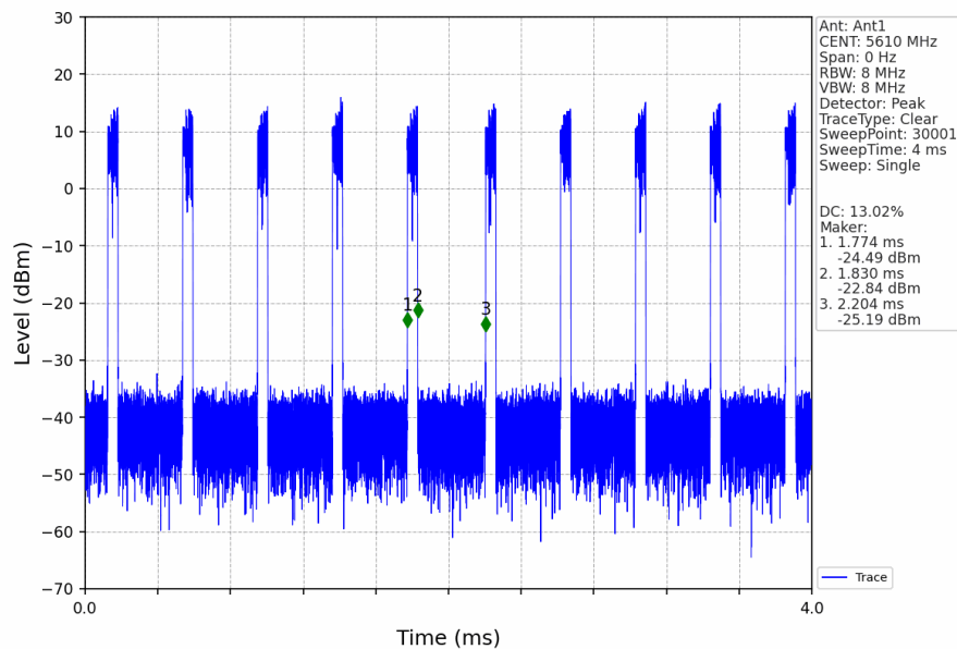
802.11ac(VHT80)_HCH_5610MHz_Ant1_NTNV
