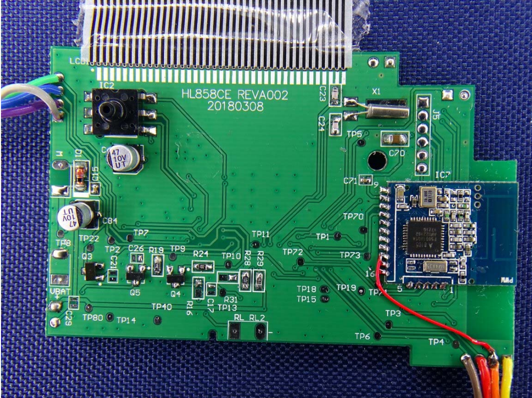
(20) EUT Photo
