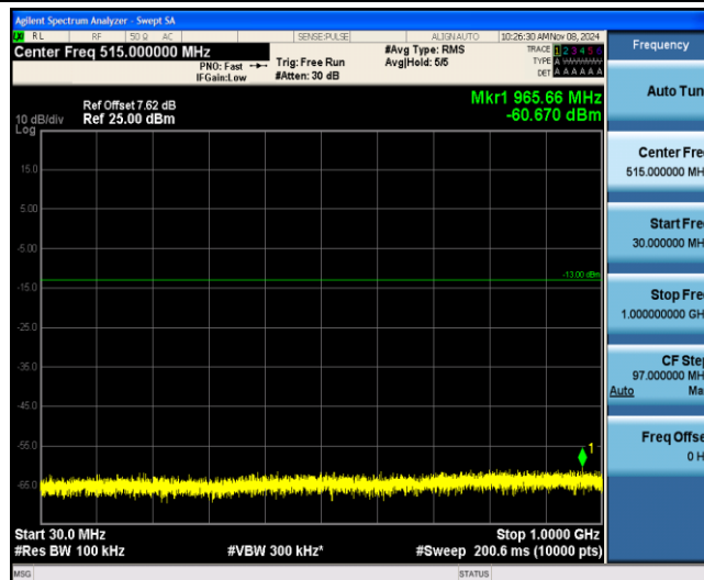
Band25-1.4MHz-QPSK-26365-1-0-Low-30-1000--60.67-PASS
