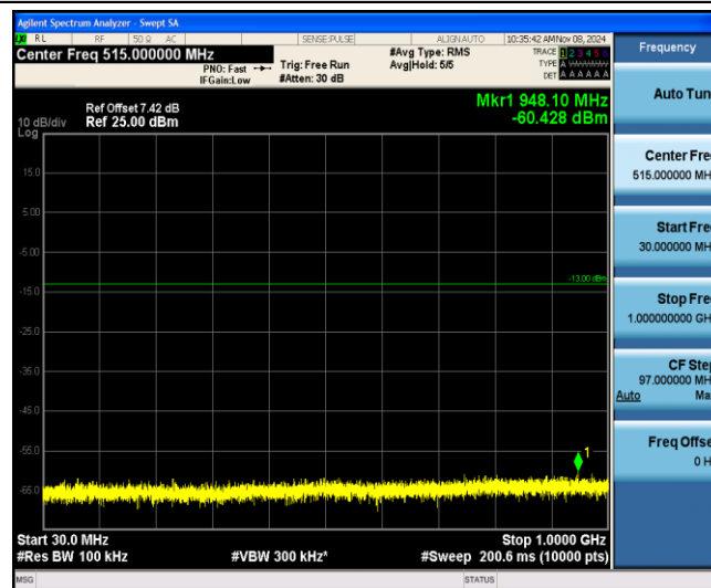
Band25-3MHz-QPSK-26675-1-0-Low-30-1000--60.43-PASS
