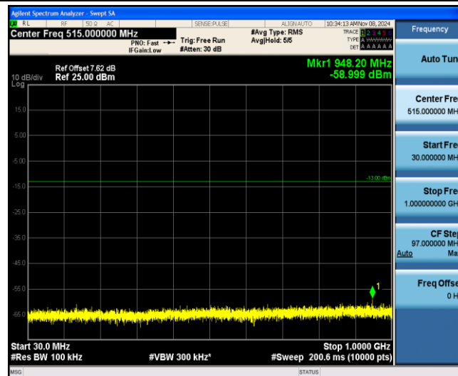
Band25-3MHz-QPSK-26365-1-0-Low-30-1000--59-PASS
