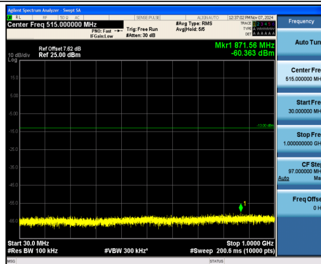
Band25-5MHz-QPSK-26365-1-0-Low-30-1000--60.36-PASS
