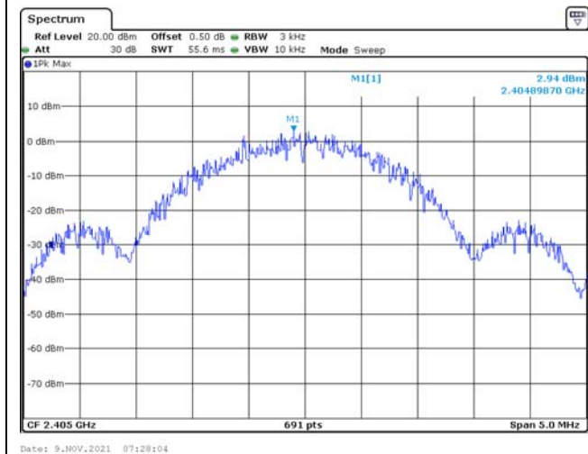
O-QPSK / 2405 MHz
