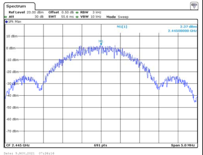
O-QPSK / 2445 MHz
