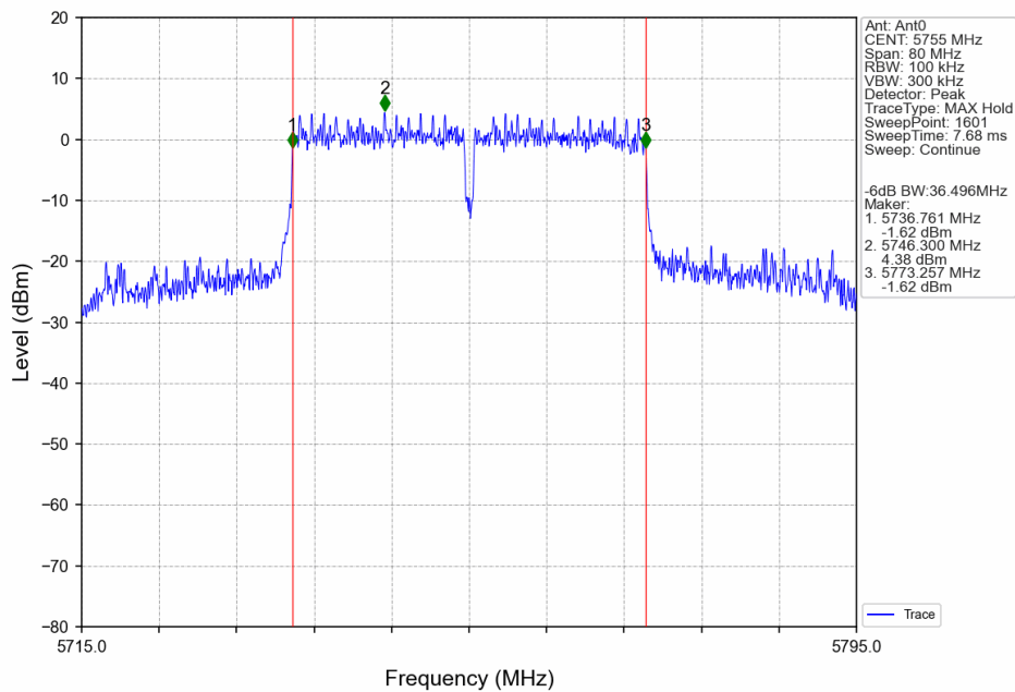
802.11ac(VHT40)_LCH_5755MHz_Ant0_NTNV
