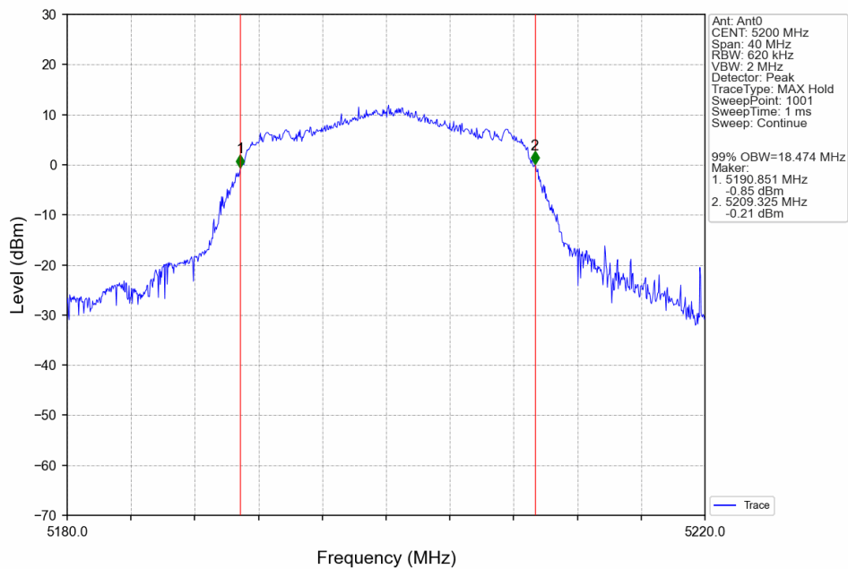
802.11n(HT20)_MCH_5200MHz_Ant0_NTNV
