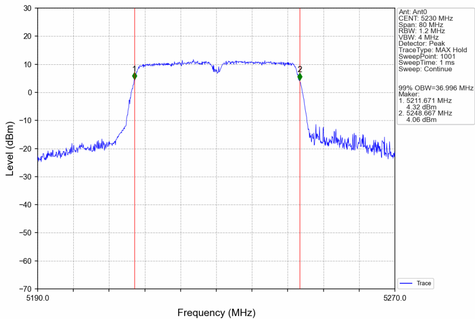
802.11ax(HEW40)_HCH_5230MHz_SU_Ant0_NTNV
