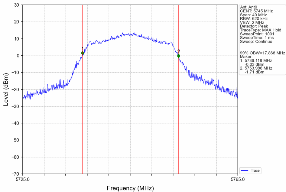
802.11a_LCH_5745MHz_Ant0_NTNV
