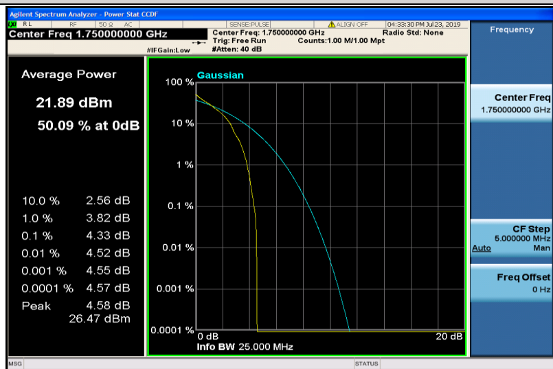
Band4-10MHz-QPSK-20350-1RB#0
