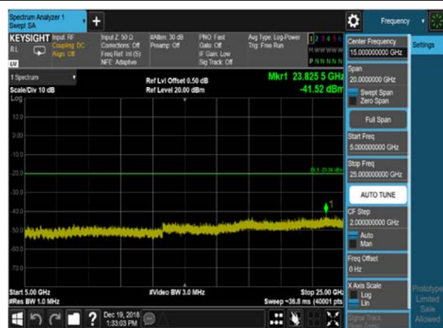
2402MHz,Plot 5,5000MHz~25000MHz
