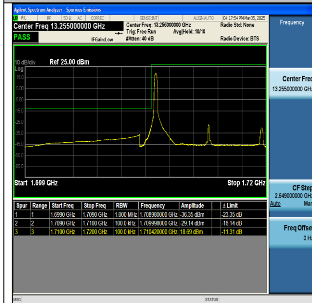
NTNV-n66-PC3-15-10-L-CP-QPSK-Edge_1RB_Left-PASS
