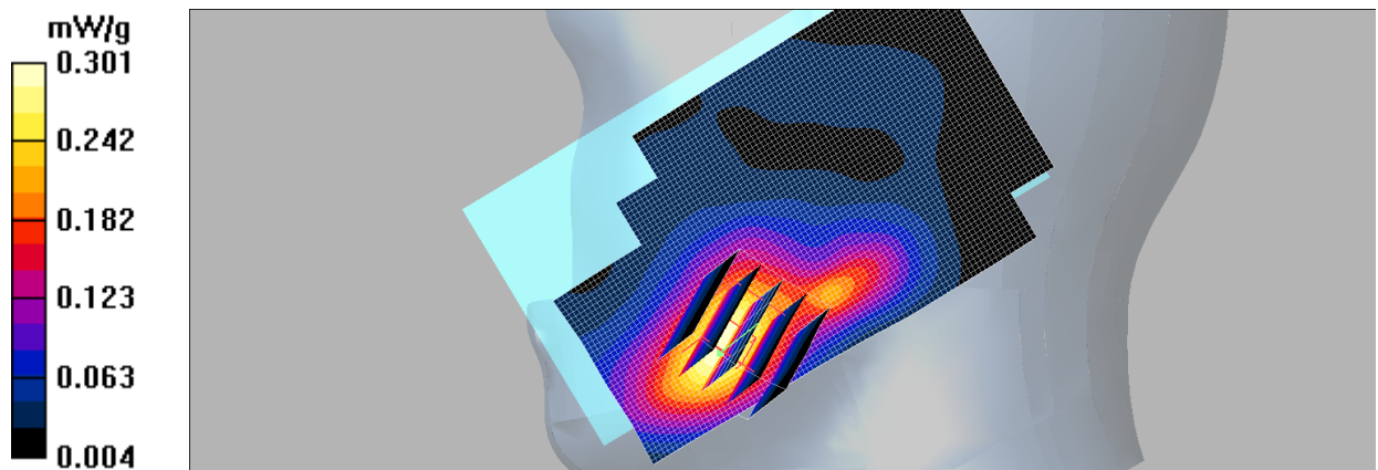
Fig.7 WCDMA1900 CH9538
