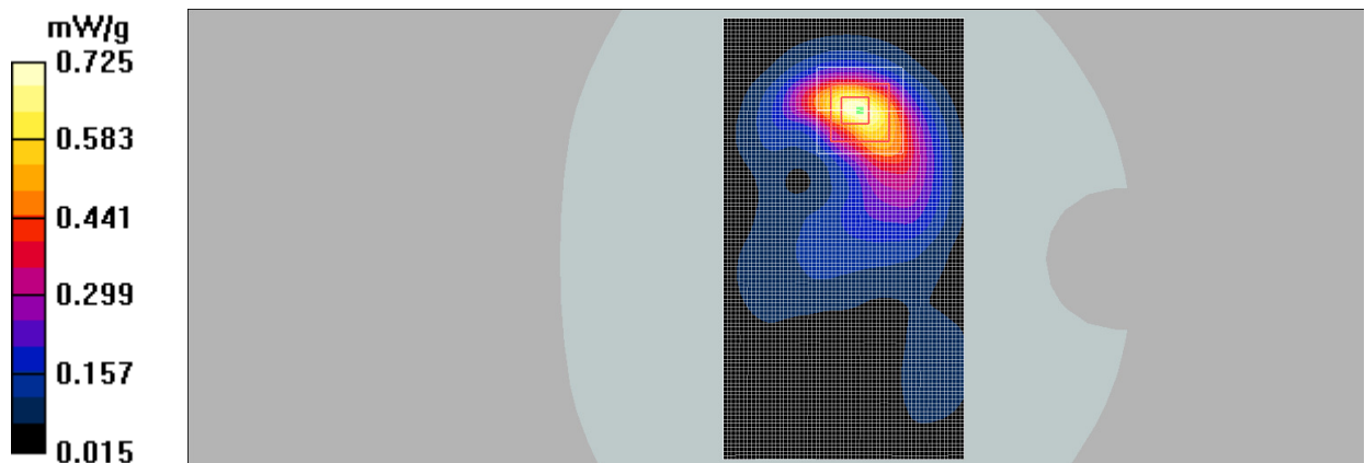
Fig.8 WCDMA1900 CH9538
