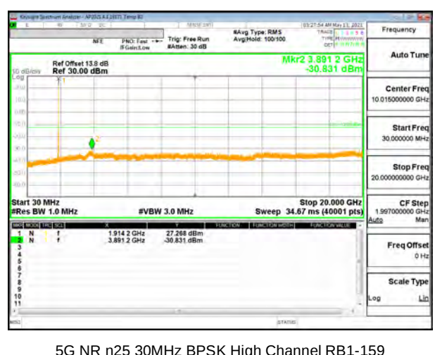
5G NR n25 30MHz BPSK High Channel RB1-159
