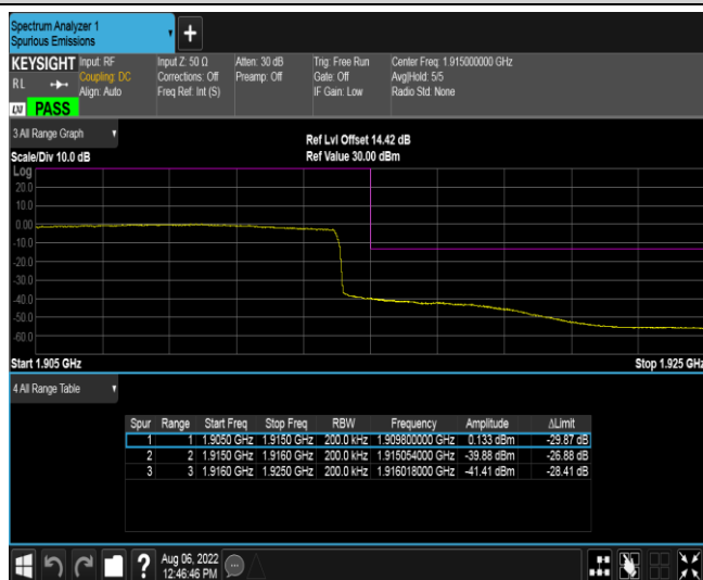
Band25-20MHz-QPSK-26590-100RB#0
