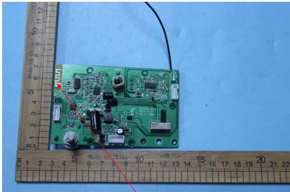
Antenna
