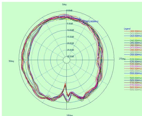
\Phi=90^\circ YZ面
