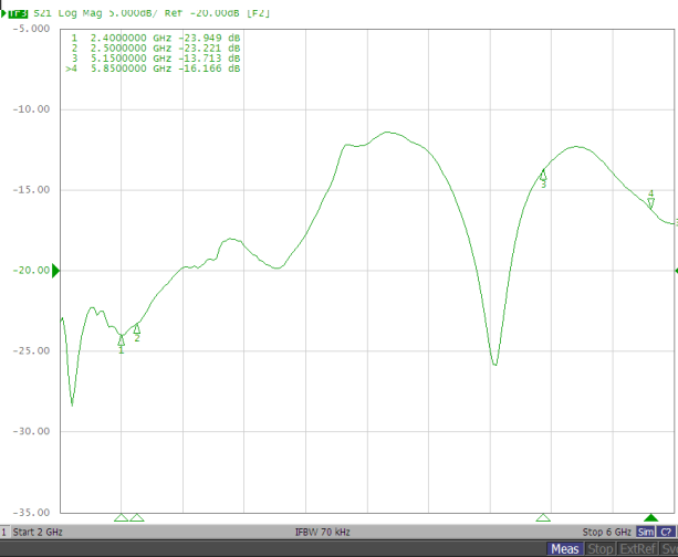
BT&WIFI1
