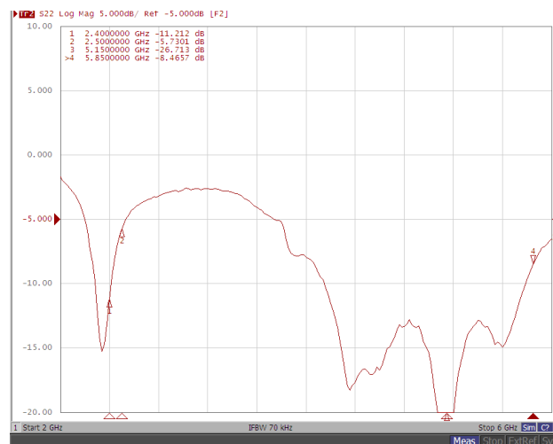
WIFI1
