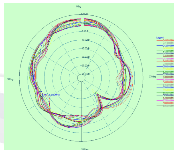
\Theta=90^\circ XY面
