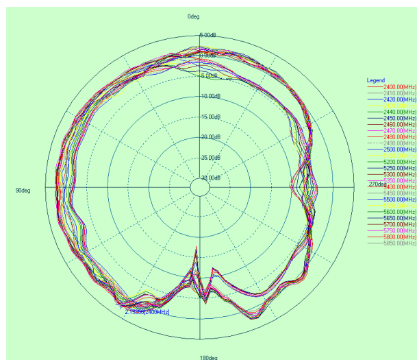
\Phi=0^\circ XZ面
