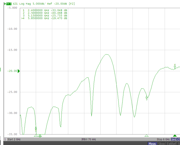
BT&WIFI2
