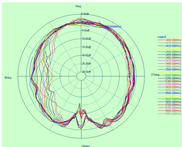
\Phi=0^\circ XZ面
