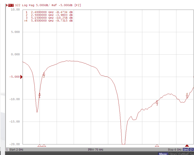
WIFI2
