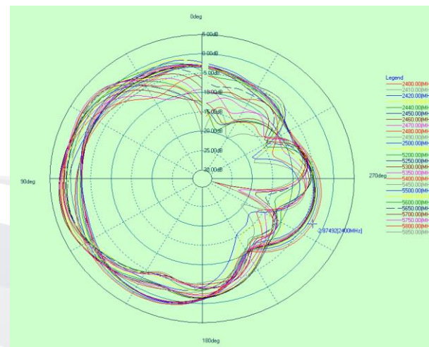
\Theta=90^\circ XY面
