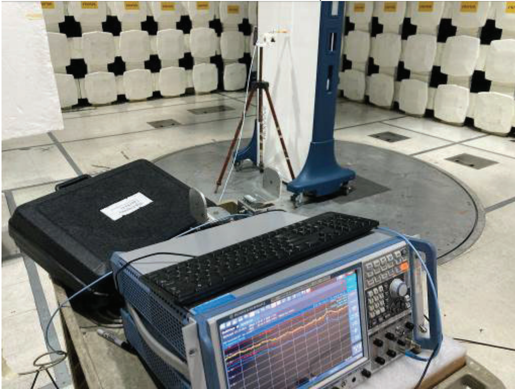
60-90 GHz Test Setup
