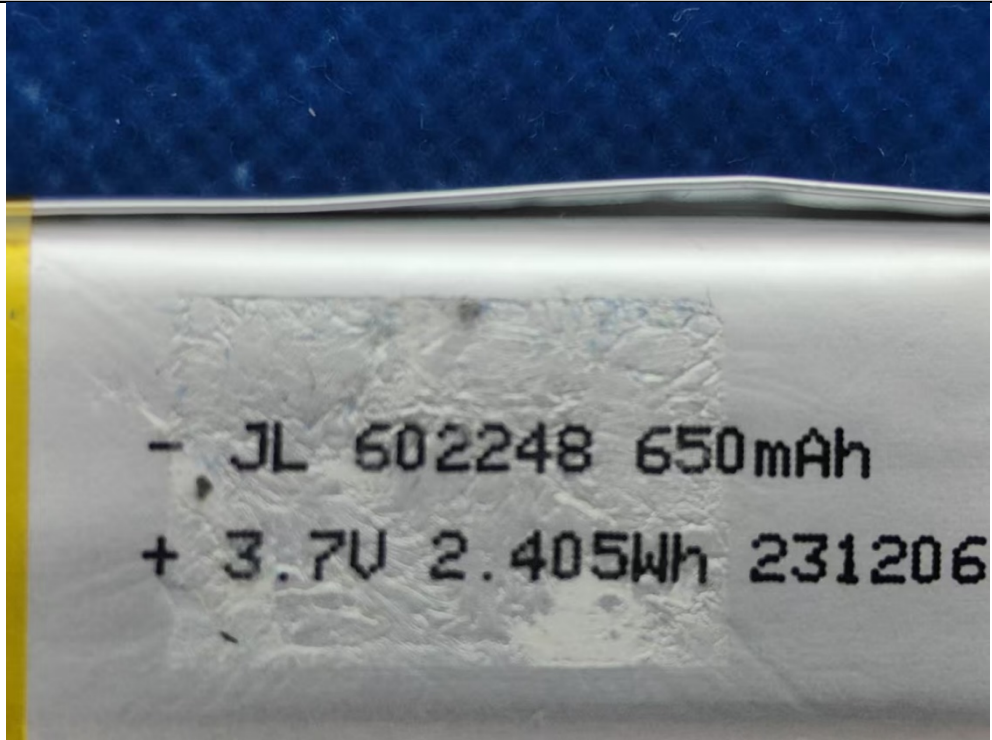
EUT Photo
