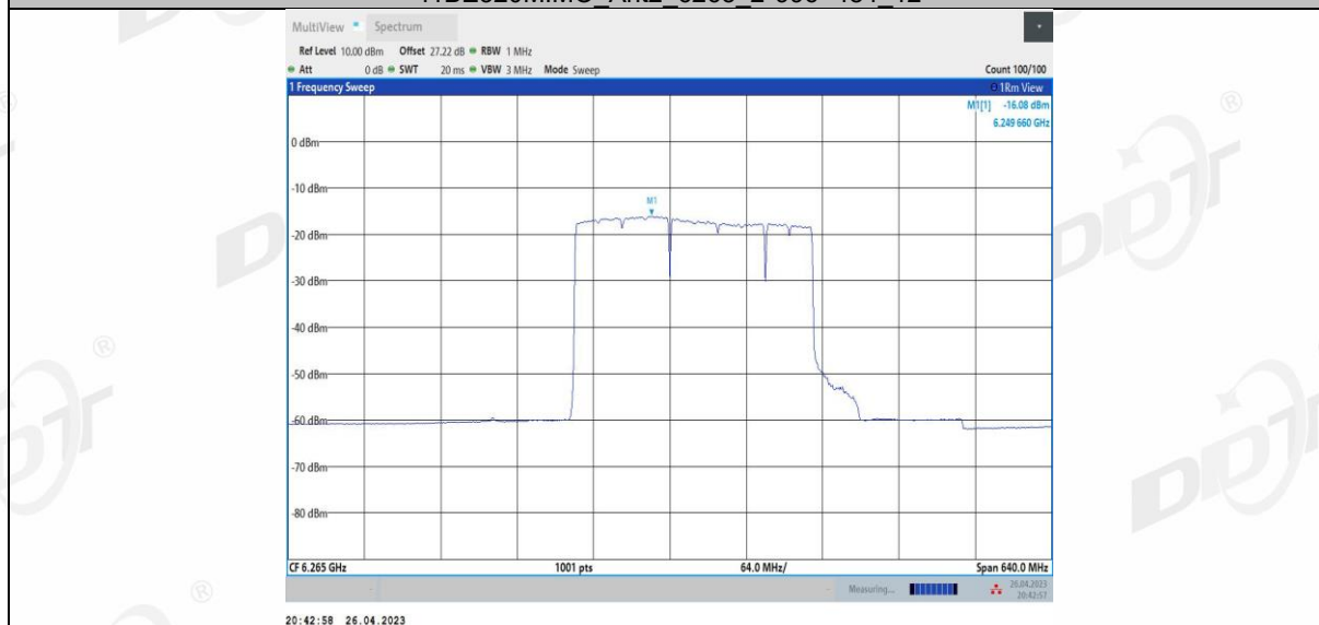
11BE320MIMO_Ant2_6265_3*996_1
