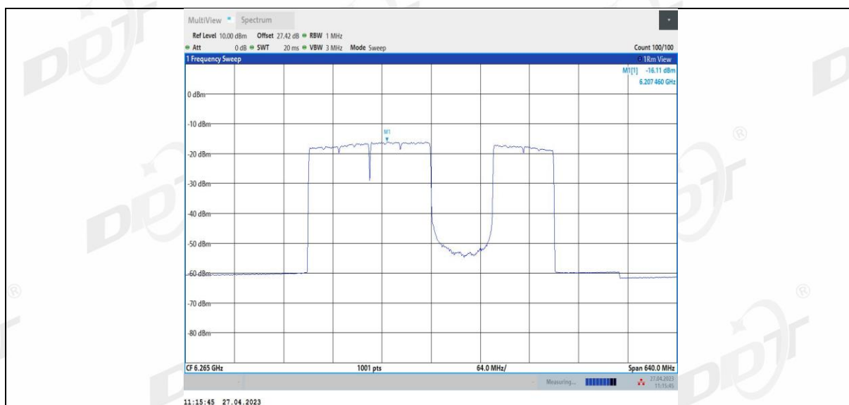
11BE320MIMO Ant4 6265 3*996 4
