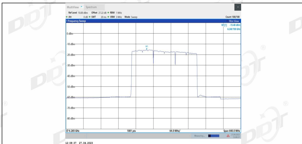
11BE320MIMO Ant2 6265 3*996 2
