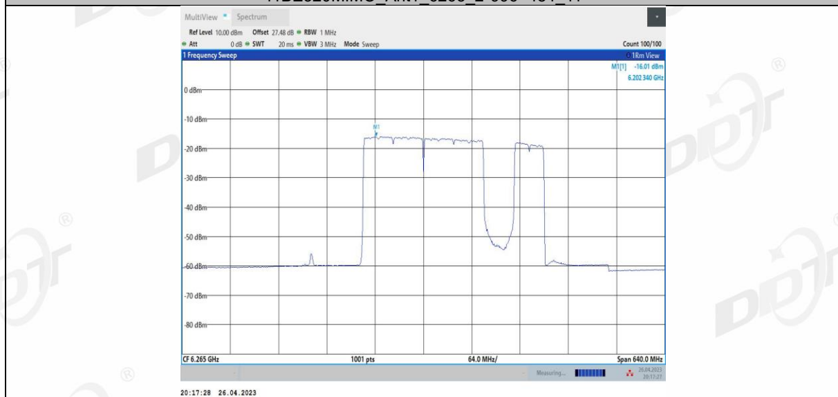
11BE320MIMO Ant1_6265_2*996+484_12
