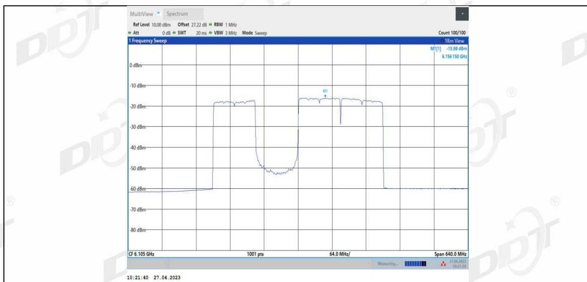
11BE320MIMO Ant4 6105 3*996 3
