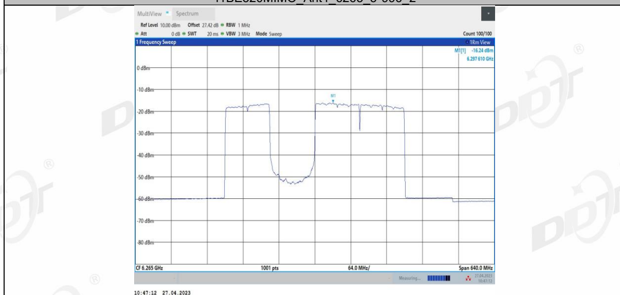
11BE320MIMO_Ant4_6265_3*996_3
