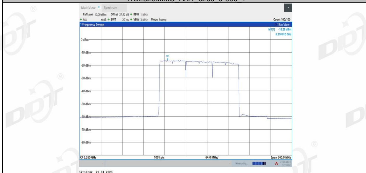
11BE320MIMO_Ant4_6265_3*996_2
