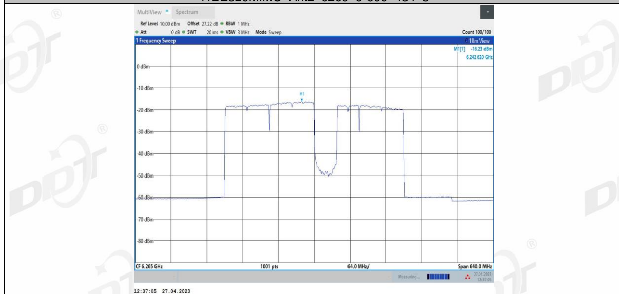
11BE320MIMO Ant2 6265 3*996+484 6
