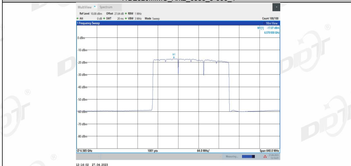
11BE320MIMO_Ant2_6585_3*996_2
