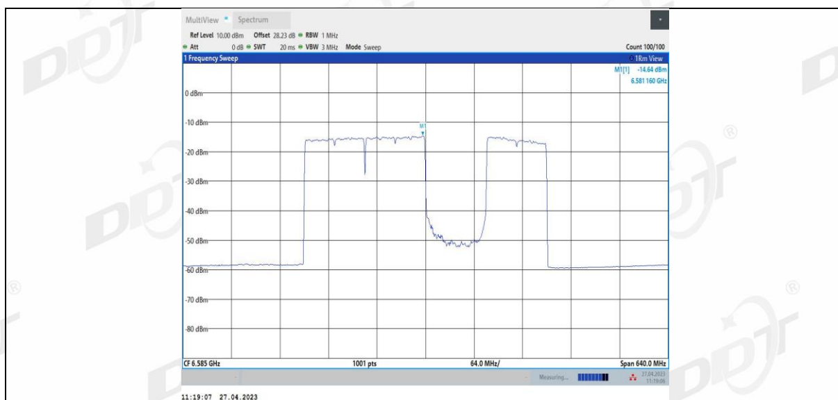
11BE320MIMO Ant3 6585 3*996 4
