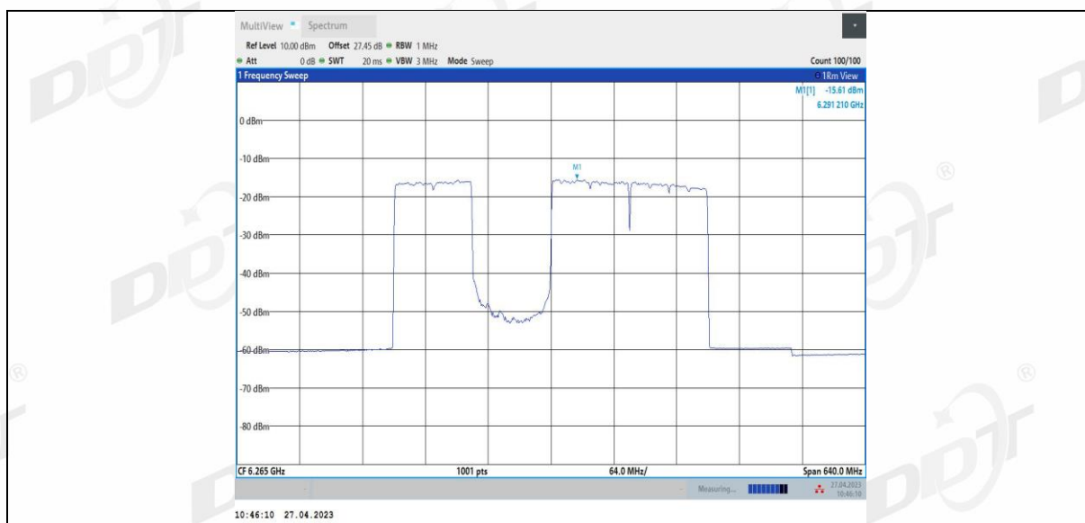
11BE320MIMO Ant3 6265 3*996 3
