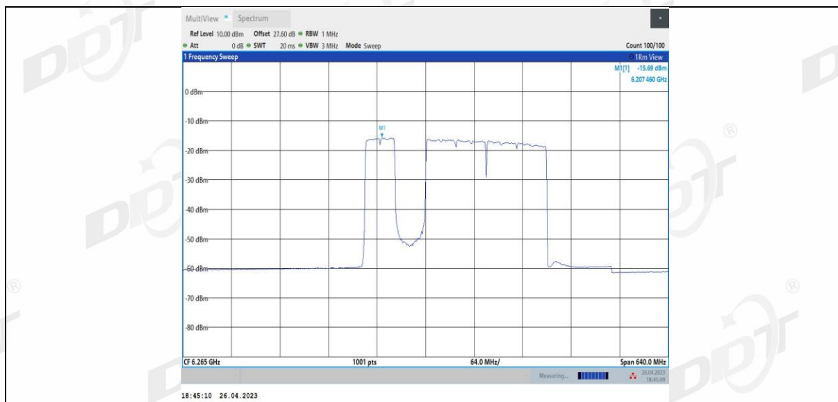
11BE320MIMO Ant3 6265 2*996+484 9
