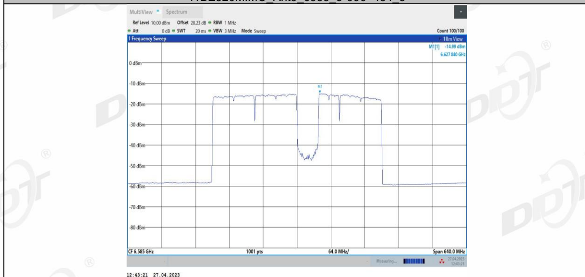
11BE320MIMO Ant3 6585 3*996+484 6
