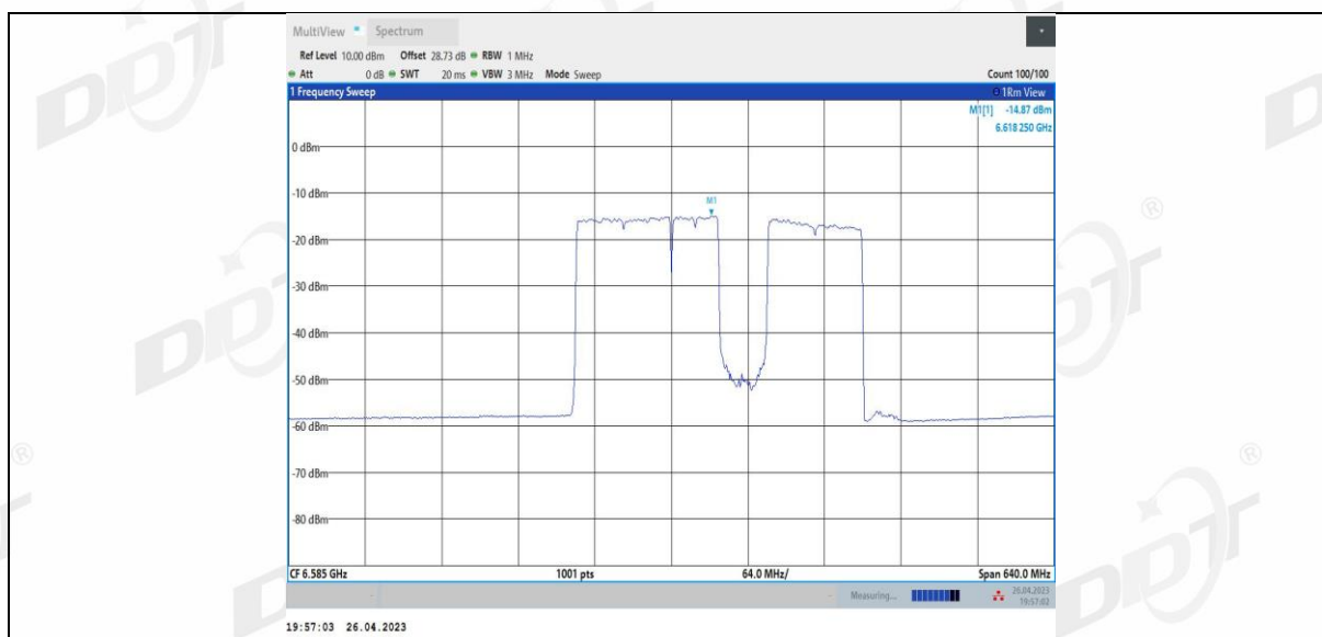
11BE320MIMO_Ant1_6585_2*996+484_11
