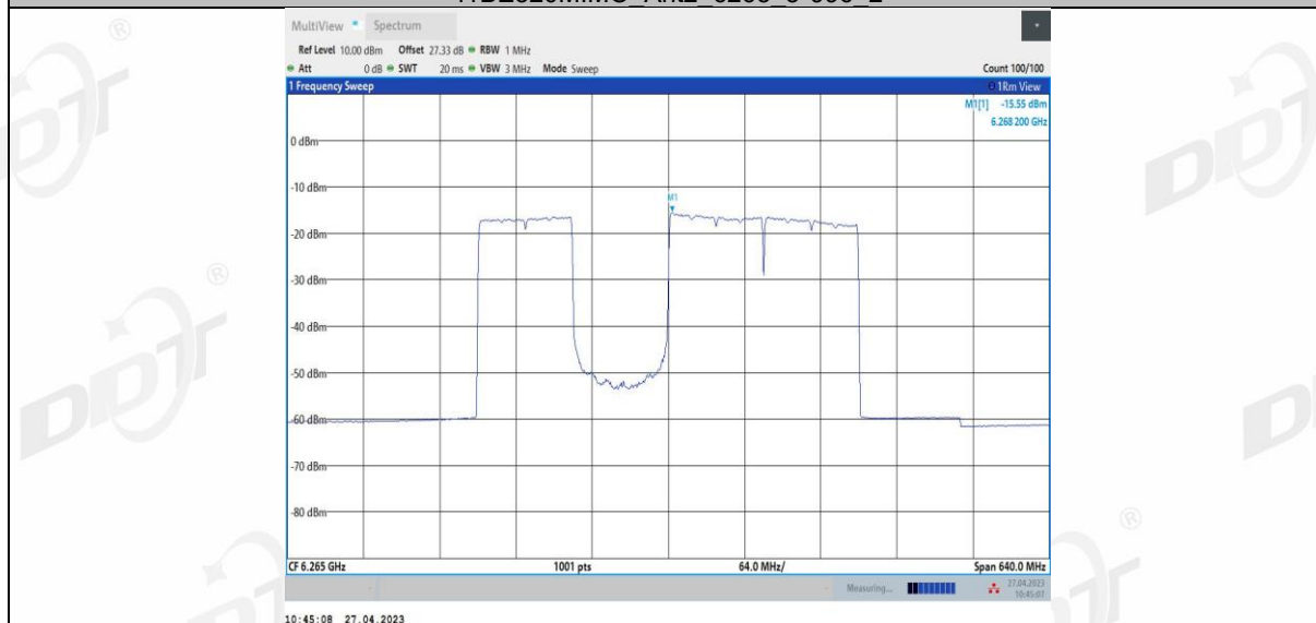
11BE320MIMO Ant2 6265 3*996 3
