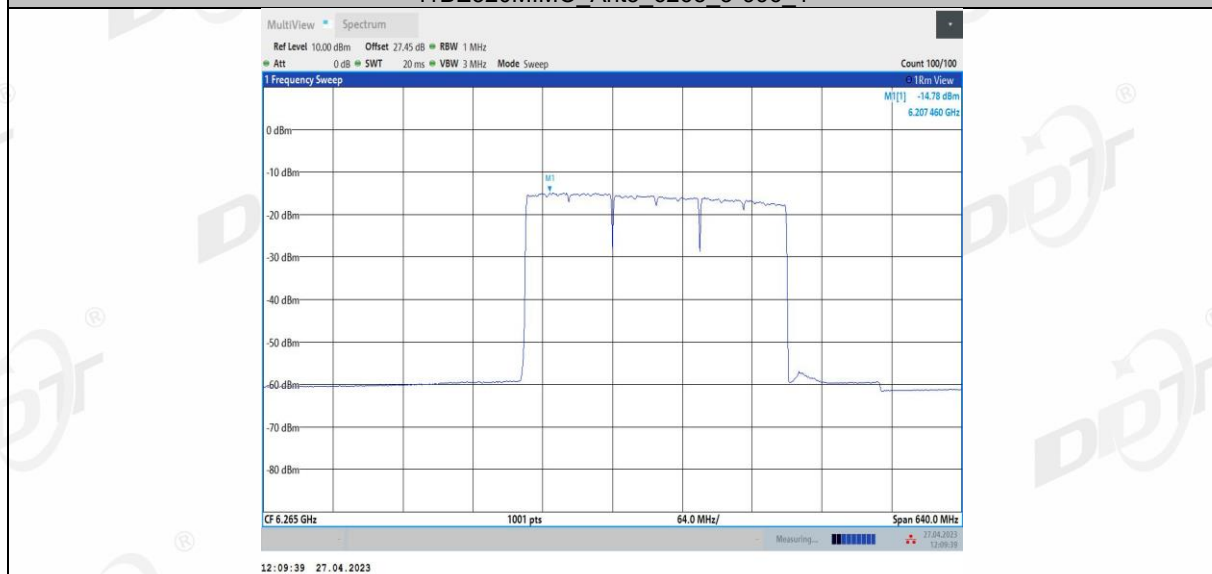
11BE320MIMO_Ant3_6265_3*996_2
