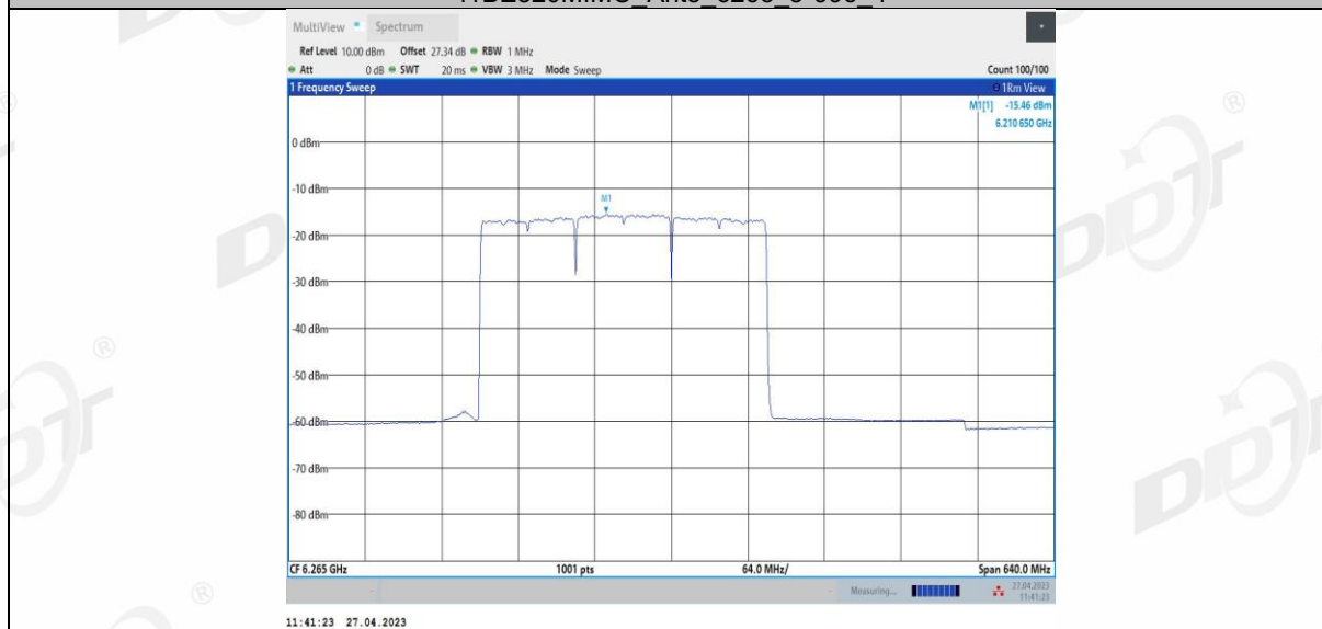
11BE320MIMO Ant3 6265 3*996+484 5
