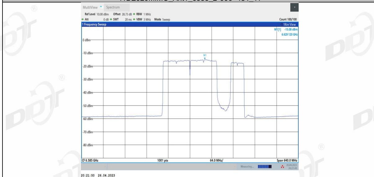
11BE320MIMO_Ant1_6585_2*996+484_12
