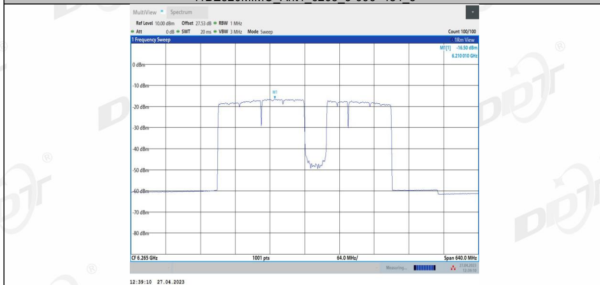
11BE320MIMO Ant4 6265 3*996+484 6
