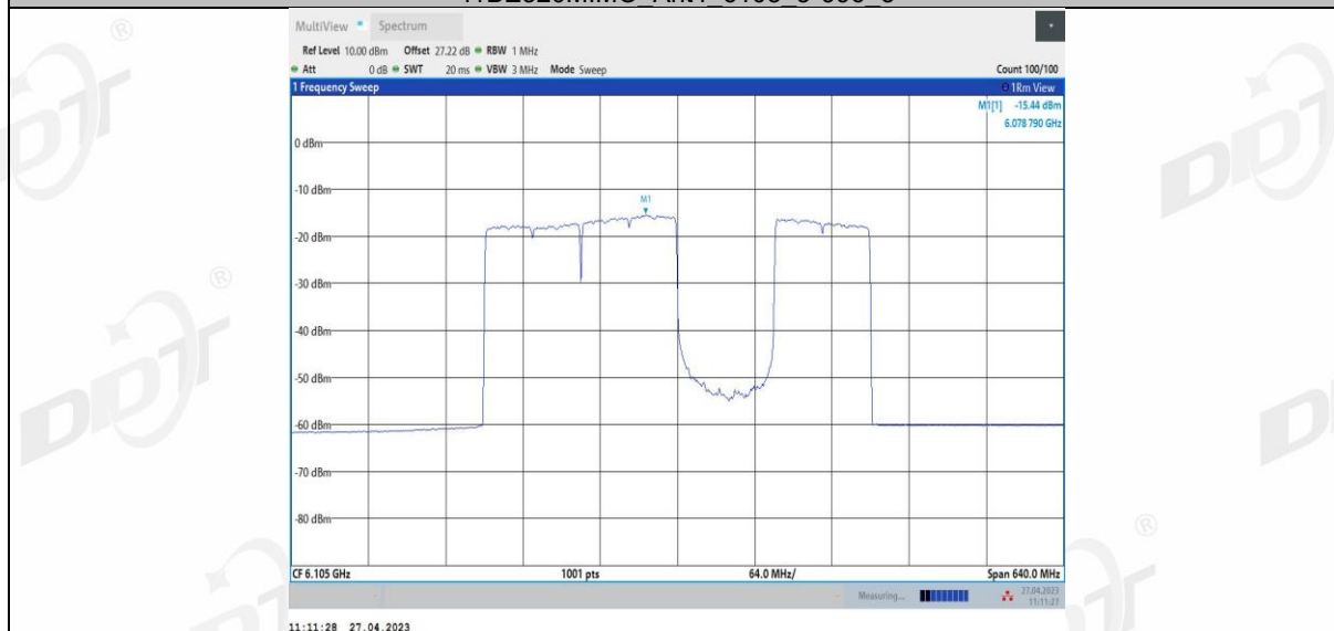
11BE320MIMO Ant4 6105 3*996 4
