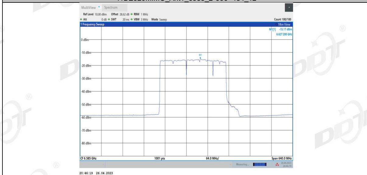
11BE320MIMO_Ant1_6585_3*996_1
