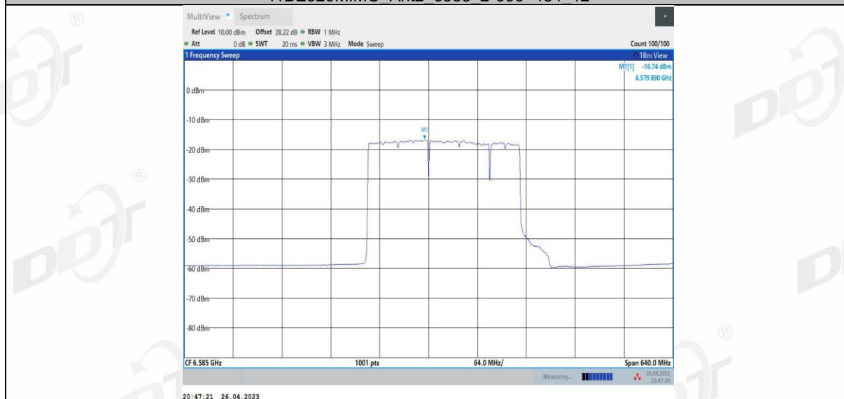
11BE320MIMO_Ant2_6585_3*996_1
