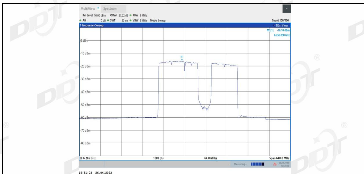
11BE320MIMO_Ant2_6265_2*996+484_11
