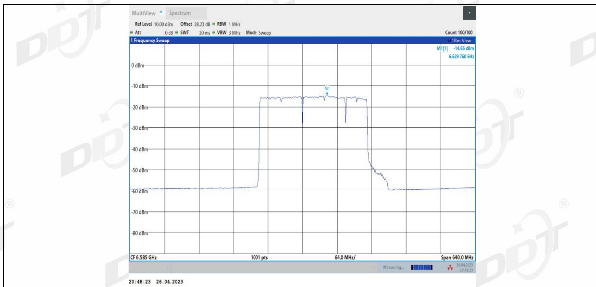
11BE320MIMO_Ant3_6585_3*996_1
