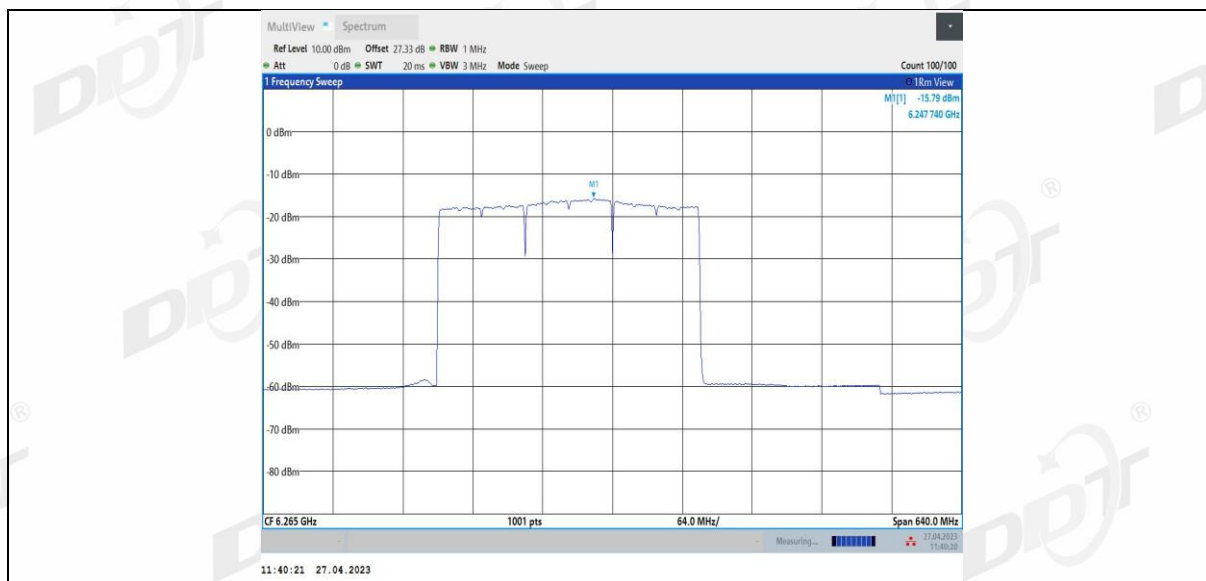
11BE320MIMO Ant2 6265 3*996+484 5
