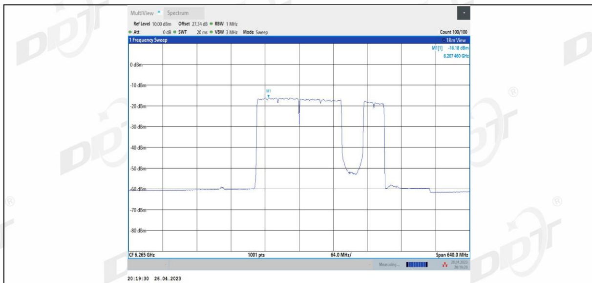
11BE320MIMO_Ant3_6265_2*996+484_12
