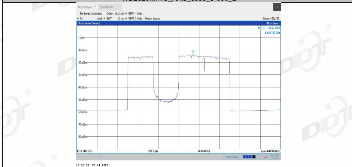
11BE320MIMO_Ant3_6585_3*996_3
