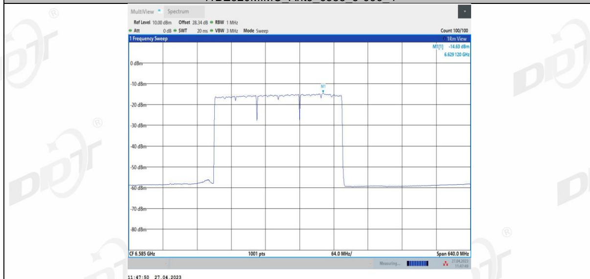
11BE320MIMO Ant3 6585 3*996+484 5
