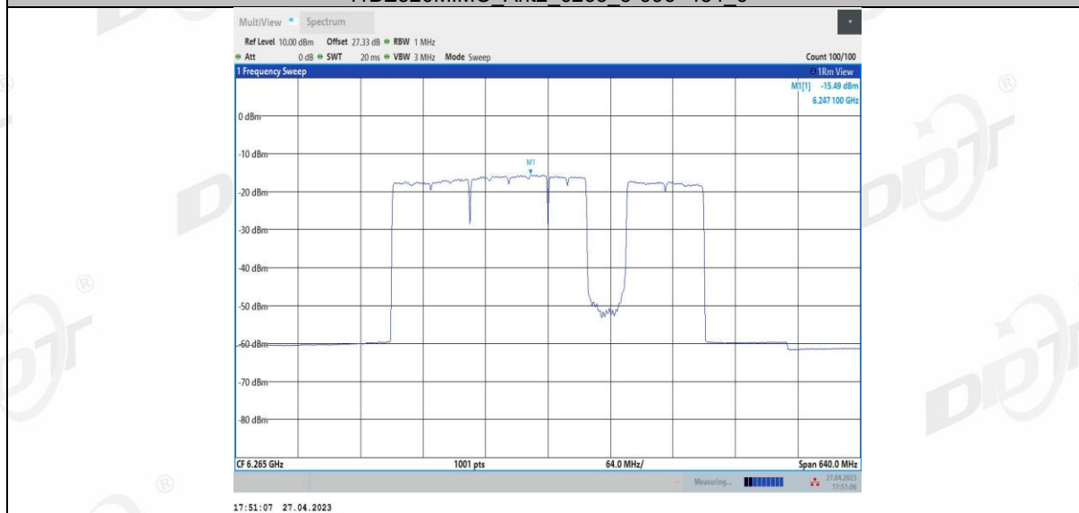
11BE320MIMO Ant2 6265 3*996+484 7
