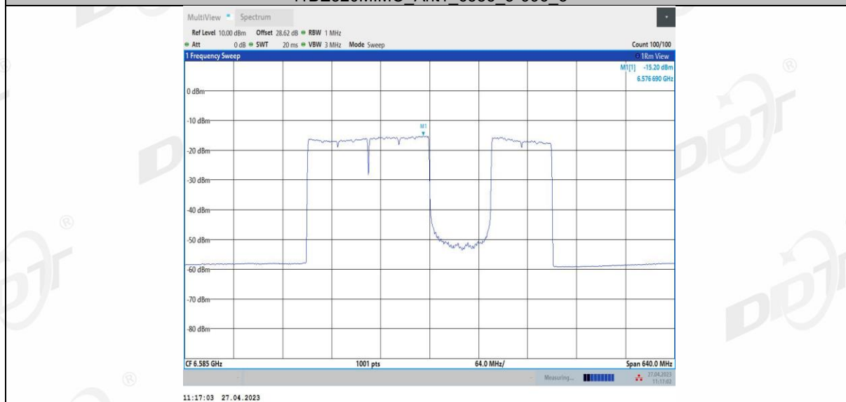
11BE320MIMO Ant1_6585_3*996_4
