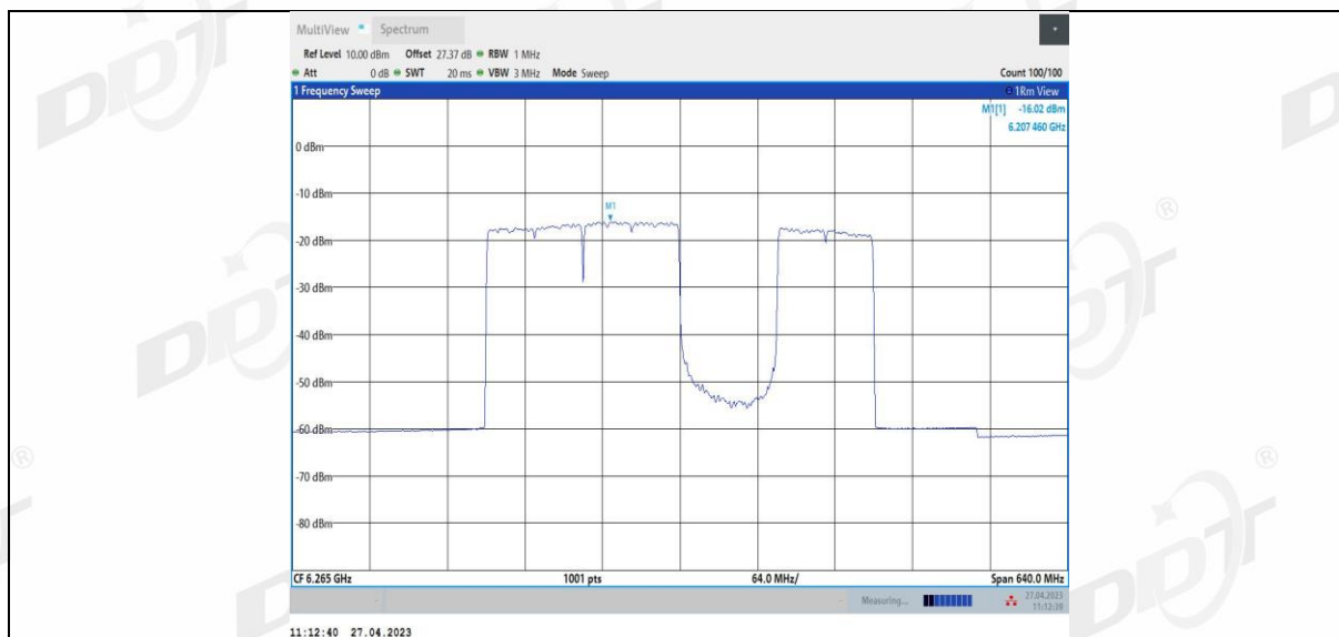
11BE320MIMO Ant1 6265 3*996 4
