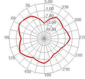
5850.000MHz H
