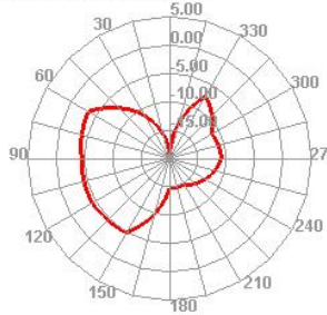
5490.000MHz E1
