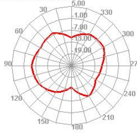
5150.000MHz H
