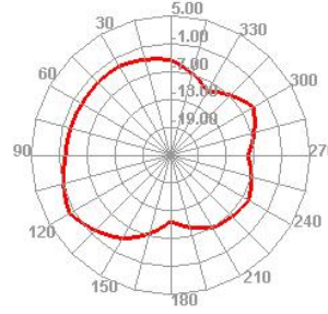
5490.000MHz E2
