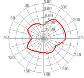
5850.000MHz E1
