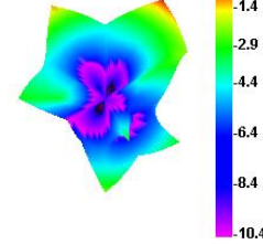
5850.000MHz E1
