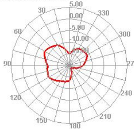
5150.000MHz E1
