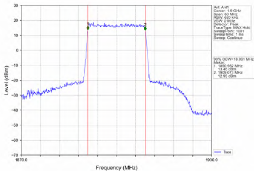
Band2_20MHz_16QAM_HCH_1900MHz_RB_100_0_NTNV
