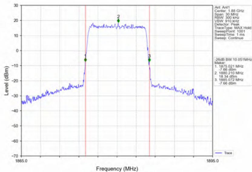
Band2_10MHz_QPSK_MCH_1880MHz_RB_50_0_NTNV
