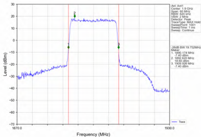
Band2_20MHz_16QAM_HCH_1900MHz_RB_100_0_NTNV
