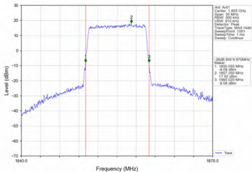
Band2_10MHz_16QAM_LCH_1855MHz_RB_50_0_NTNV
