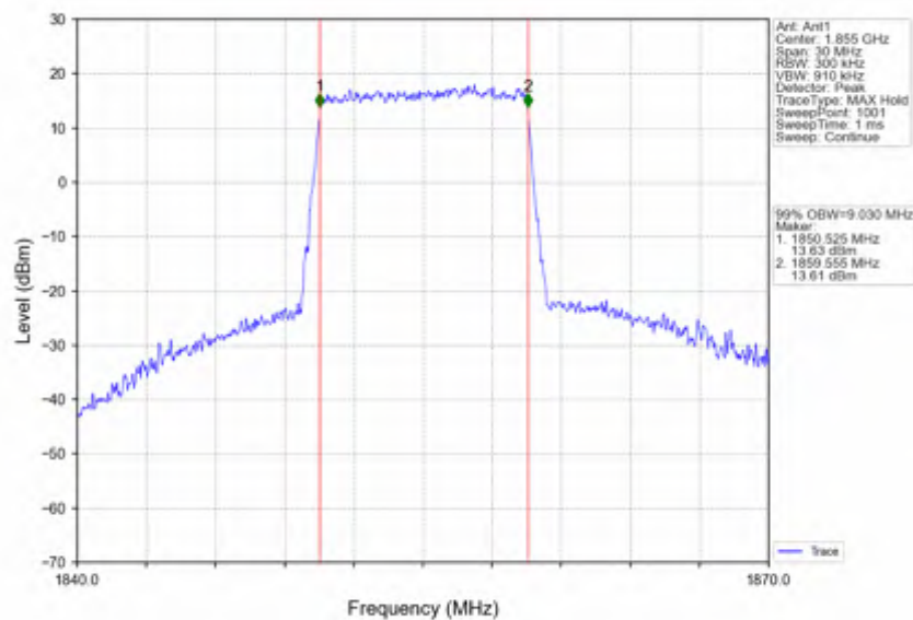
Band2_10MHz_16QAM_LCH_1855MHz_RB_50_0_NTNV
