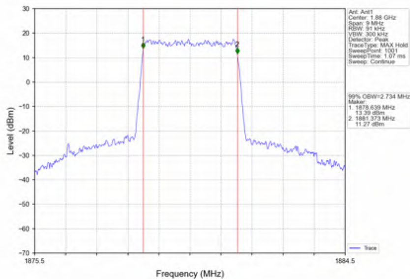
Band2_3MHz_QPSK_MCH_1880MHz_RB_15_0_NTNV
