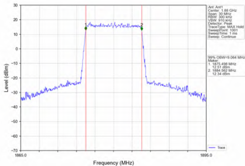
Band2_10MHz_QPSK_MCH_1880MHz_RB_50_0_NTNV
