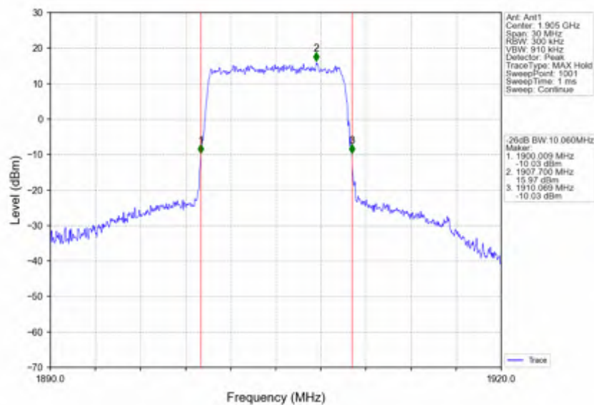
Band2_10MHz_256QAM_HCH_1905MHz_RB_50_0_NTNV
