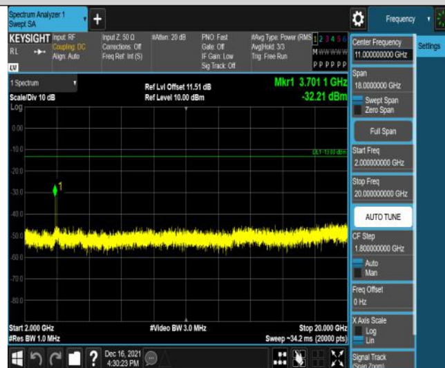
Band2-3MHz-QPSK-18615-15RB#0-Range3:2000~20000MHz
