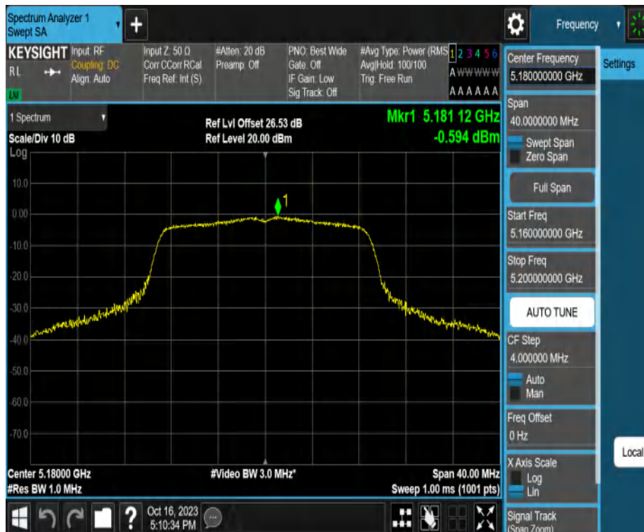
11AC20MIMO_Ant2_5180
