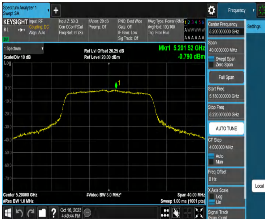
11N20MIMO_Ant2_5200
