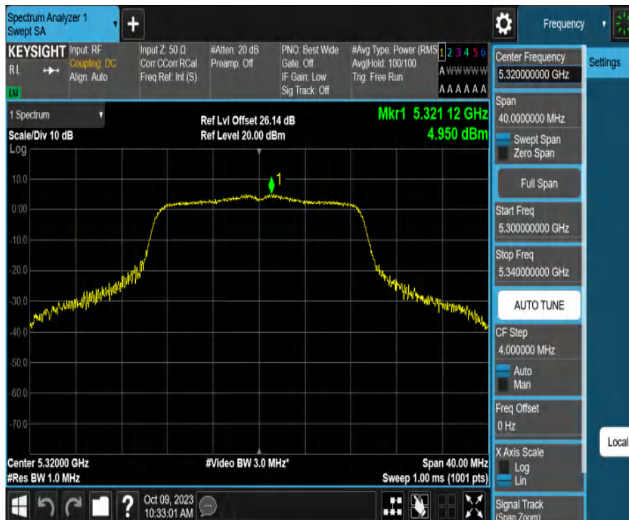
11AC20MIMO_Ant2_5320
