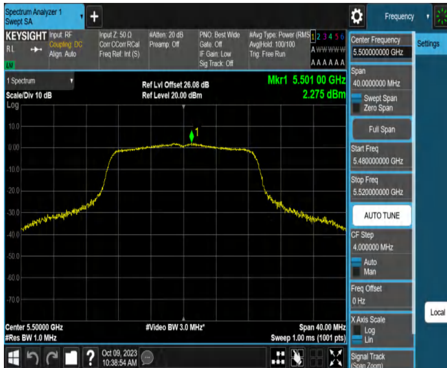
11AC20MIMO_Ant2_5500
