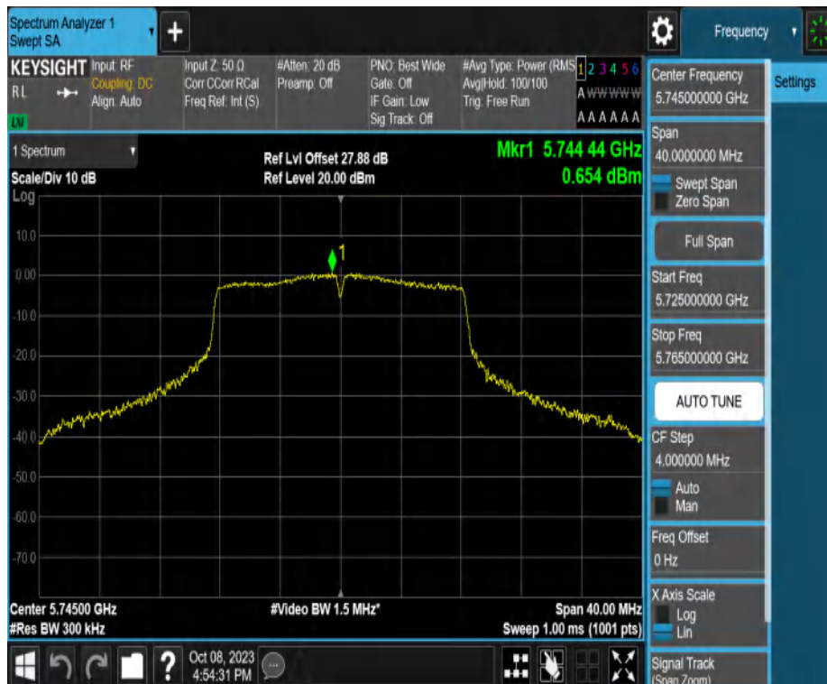
11A-CDD_Ant2_5745
