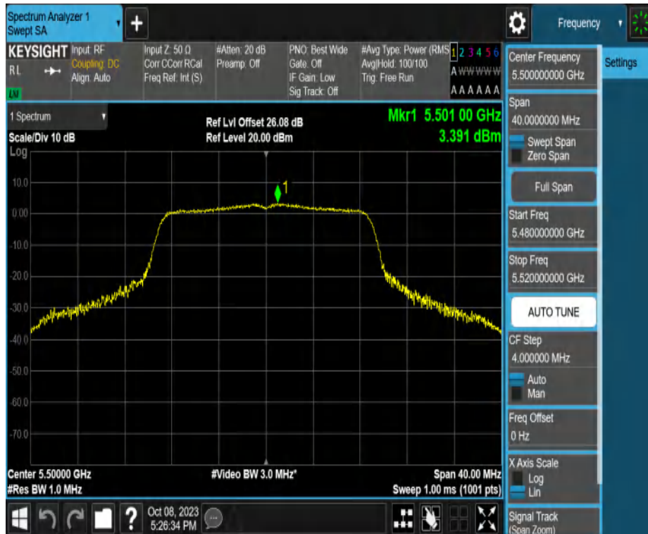
11N20MIMO_Ant2_5500
