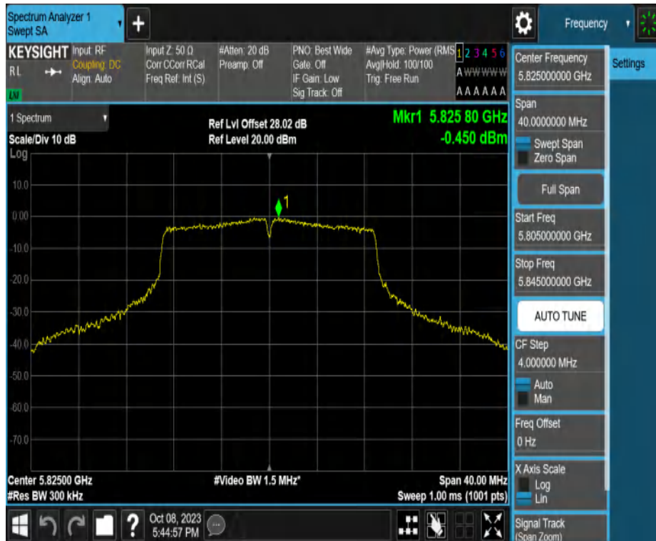
11N20MIMO_Ant2_5825
