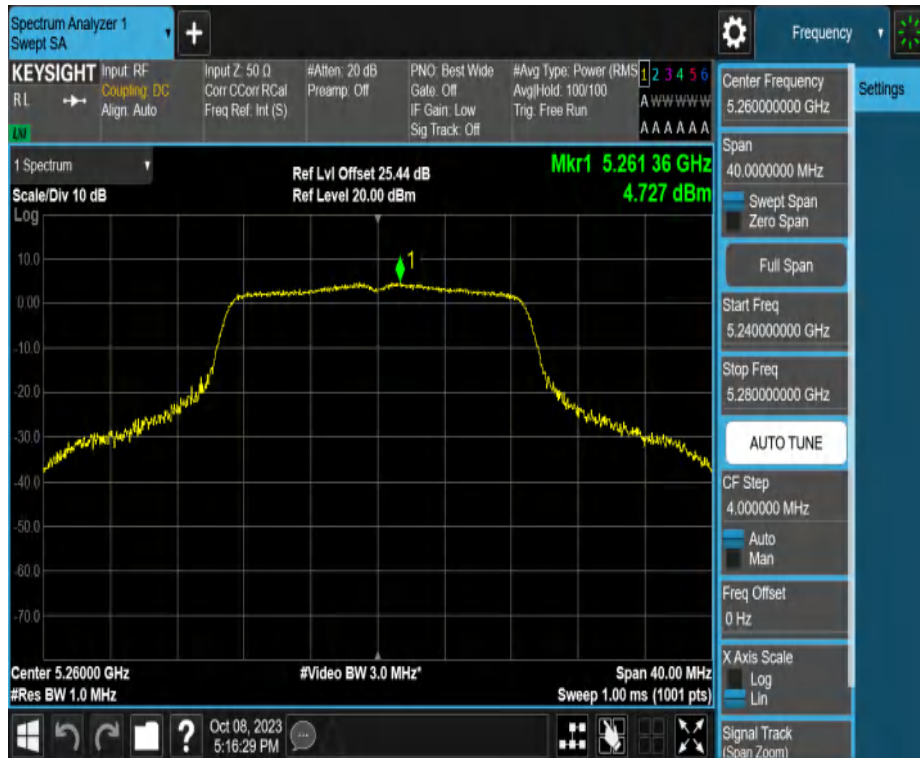
11N20MIMO_Ant2_5260
