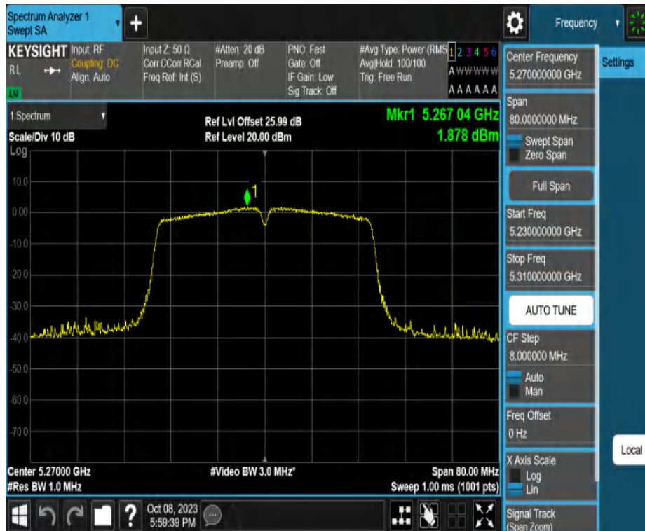
11N40MIMO_Ant2_5270
