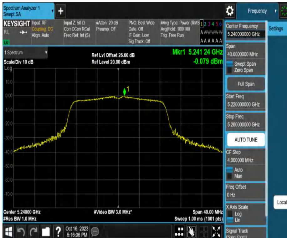
11AC20MIMO_Ant2_5240
