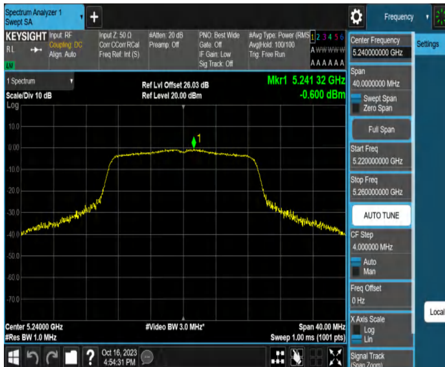
11N20MIMO_Ant2_5240
