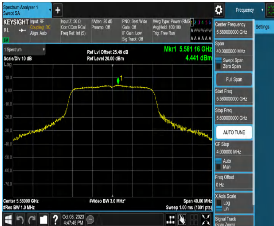
11A-CDD_Ant2_5580
