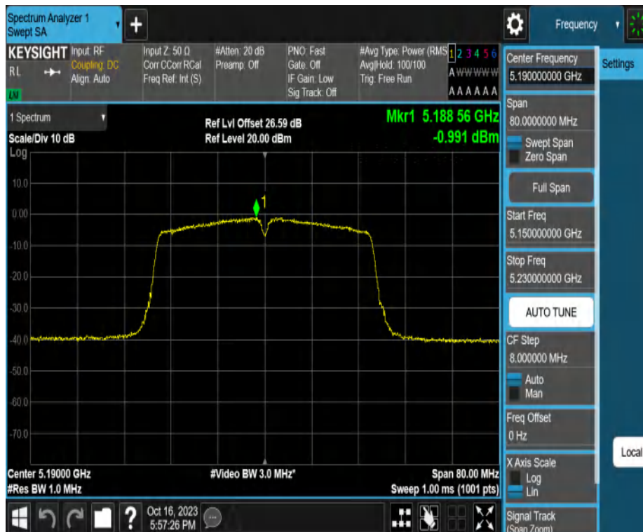
11N40MIMO_Ant2_5190
