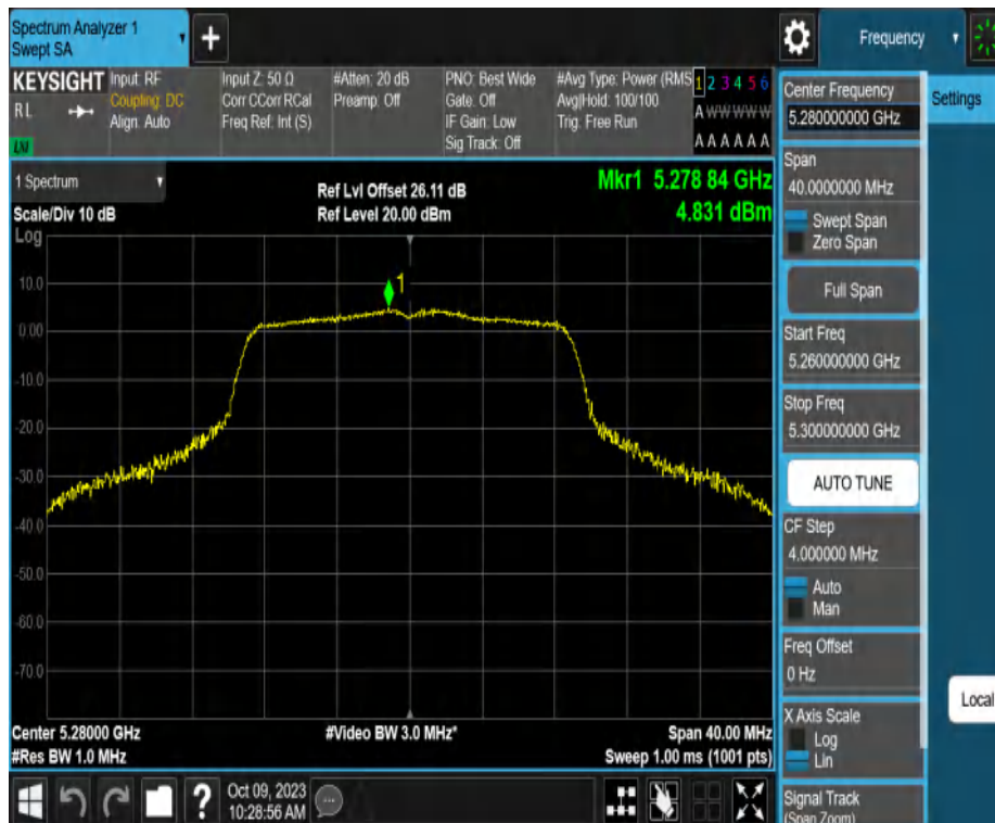
11AC20MIMO_Ant2_5280
