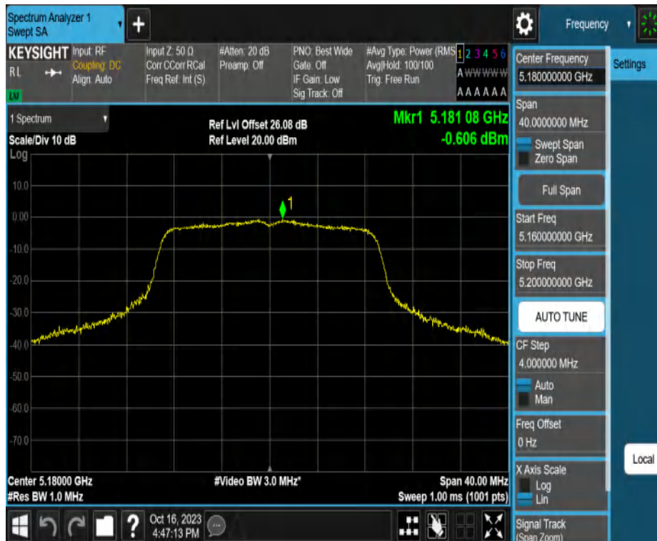
11N20MIMO_Ant2_5180
