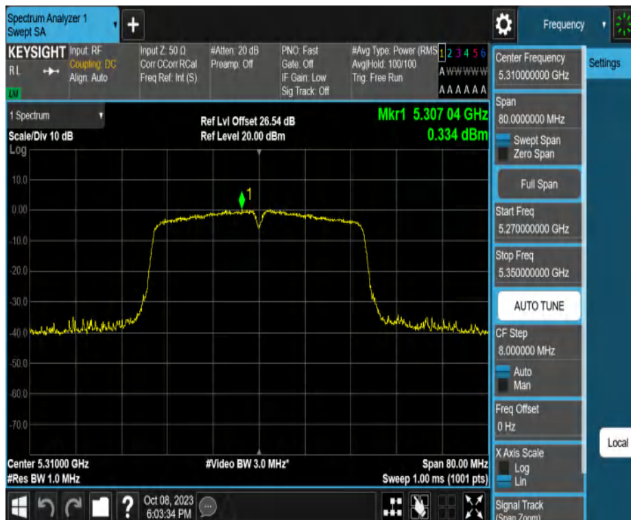
11N40MIMO_Ant2_5310
