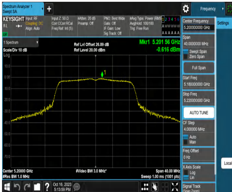
11AC20MIMO_Ant2_5200
