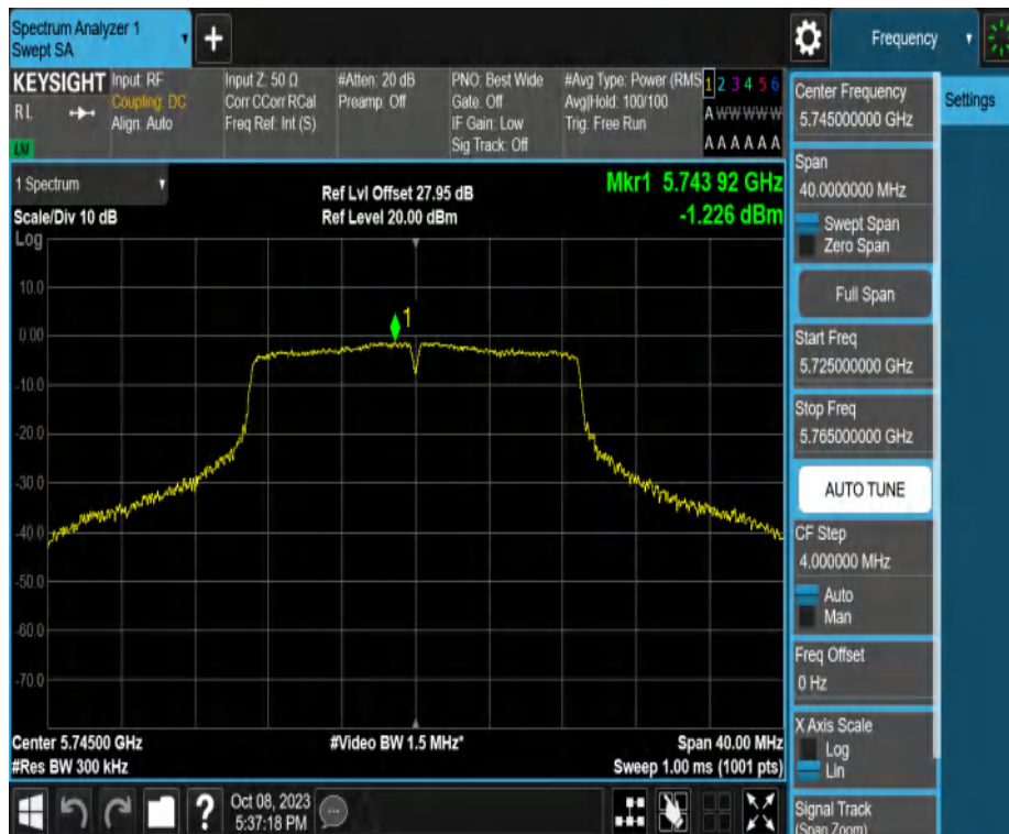
11N20MIMO_Ant2_5745
