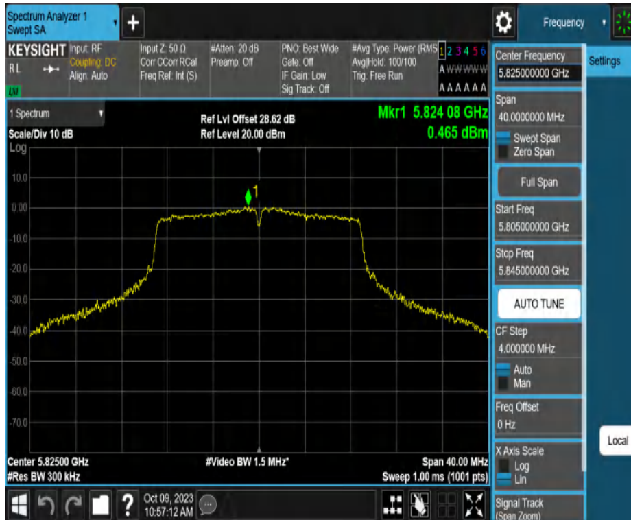
11AC20MIMO_Ant2_5825
