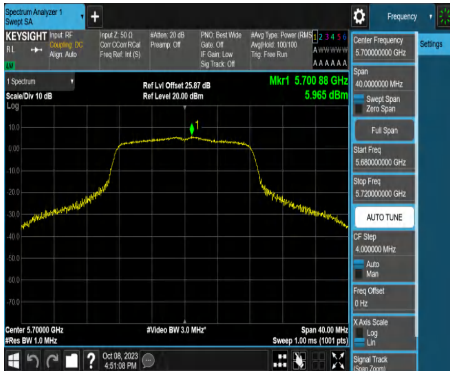
11A-CDD_Ant2_5700
