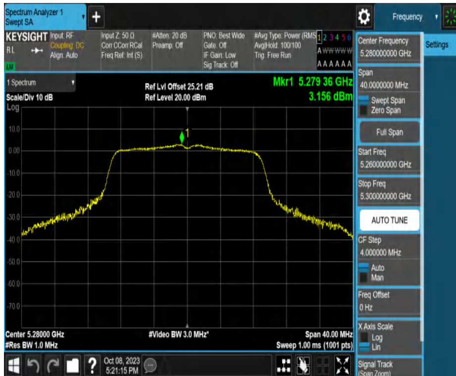
11N20MIMO_Ant2_5280
