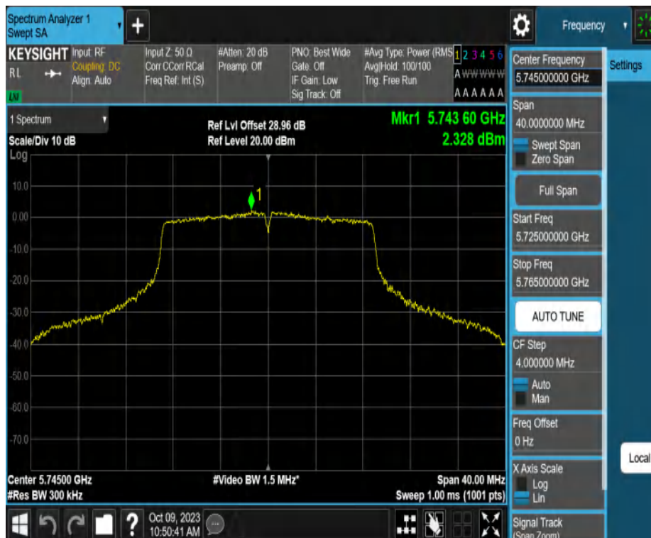
11AC20MIMO_Ant2_5745
