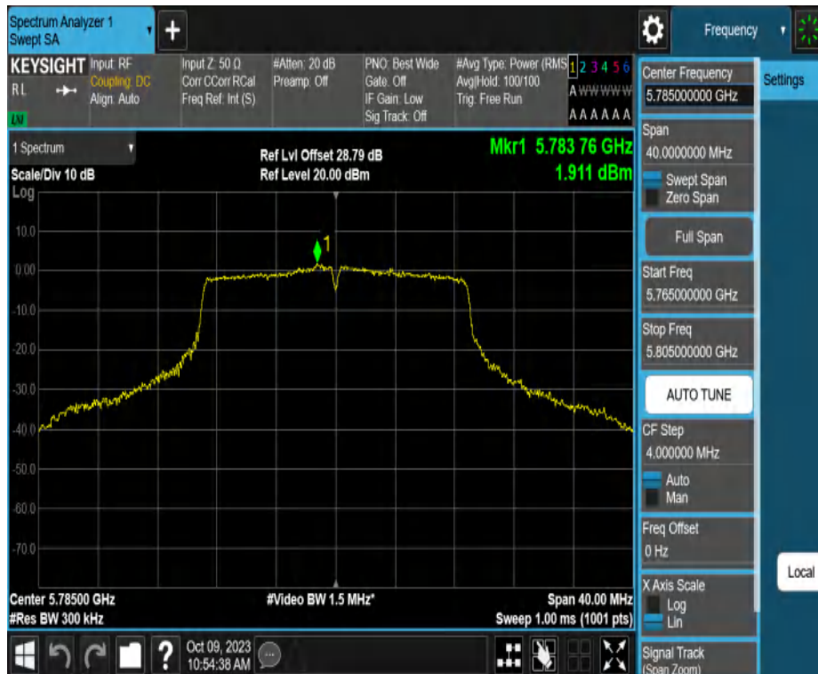
11AC20MIMO_Ant2_5785
