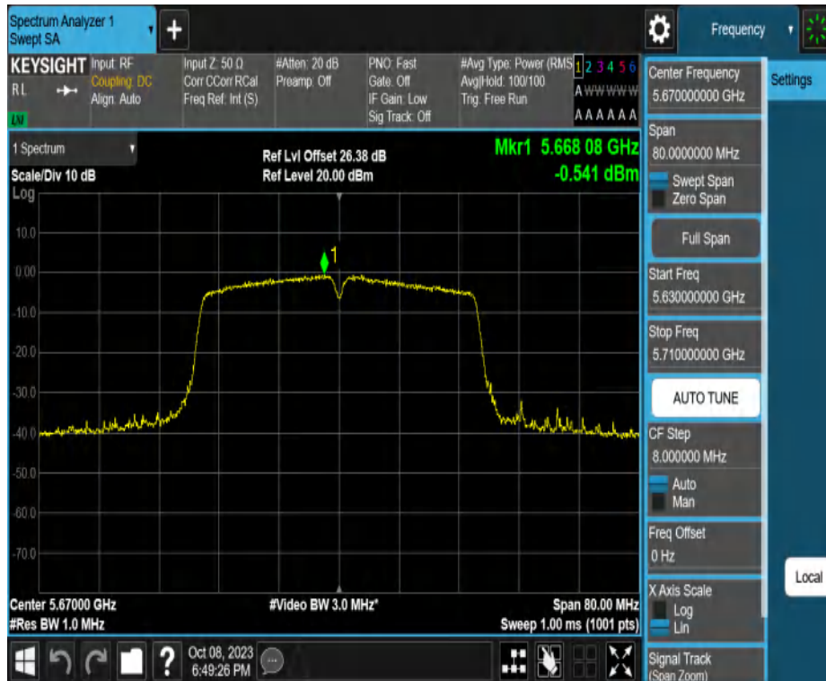
11N40MIMO_Ant2_5670
