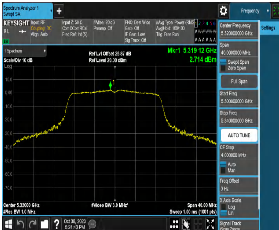
11N20MIMO_Ant2_5320
