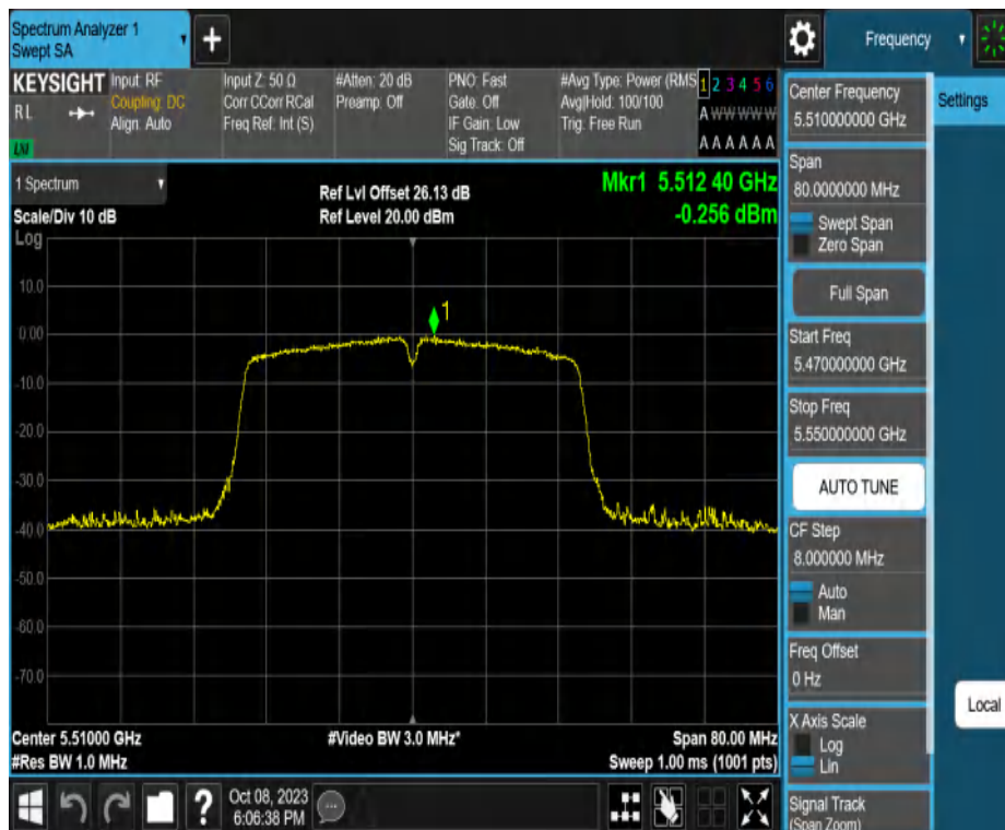
11N40MIMO_Ant2_5510
