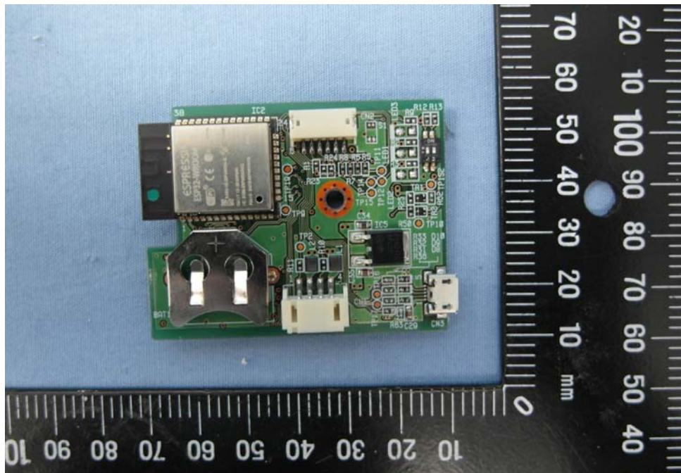
EUT Photo (36)
