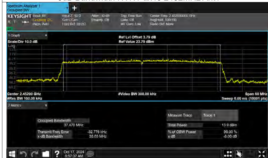
-6dB Bandwidth NVNT ax40 2452MHz Ant1
