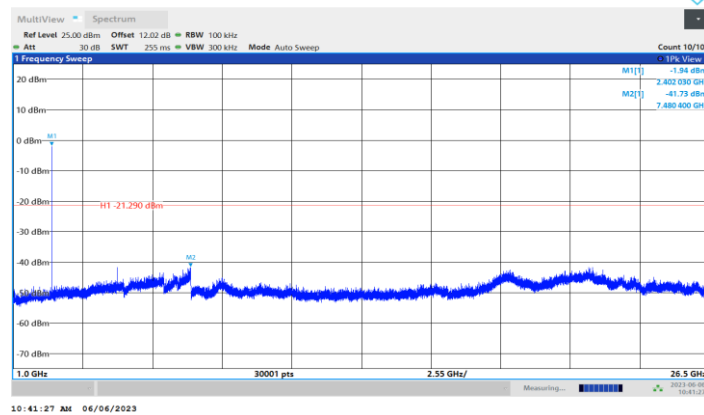
BLE_2M_Ant1_2402_1000~26500
