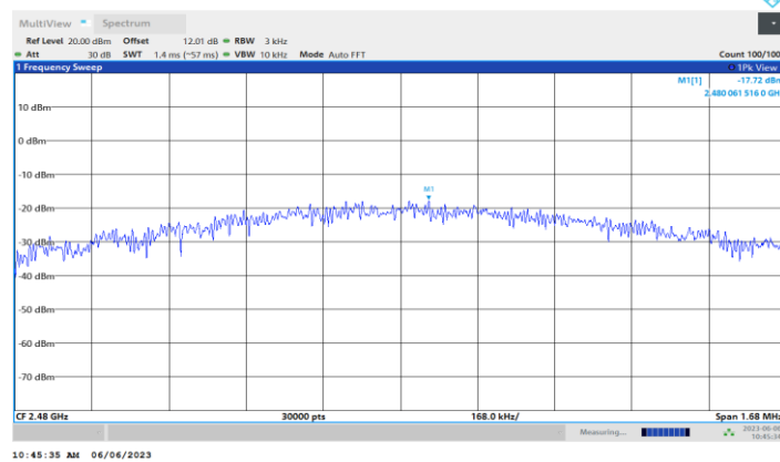
BLE_2M_Ant1_2480
