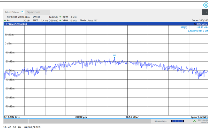
BLE_2M_Ant1_2402
