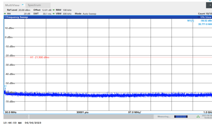
BLE_2M_Ant1_2480_30~1000
