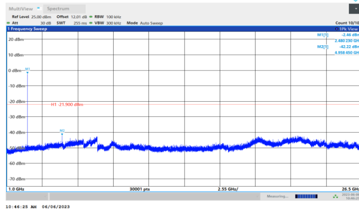
BLE_2M_Ant1_2480_1000~26500
