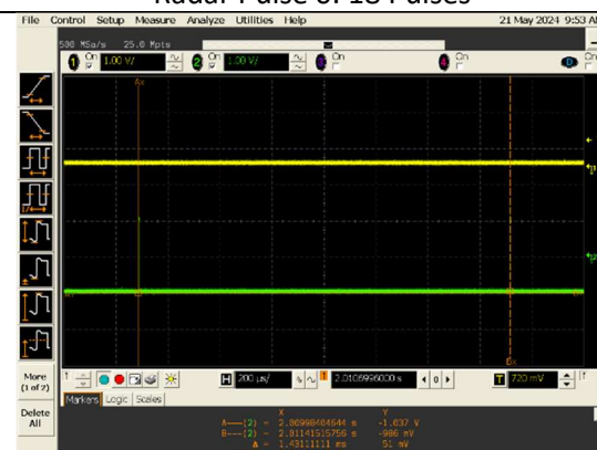
Radar Pulse 0: PRI 1.428 msec
