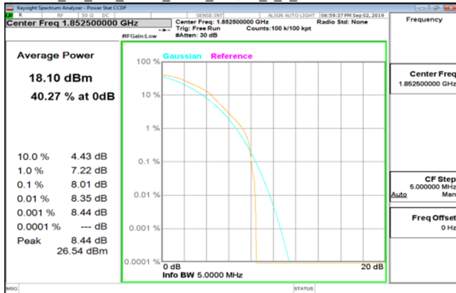
Cat M1 LTE_Band2_5MHz_16QAM_6_0_LowCH18625-1852.5
