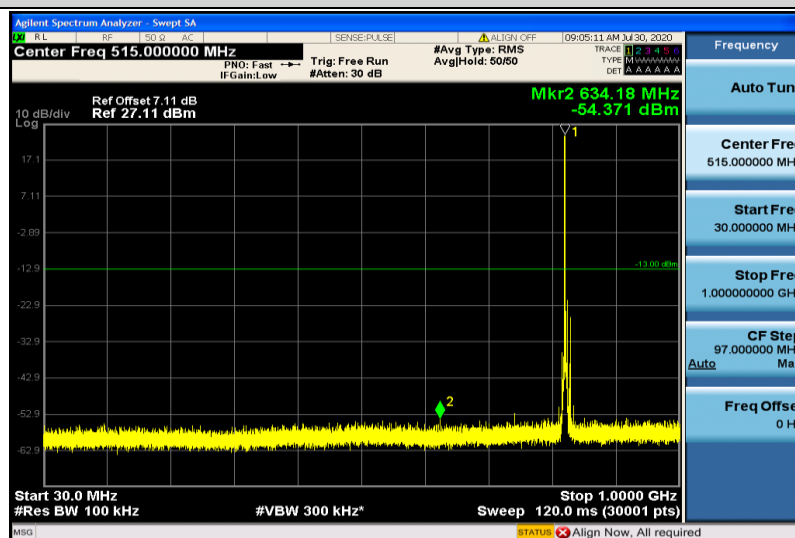
Band5-5MHz-QPSK-20425-1RB#0-30~1000MHz
