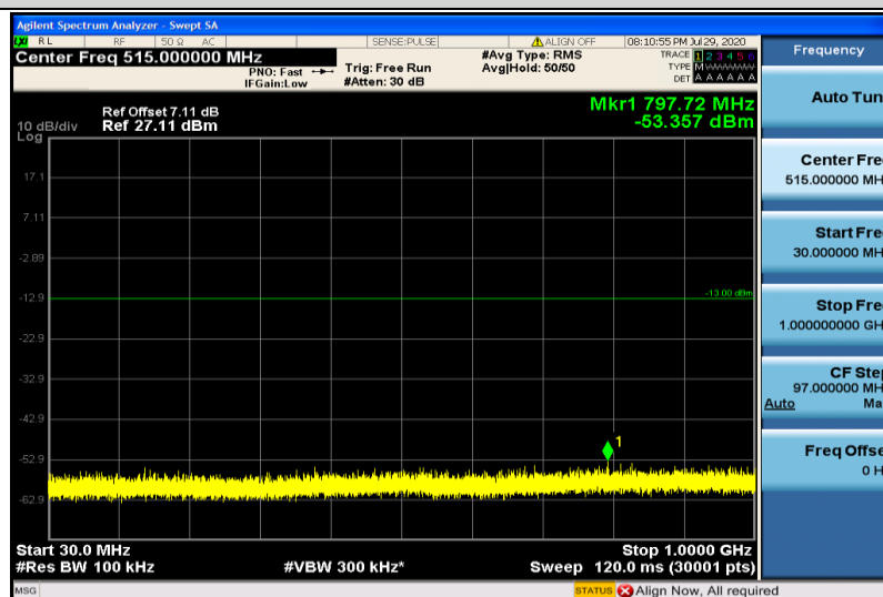
Band4-10MHz-QPSK-20000-1RB#0-30~1000MHz
