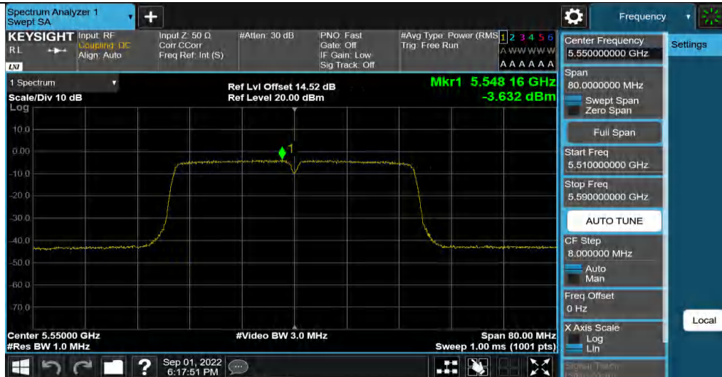
11N40MIMO Ant2 5550
