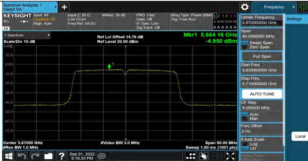
11N40MIMO Ant4 5670
