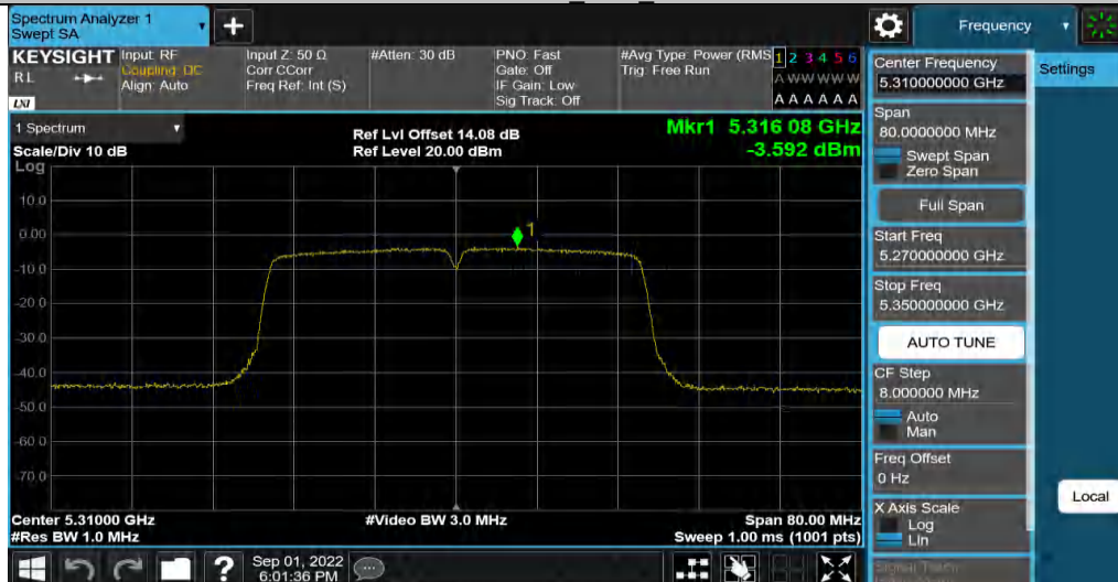
11N40MIMO Ant2 5310
