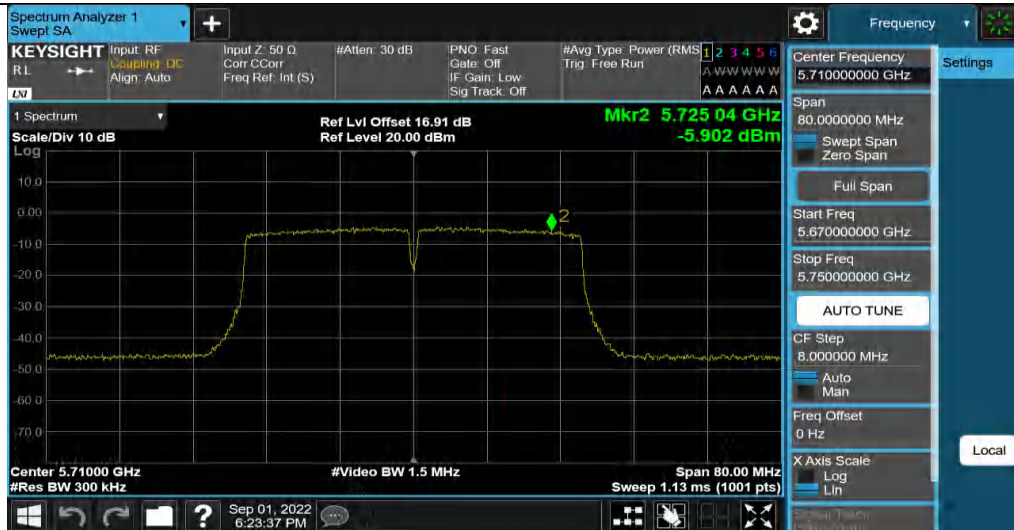
11N40MIMO_Ant2_5710_UNII-3
