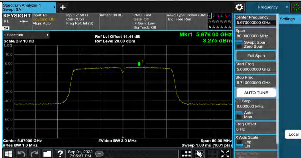
11AC40MIMO_Ant2_5670
