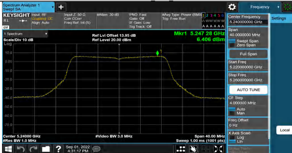
11AC20MIMO_Ant2_5240
