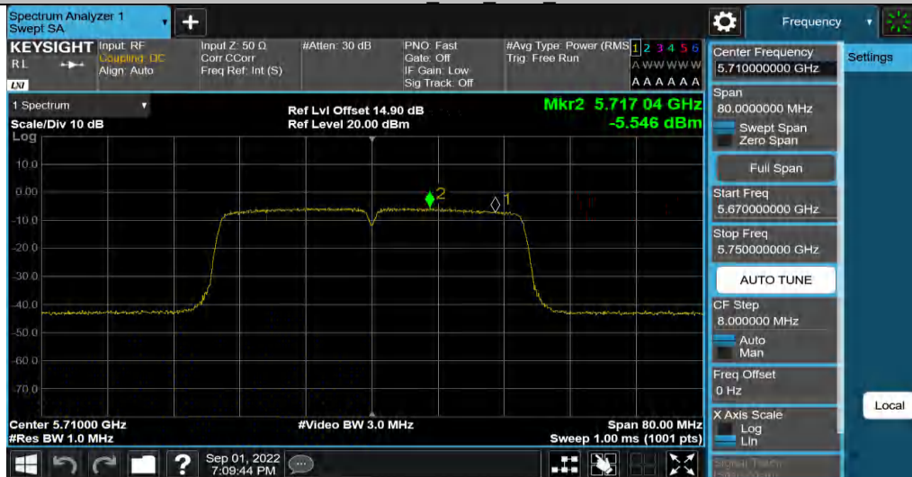
11AC40MIMO_Ant4_5710_UNII-2C
