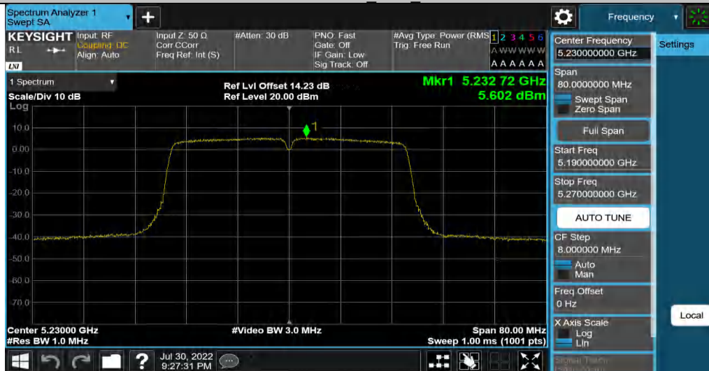
11AC40MIMO_Ant4_5230
