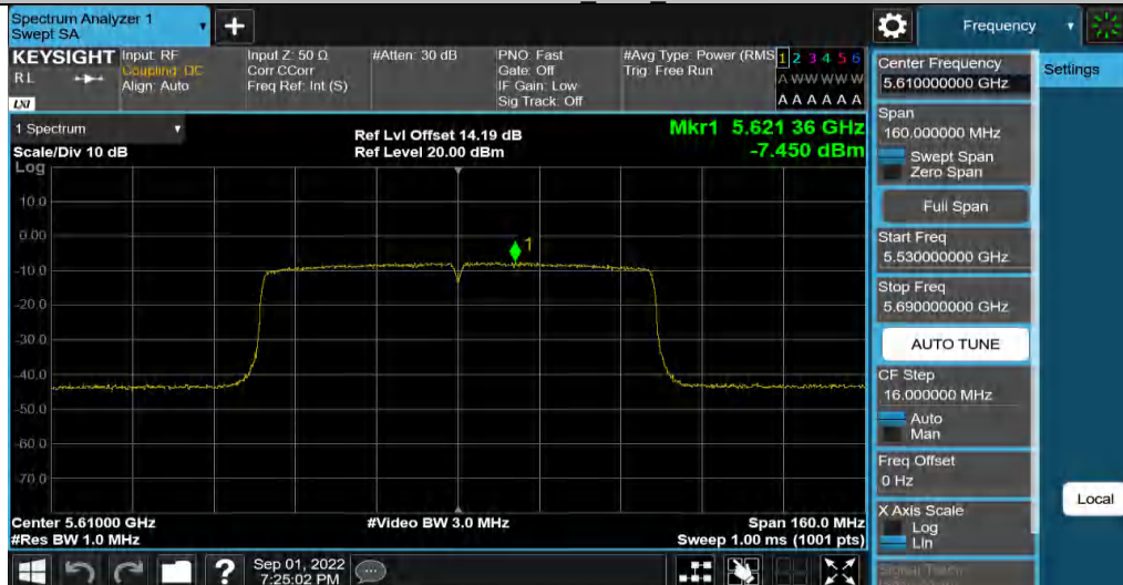
11AC80MIMO_Ant2_5610
