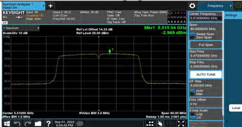
11N40MIMO Ant2 5510
