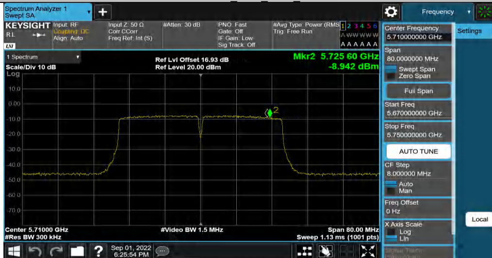
11N40MIMO_Ant4_5710_UNII-3
