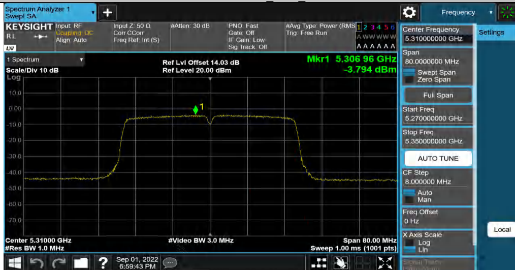
11AC40MIMO_Ant2_5310
