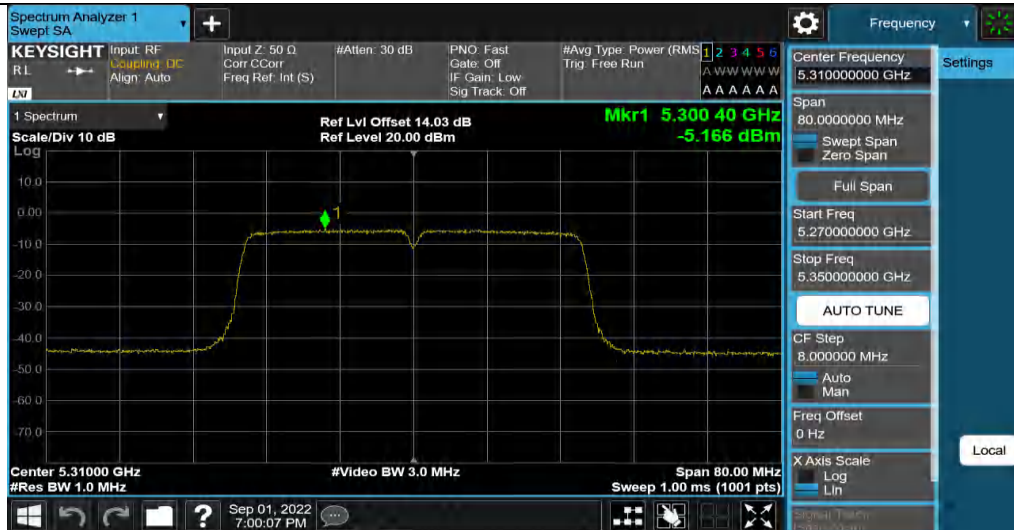
11AC40MIMO_Ant3_5310
