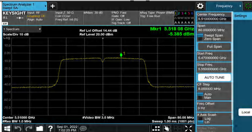
11AC40MIMO_Ant4_5510
