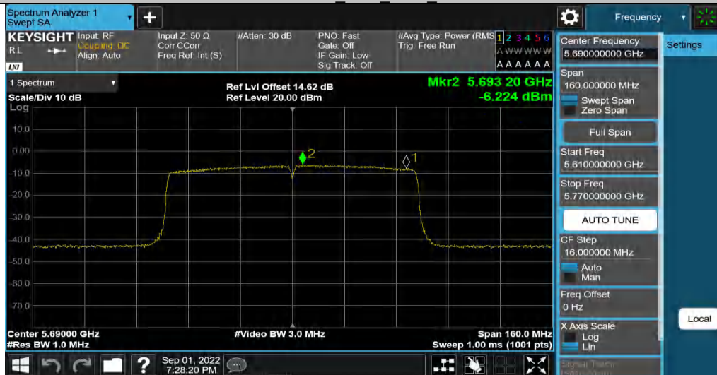
11AC80MIMO_Ant2_5690_UNII-2C
