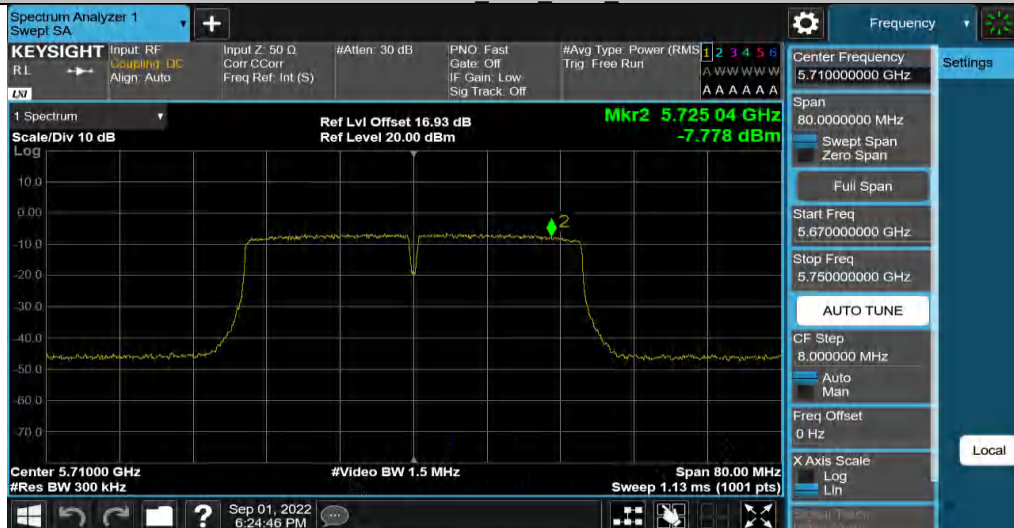
11N40MIMO_Ant3_5710_UNII-3
