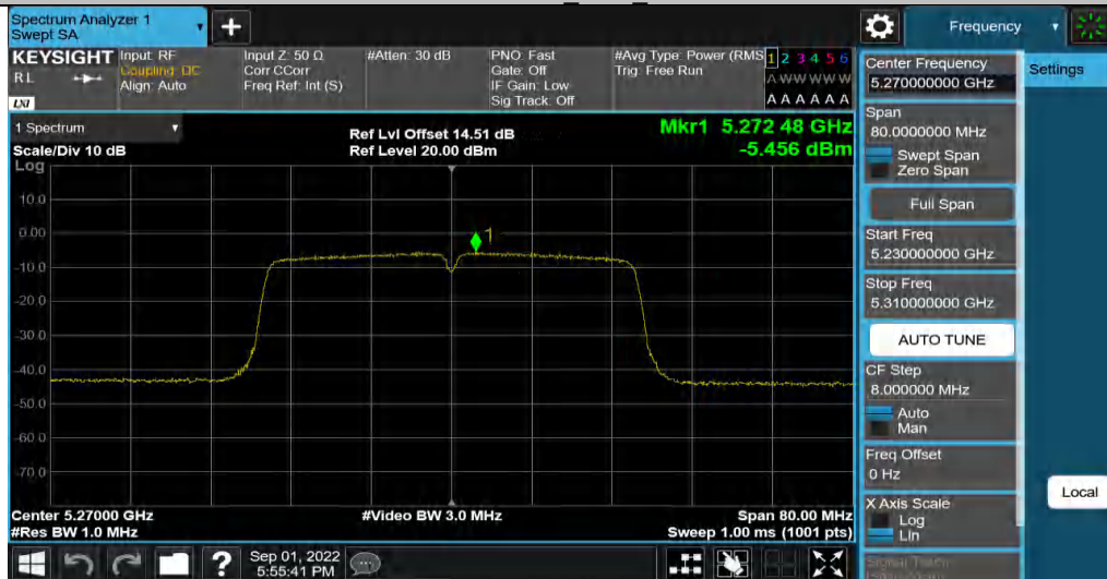
11N40MIMO Ant4 5270
