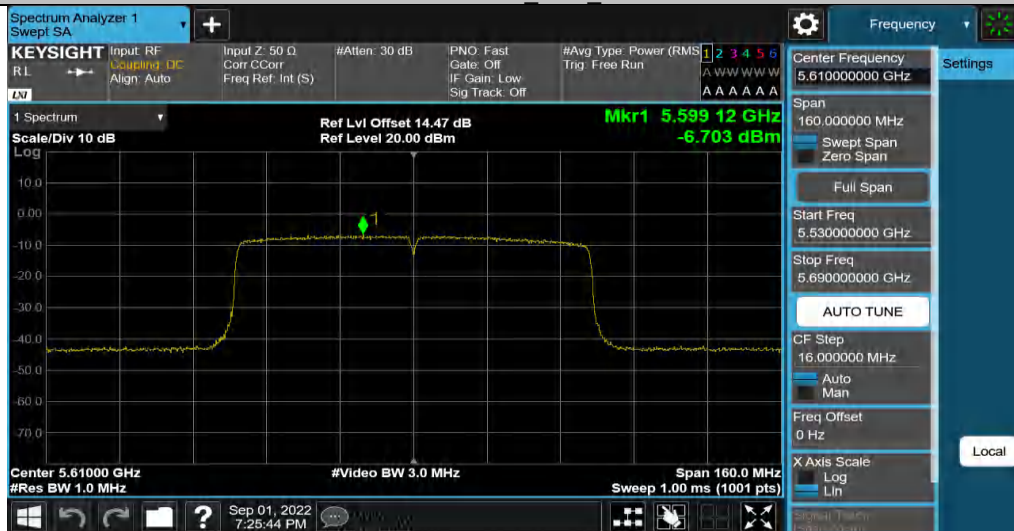
11AC80MIMO_Ant3_5610
