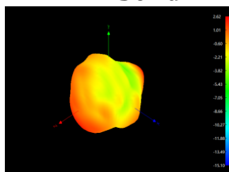
2450 -dBi
