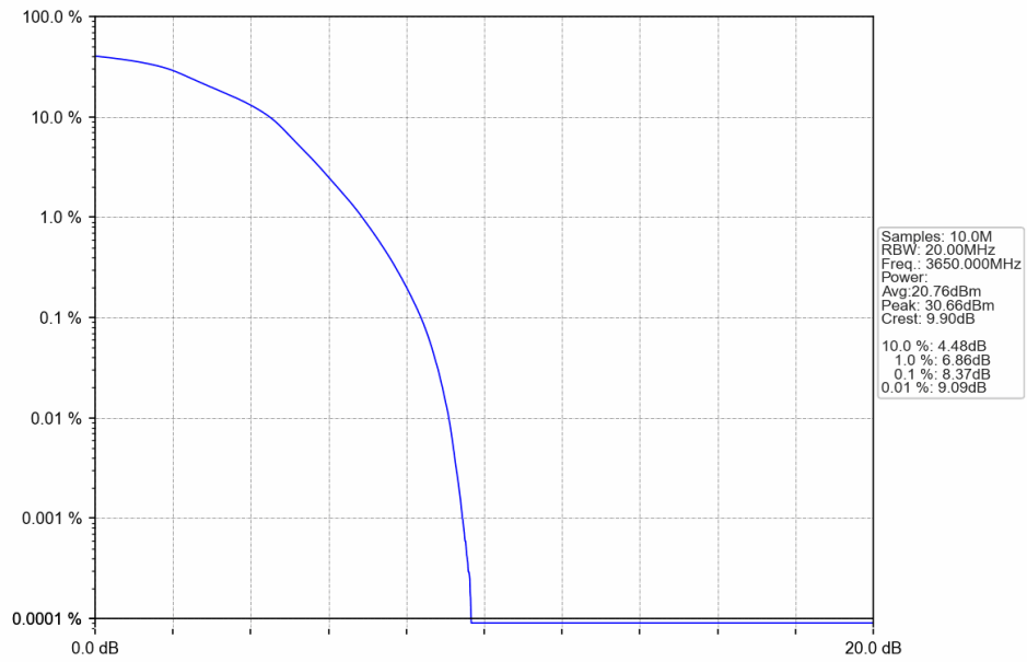
Band43c 20MHz 16QAM MCH 3650MHz RB 100 0 NTNV
