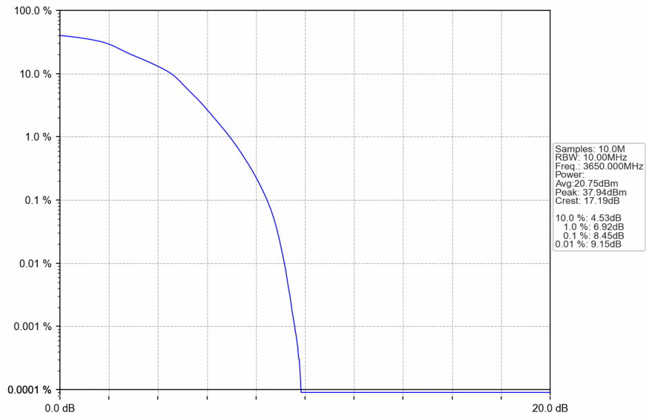
Band43c 10MHz 16QAM MCH 3650MHz RB 50 0 NTNV
