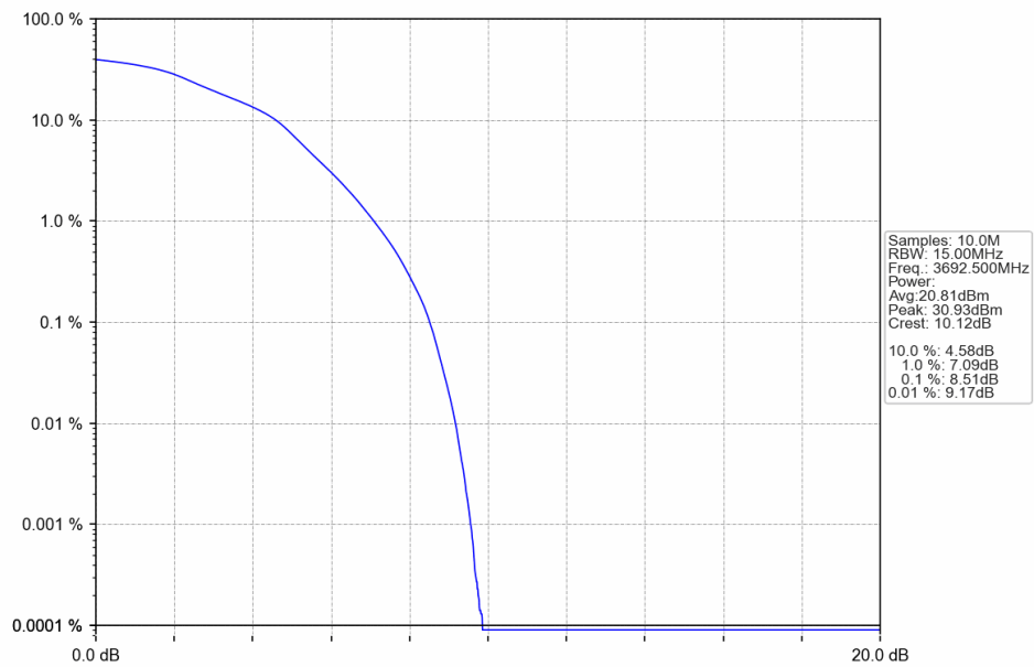
Band43c 15MHz 16QAM HCH 3692.5MHz RB 75 0 NTNV
