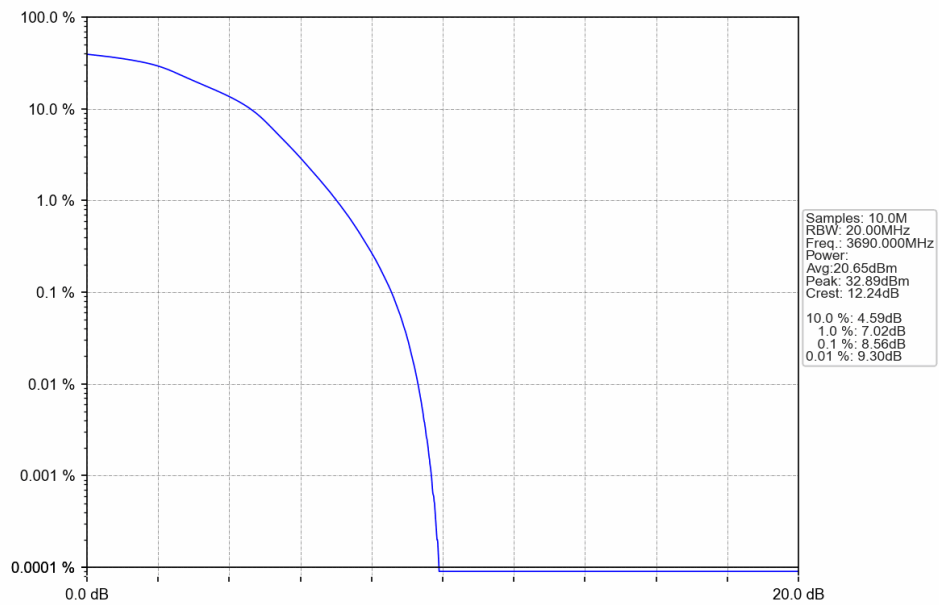
Band43c 20MHz 16QAM HCH 3690MHz RB 100 0 NTNV
