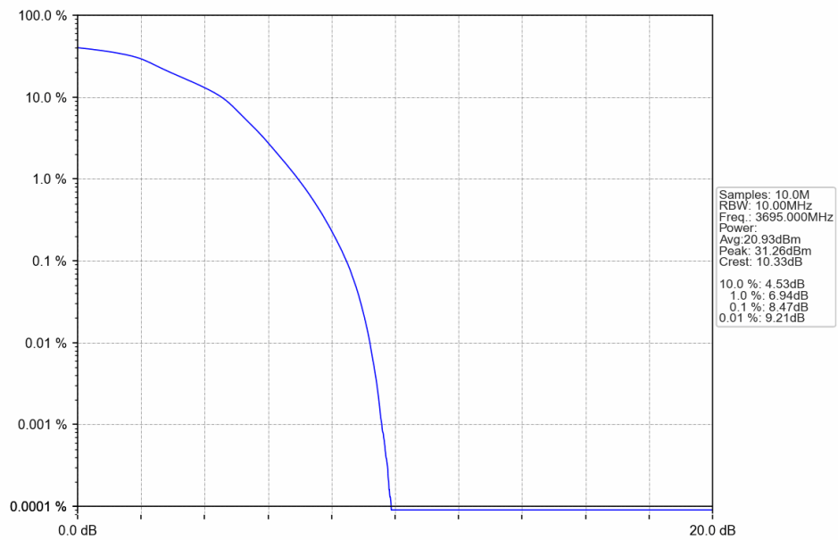
Band43c 10MHz 16QAM HCH 3695MHz RB 50 0 NTNV
