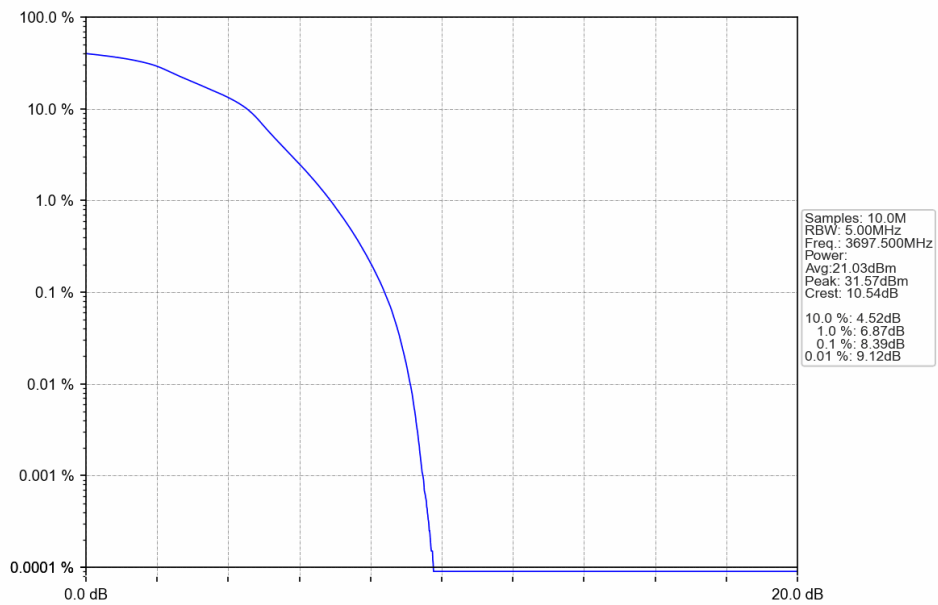
Band43c 5MHz 16QAM HCH 3697.5MHz RB 25 0 NTNV
