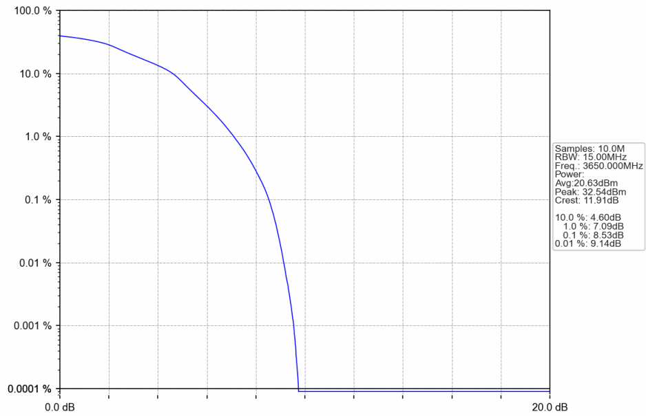
Band43c 15MHz 16QAM MCH 3650MHz RB 75 0 NTNV
