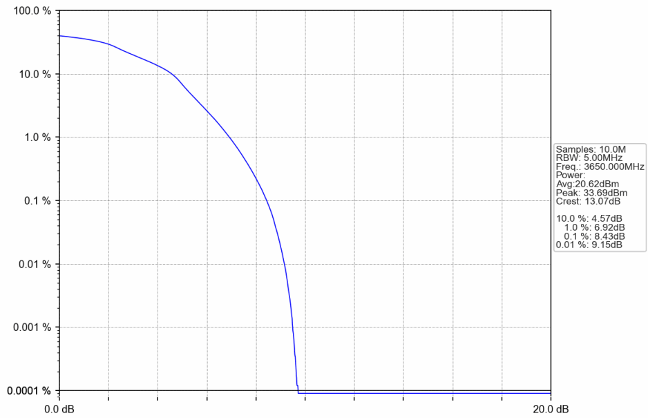
Band43c 5MHz 16QAM MCH 3650.00MHz RB 25 0 NTNV
