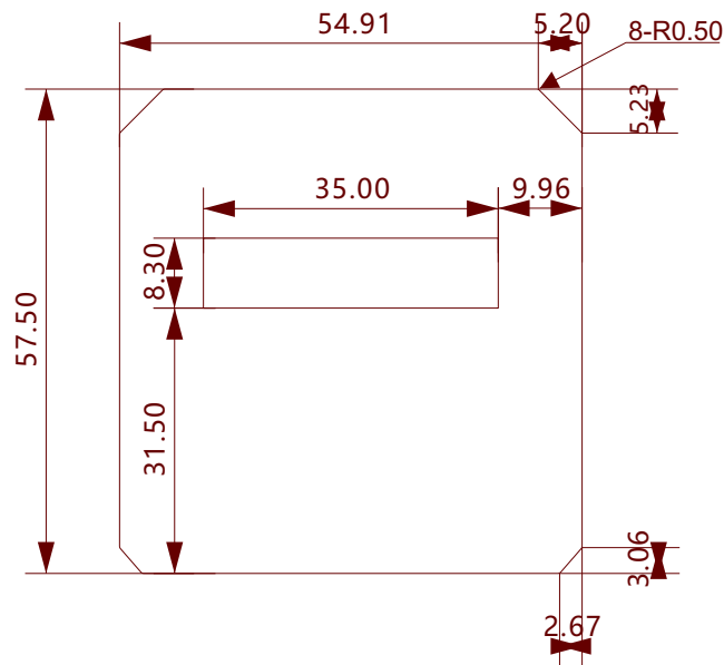
(尺寸图)
