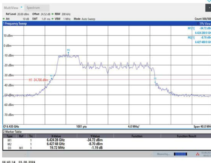
11AX20MIMO_Ant2_6435_106Tone_RU53
