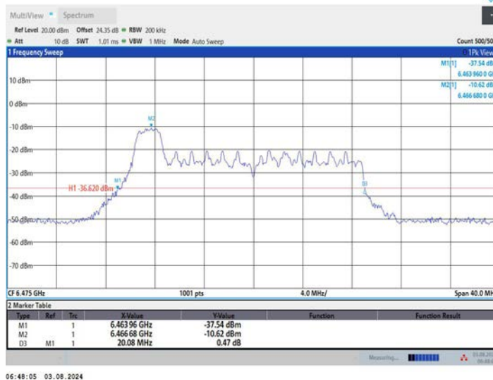
11AX20MIMO_Ant1_6475_52Tone_RU37
