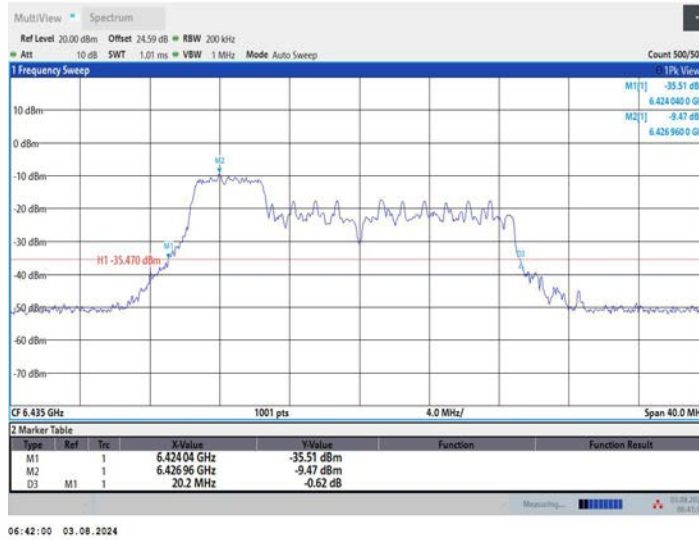
11AX20MIMO_Ant1_6435_106Tone_RU53
