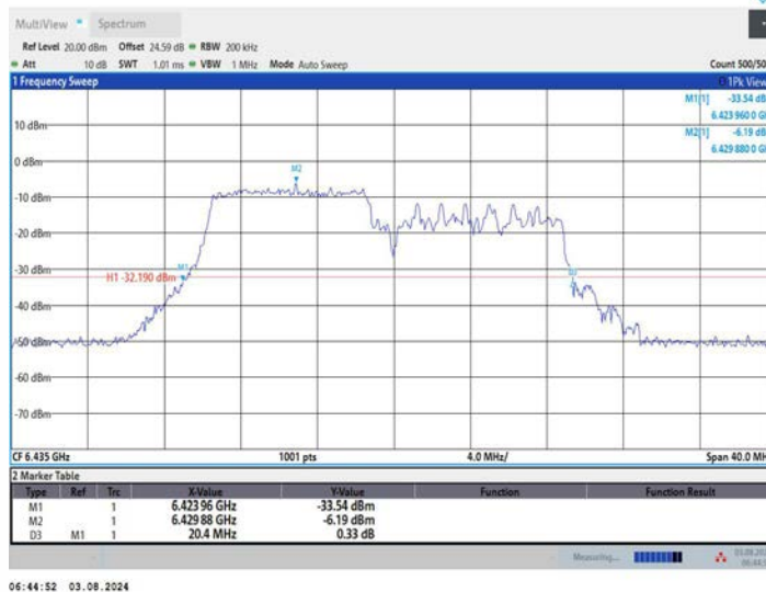
11AX20MIMO_Ant2_6435_26Tone_RU0
