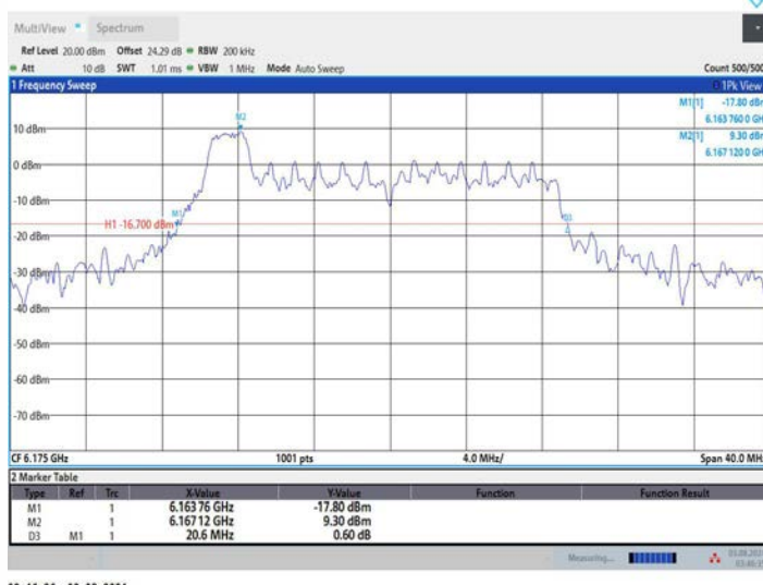
11AX20MIMO_Ant1_6175_52Tone_RU37
