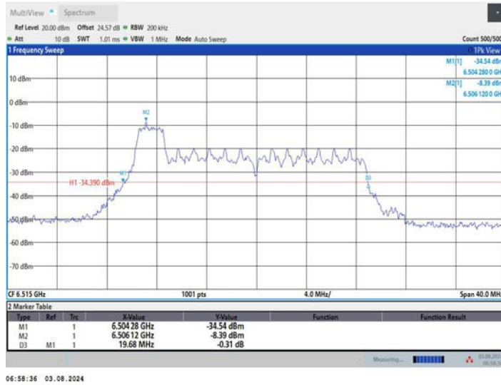
11AX20MIMO_Ant2_6515_52Tone_RU37
