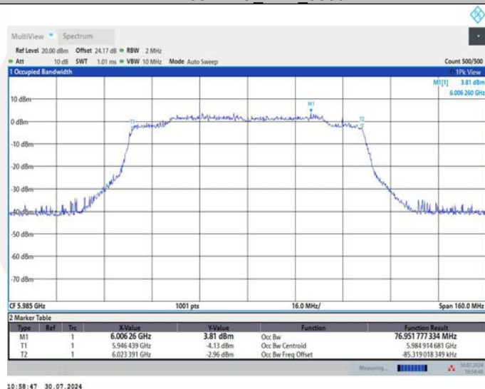
11AX80MIMO_Ant2_5985
