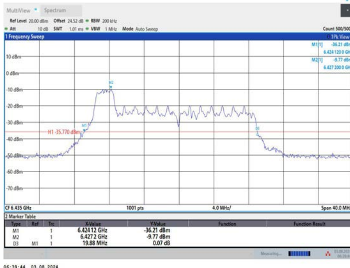
11AX20MIMO_Ant2_6435_52Tone_RU37
