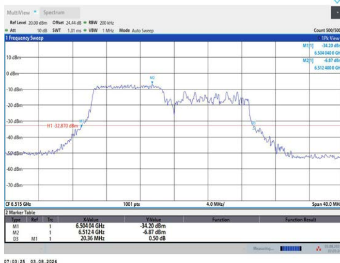
11AX20MIMO_Ant2_6515_26Tone_RU0
