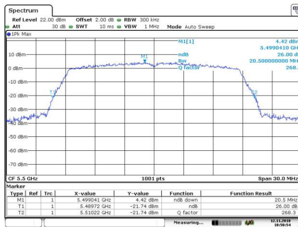
26dB_802.11n_HT20_5500MHz
