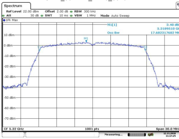
OBW_802.11n_HT20_5320MHz
