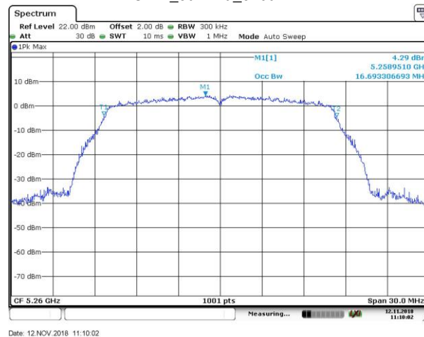
OBW_802.11a_5260MHz
