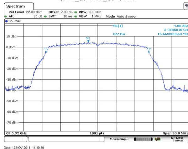
OBW_802.11a_5320MHz
