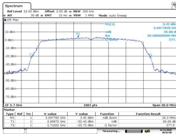
26dB_802.11n_HT20_5700MHz
