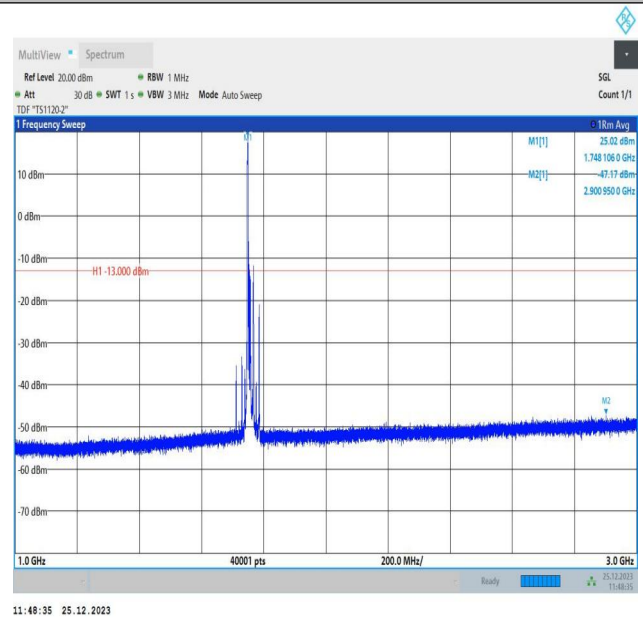
66-66-10MHz-5MHz-QPSK-QPSK-132397-132469-1RB#0-0R B#0-1000~3000MHz-PASS
