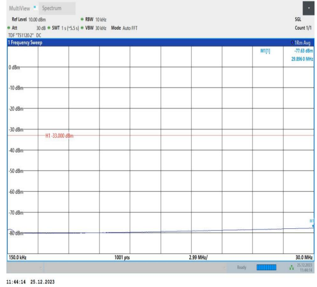
66-66-10MHz-5MHz-QPSK-QPSK-132022-132094-1RB#0-1R B#24-0.15~30MHz-PASS
