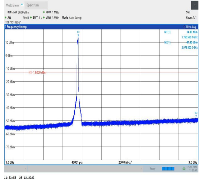
66-66-10MHz-5MHz-QPSK-QPSK-132397-132469-50RB#0-25RB#0-1000~3000MHz-PASS
