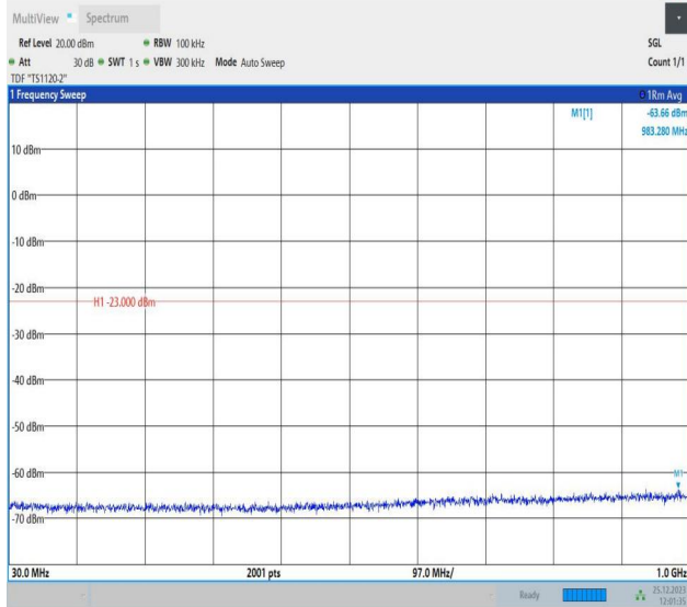
66-66-10MHz-5MHz-QPSK-QPSK-132572-132644-50RB#0-25RB#0-30~1000MHz-PASS
