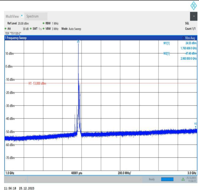
66-66-10MHz-5MHz-QPSK-QPSK-132572-132644-1RB#0-0R B#0-1000~3000MHz-PASS
