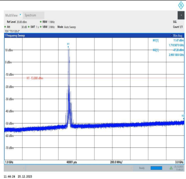
66-66-10MHz-5MHz-QPSK-QPSK-132022-132094-1RB#0-1R B#24-1000~3000MHz-PASS
