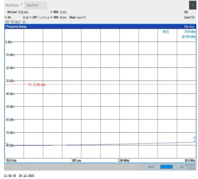
66-66-10MHz-5MHz-QPSK-QPSK-132397-132469-1RB#0-1R B#24-0.15~30MHz-PASS
