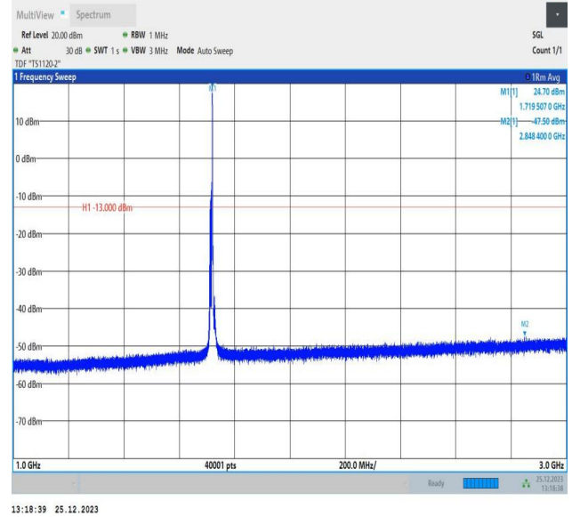
66-66-10MHz-10MHz-QPSK-QPSK-132022-132121-1RB#49- ORB#0-1000~3000MHz-PASS
