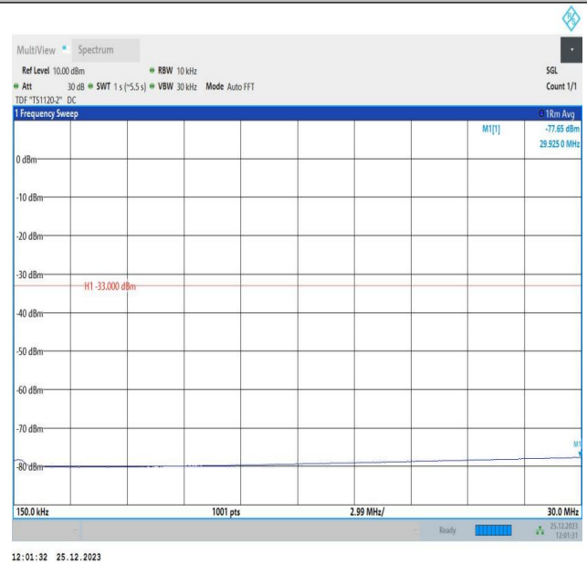
66-66-10MHz-5MHz-QPSK-QPSK-132572-132644-50RB#0-25RB#0-0.15~30MHz-PASS
