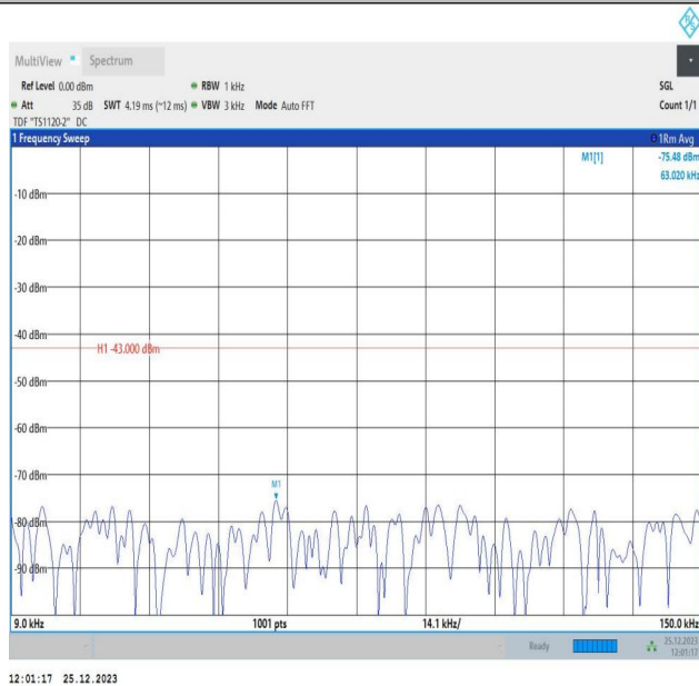
66-66-10MHz-5MHz-QPSK-QPSK-132572-132644-50RB#0-25RB#0-0.009~0.15MHz-PASS
