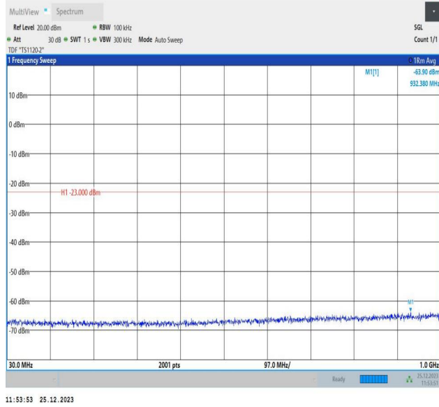
66-66-10MHz-5MHz-QPSK-QPSK-132397-132469-50RB#0-25RB#0-30~1000MHz-PASS
