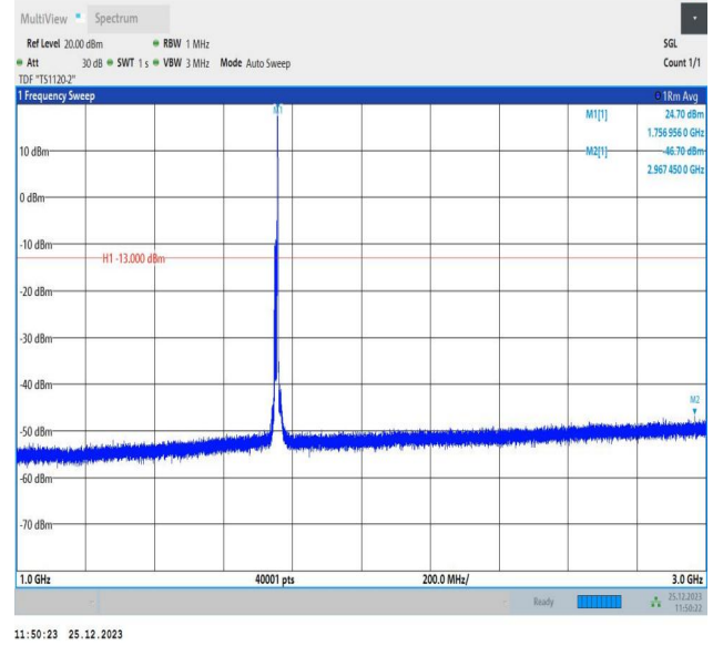
66-66-10MHz-5MHz-QPSK-QPSK-132397-132469-1RB#49-0 RB#0-1000~3000MHz-PASS
