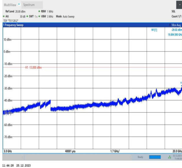
66-66-10MHz-5MHz-QPSK-QPSK-132022-132094-1RB#0-1 RB#24-3000~20000MHz-PASS
