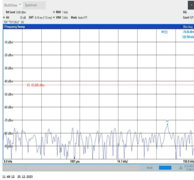
66-66-10MHz-5MHz-QPSK-QPSK-132397-132469-1RB#0-0 RB#0-0.009~0.15MHz-PASS
