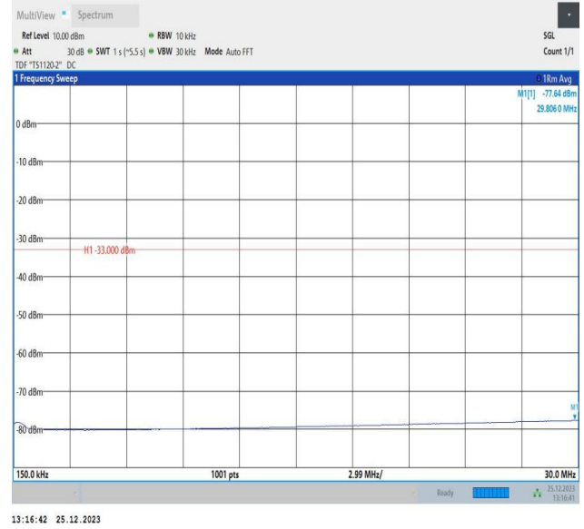
66-66-10MHz-10MHz-QPSK-QPSK-132022-132121-1RB#0-0RB#0-0.15~30MHz-PASS
