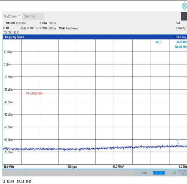
66-66-10MHz-5MHz-QPSK-QPSK-132397-132469-1RB#0-1 RB#24-30~1000MHz-PASS
