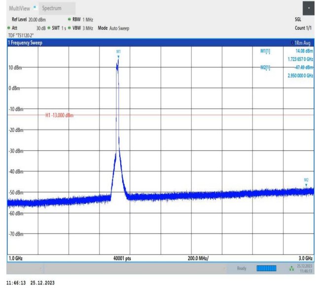
66-66-10MHz-5MHz-QPSK-QPSK-132022-132094-50RB#0-25RB#0-1000~3000MHz-PASS
