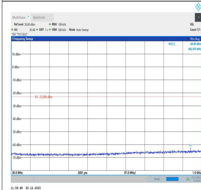
66-66-10MHz-5MHz-QPSK-QPSK-132572-132644-1RB#0-1 RB#24-30~1000MHz-PASS
