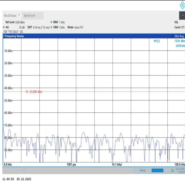
66-66-10MHz-5MHz-QPSK-QPSK-132397-132469-1RB#49-0RB#0-0.009~0.15MHz-PASS
