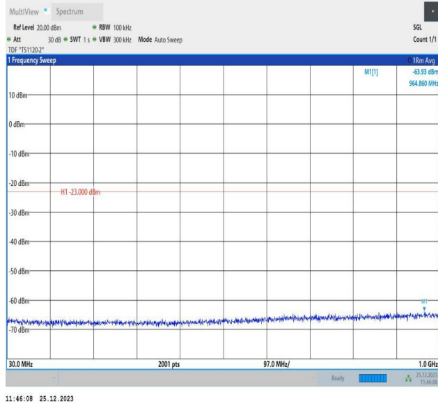
66-66-10MHz-5MHz-QPSK-QPSK-132022-132094-50RB#0-25RB#0-30~1000MHz-PASS
