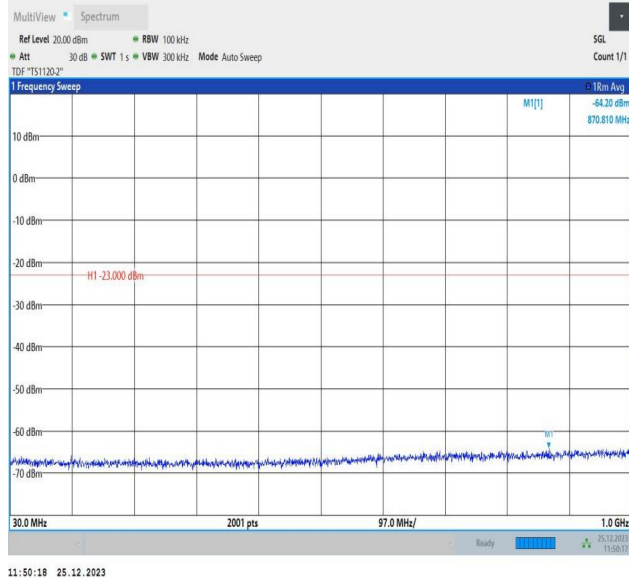
66-66-10MHz-5MHz-QPSK-QPSK-132397-132469-1RB#49- ORB#0-30~1000MHz-PASS
