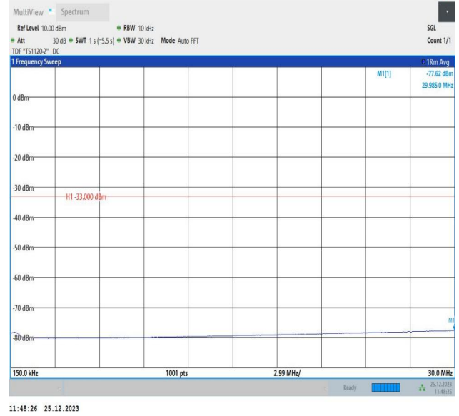
66-66-10MHz-5MHz-QPSK-QPSK-132397-132469-1RB#0-0R B#0-0.15~30MHz-PASS
