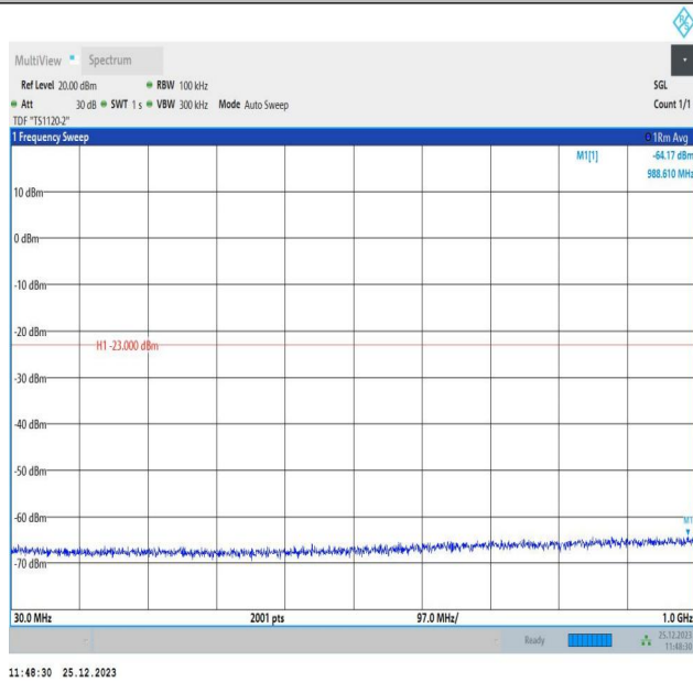
66-66-10MHz-5MHz-QPSK-QPSK-132397-132469-1RB#0-0 RB#0-30~1000MHz-PASS
