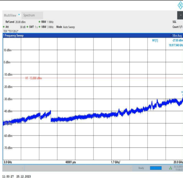
66-66-10MHz-5MHz-QPSK-QPSK-132397-132469-1RB#49- ORB#0-3000~20000MHz-PASS
