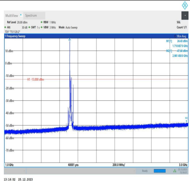
66-66-10MHz-10MHz-QPSK-QPSK-132022-132121-1RB#0-0RB#0-1000~3000MHz-PASS
