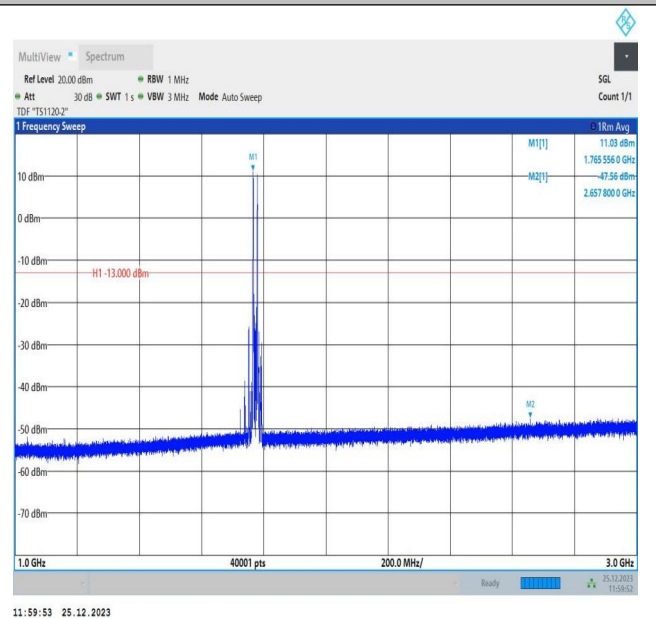
66-66-10MHz-5MHz-QPSK-QPSK-132572-132644-1RB#0-1R B#24-1000~3000MHz-PASS
