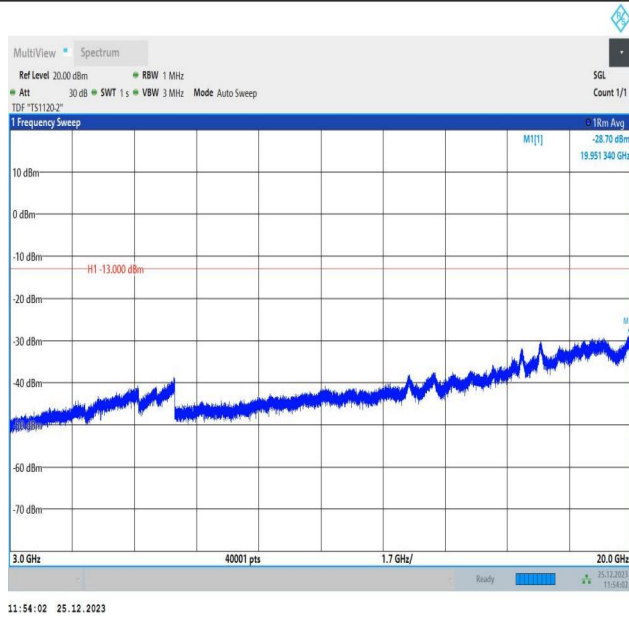
66-66-10MHz-5MHz-QPSK-QPSK-132397-132469-50RB#0-25RB#0-3000~20000MHz-PASS
