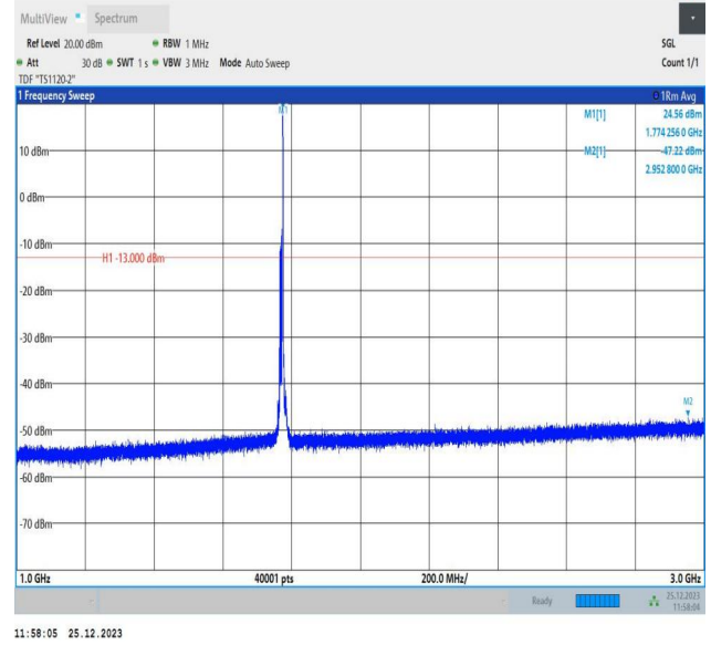
66-66-10MHz-5MHz-QPSK-QPSK-132572-132644-1RB#49-0 RB#0-1000~3000MHz-PASS
