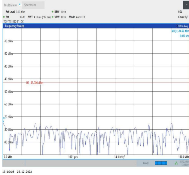
66-66-10MHz-10MHz-QPSK-QPSK-132022-132121-1RB#0-0RB#0-0.009~0.15MHz-PASS
