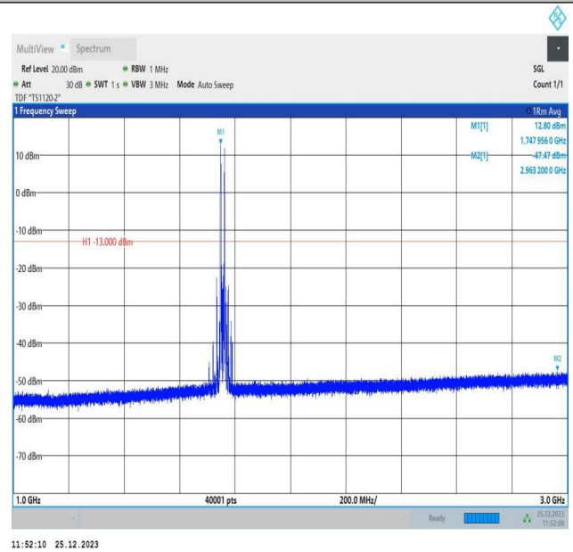
66-66-10MHz-5MHz-QPSK-QPSK-132397-132469-1RB#0-1R B#24-1000~3000MHz-PASS
