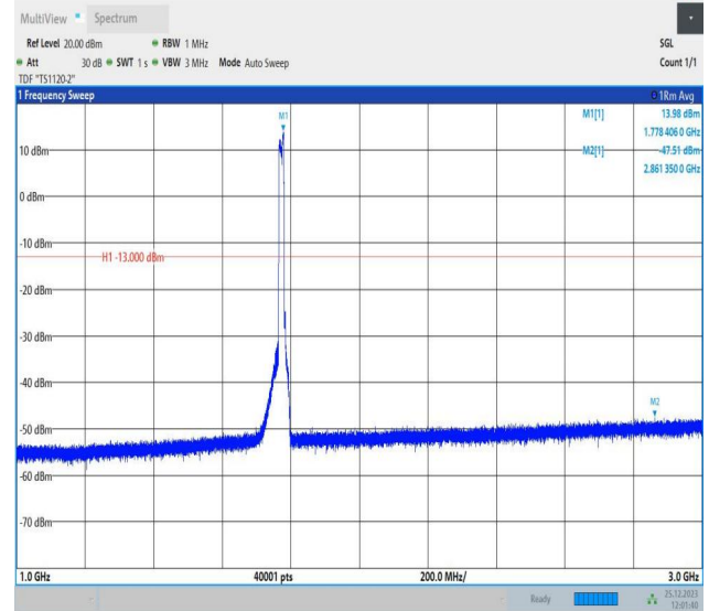
66-66-10MHz-5MHz-QPSK-QPSK-132572-132644-50RB#0-25RB#0-1000~3000MHz-PASS
