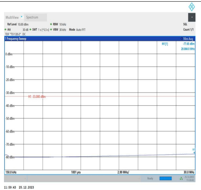
66-66-10MHz-5MHz-QPSK-QPSK-132572-132644-1RB#0-1R B#24-0.15~30MHz-PASS
