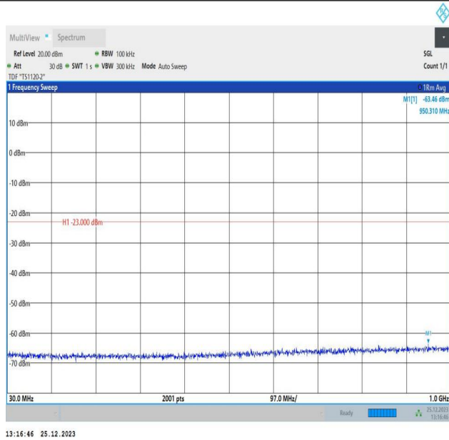
66-66-10MHz-10MHz-QPSK-QPSK-132022-132121-1RB#0-0RB#0-30~1000MHz-PASS
