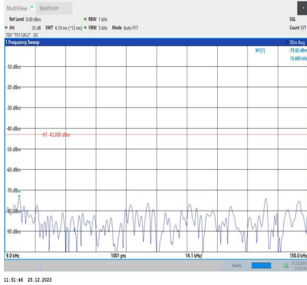
66-66-10MHz-5MHz-QPSK-QPSK-132397-132469-1RB#0-1 RB#24-0.009~0.15MHz-PASS
